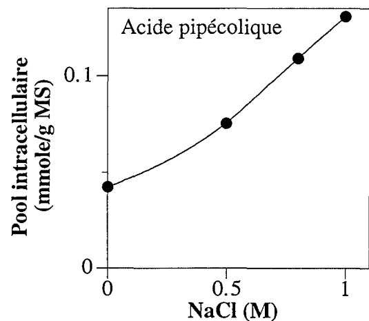
Figure n°I.19 : Teneur intracellulaire en acide pipécolique chez B. ammoniagenes cultivée à différentes concentrations en NaCl. (D'après Gouesbet et al., 1992).
