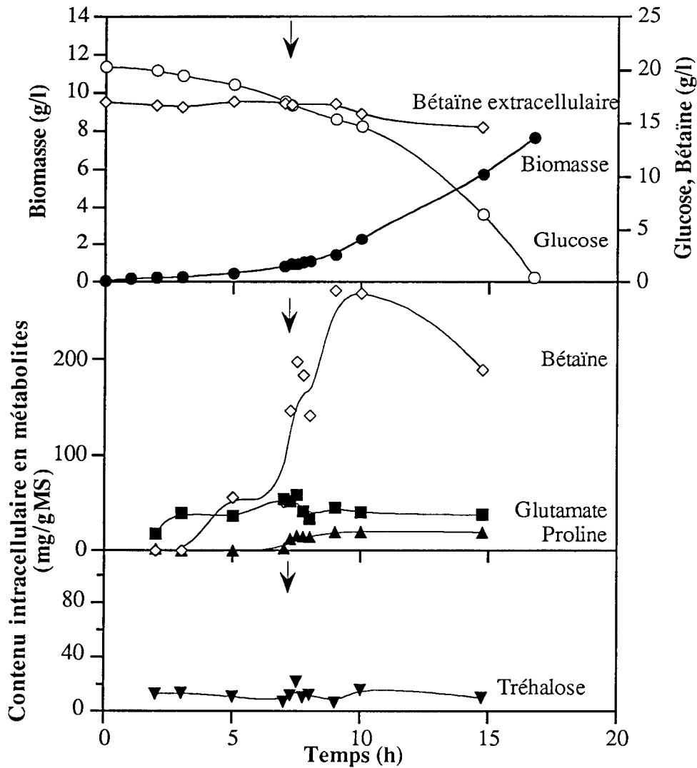
Figure n°III.11 : Cinétiques de croissance, de consommation de glucose et de bétaïne et d'accumulation de métabolites chez C. glutamicum ATCC 14752 cultivée en présence de 14 g/l de bétaïne : Biomasse (●), Glucose (○), Bétaïne (◇), Proline (▲), Acide glutamique (■) et Tréhalose (▼). La flèche indique le moment où le NaCl a été ajouté pour augmenter l'osmolalité du milieu de 0,4 à 1,5 osmol.kg -1 .
