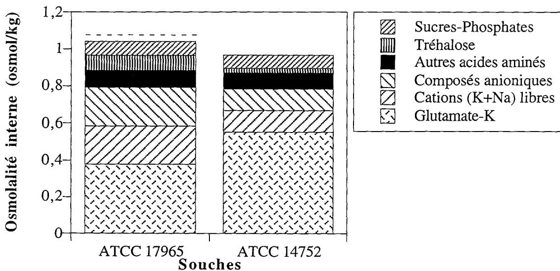
Figure n°VI.7 : Bilan osmotique de C. glutamicum ATCC 17965 et 14752 cultivée à 0,4 osmol.kg -1 . (- - -) Valeur de \Pi_{intra} mesurée
