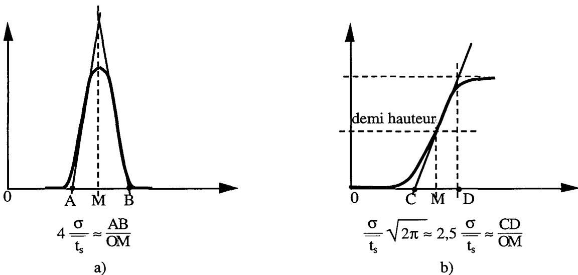
Figure 4.5 Méthodes graphiques de mesure des moments d'ordre 1 et 2 sur des courbes expérimentales symétriques. a) pic d'éluion, b) échelon frontal
