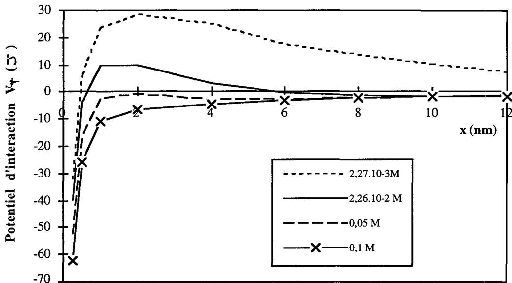
Figure 3.7 Potentiel d'interaction total pour des particules de latex de 0,23 μm en fonction de la concentration ionique en NaCl
