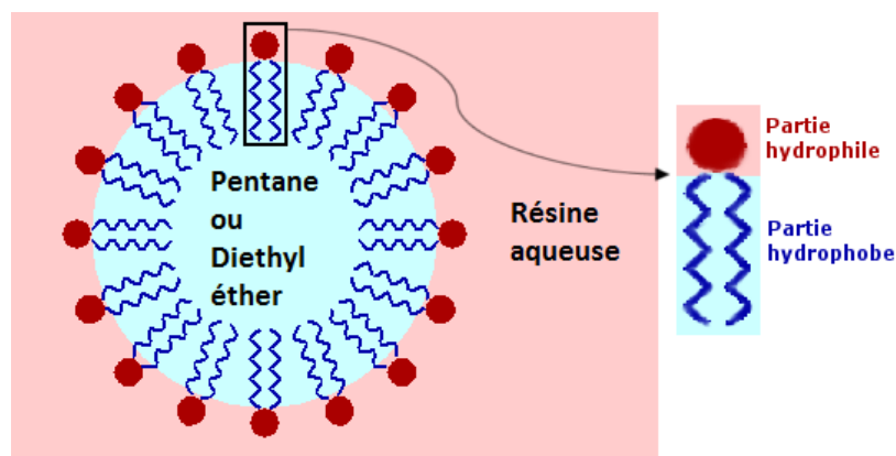
Figure 11: Emulsification de l'agent moussant (pentane ou diéthyl éther) au sein de la résine sous forme de micelles grâce à des tensioactifs.
