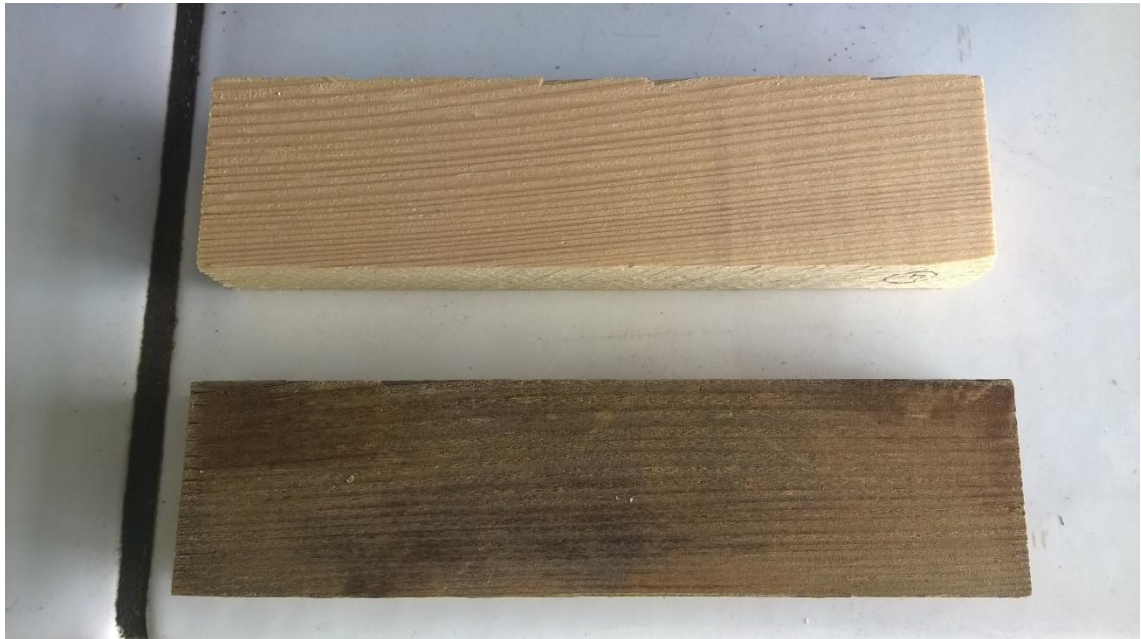
Figure 29: En haut, une pièce d'épicéa témoin; en bas celle qui a été imprégnée de mélange de tannins de châtaignier et de diméthyle carbonate, puis d'hexaméthylènediamine.
