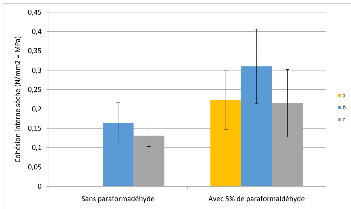
Figure 42: Cohésion interne sèche des panneaux de particules à base de résine de solution aqueuse tannins / huile de tournesol ozonisée: (a) une résine de solution tannins à 100%; (b) 90% de solution tannins et 10% d'huile ozonée pendant 480 minutes; (c) 90% de solution tannins et de 10% d'huile ozonée pendant 120 minutes.
