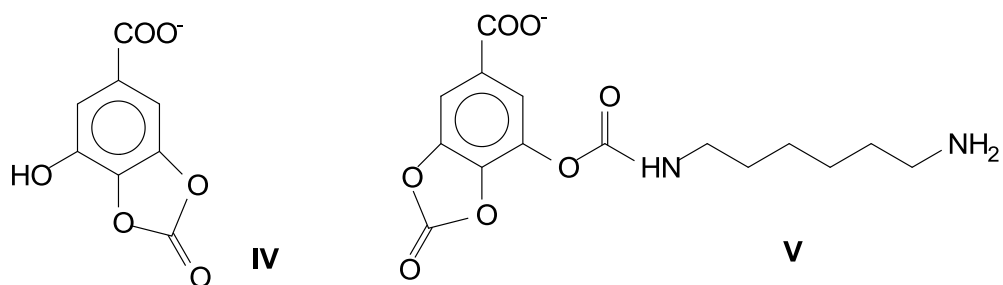
Figure 13: Formes de carbonates cycliques potentiellement obtenue par l'action du diméthyl carbonate sur l'acide gallique.
