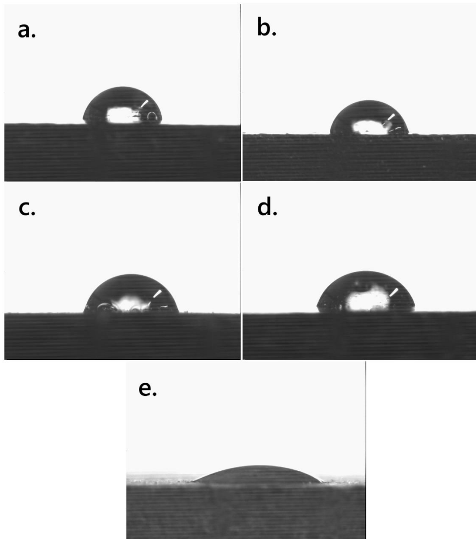
Figure 33: Position de gouttes d'eau sur les surfaces des revêtements de polyuréthane à base de tannins: (a) Mimosa; (b) Quebracho; (c) Pin Radiata; (d) Pin Maritime; (e) MDF non traité.
