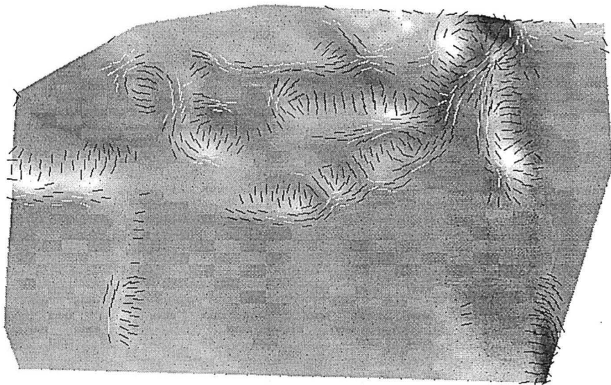
FIGURE 5-26 : Vecteurs de courbure \kappa_1
