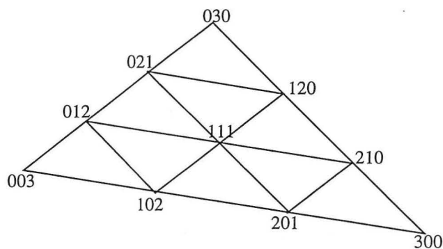
FIGURE 5-10 : «Control net» ou réseau de contrôle d'un patch de Bézier d'ordre 3
