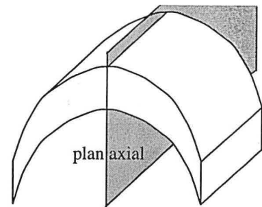
pli semblable
