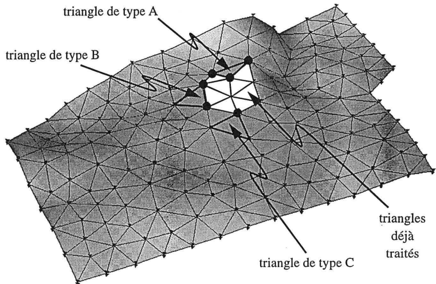
FIGURE 7-8 : types de triangles de l'auréole externe
