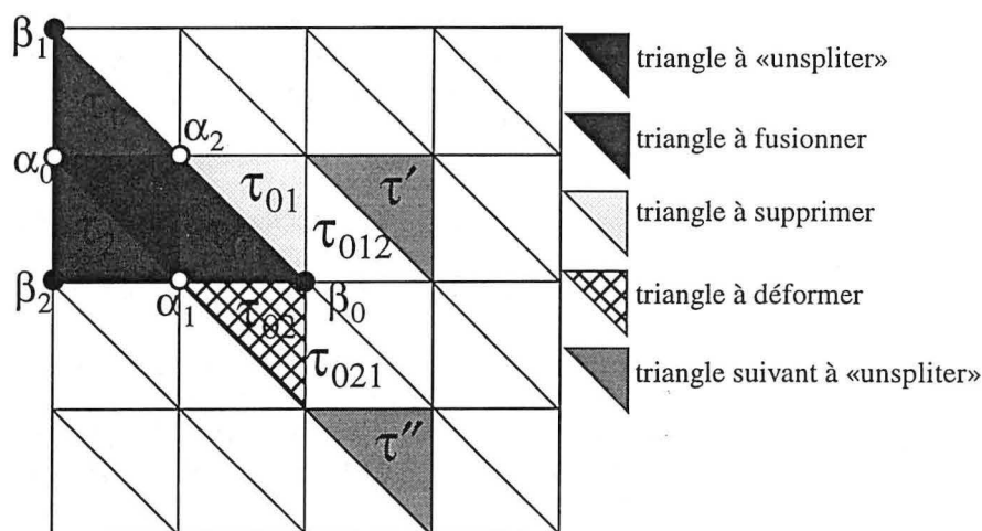
FIGURE 3-14 : Choix des triangles à «unspliter»
