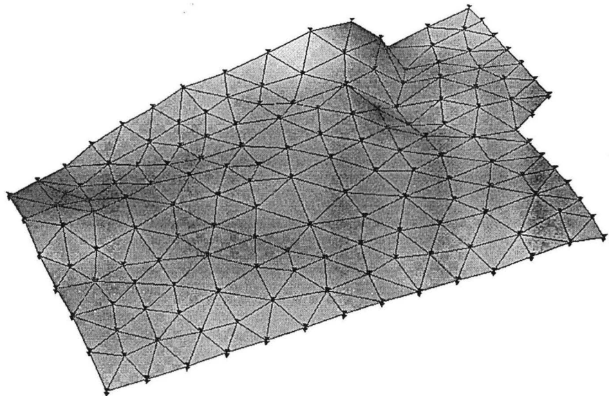
FIGURE 5-8 : Une surface triangulée gOcad, points et connectivités
