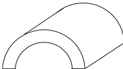
pli concentrique
