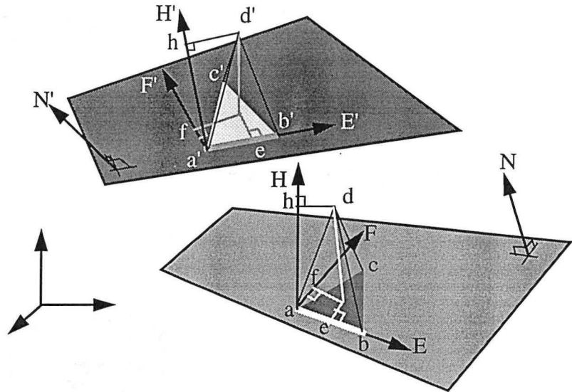
FIGURE 8-8 : Coordonnées locales d'un tétraèdre et préservation de l'épaisseur des couches
