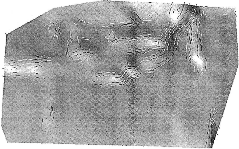
FIGURE 5-28 : Vecteurs de la courbure minimale
