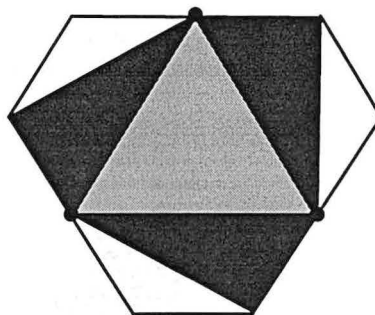
FIGURE 3-6 : maillage après «unsplit» d'un triangle
