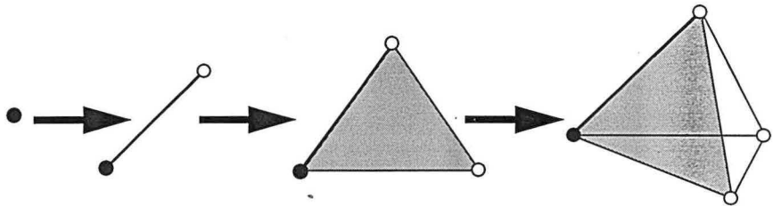
FIGURE 1-5 : Hiérarchie des simplexes définissant les objets gOcad
