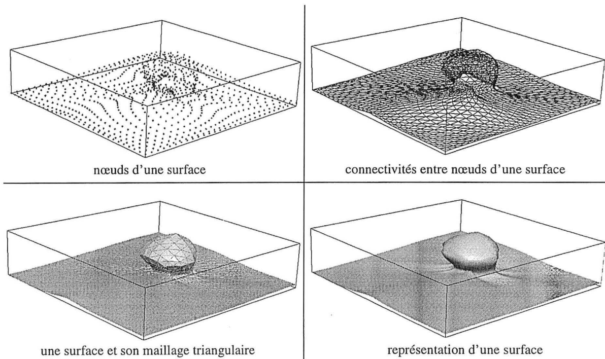
FIGURE 1-6 : Points, segments, triangles : une surface gOcad
