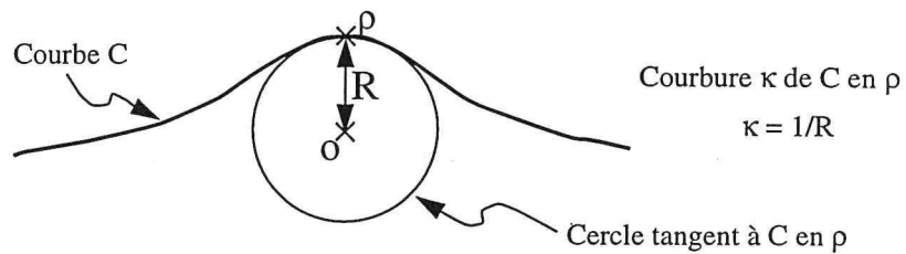
FIGURE 5-1 : définition de la courbure d'une courbe 2D (dans le plan)
