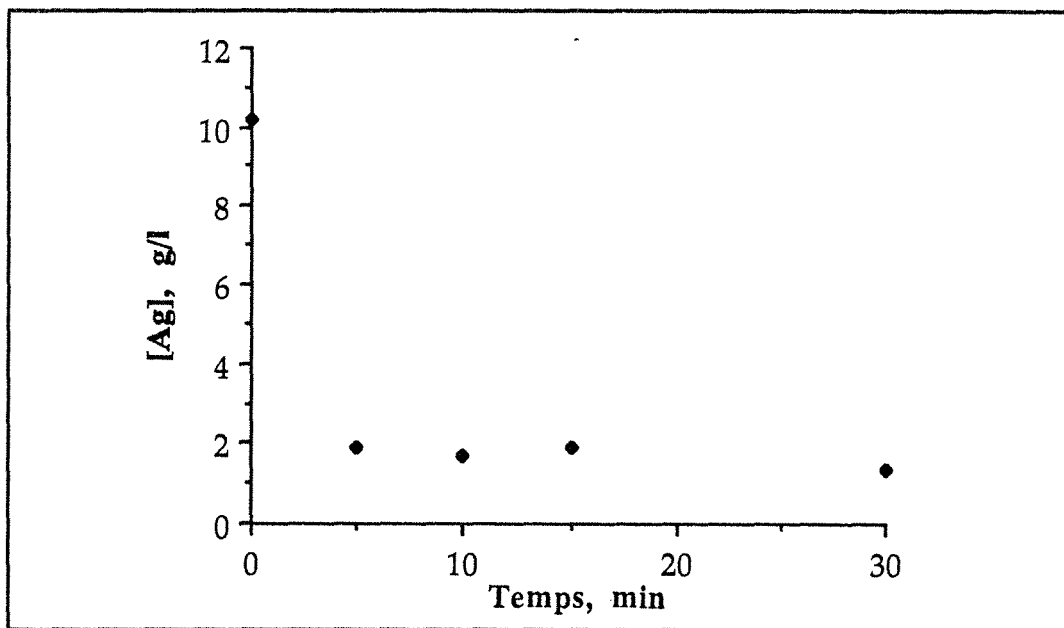
Figure IX-18 : Cimentation de l'argent sur poudre de cuivre, à partir des solutions de lixiviation des boues RTM en milieu nitrofluorosilicique.
