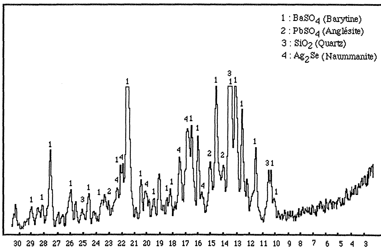
Figure VII-6 : Diffractogramme du résidu de lixiviation en milieu H_2SO_4 ( H_2SO_4 0,5M; L/S 11/1; T^\circ 100°C; P. atm.; Cond. 30 minutes).
