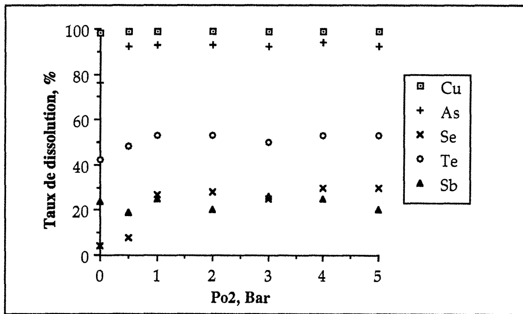
Figure VII-11 : Effet de la pression d'oxygène sur la lixiviation par autoclavage des boues anodiques RTM; H 2 SO 4 = 2,2M; L/S 22/1; T° 100 °C; Cond. 2 heures).
