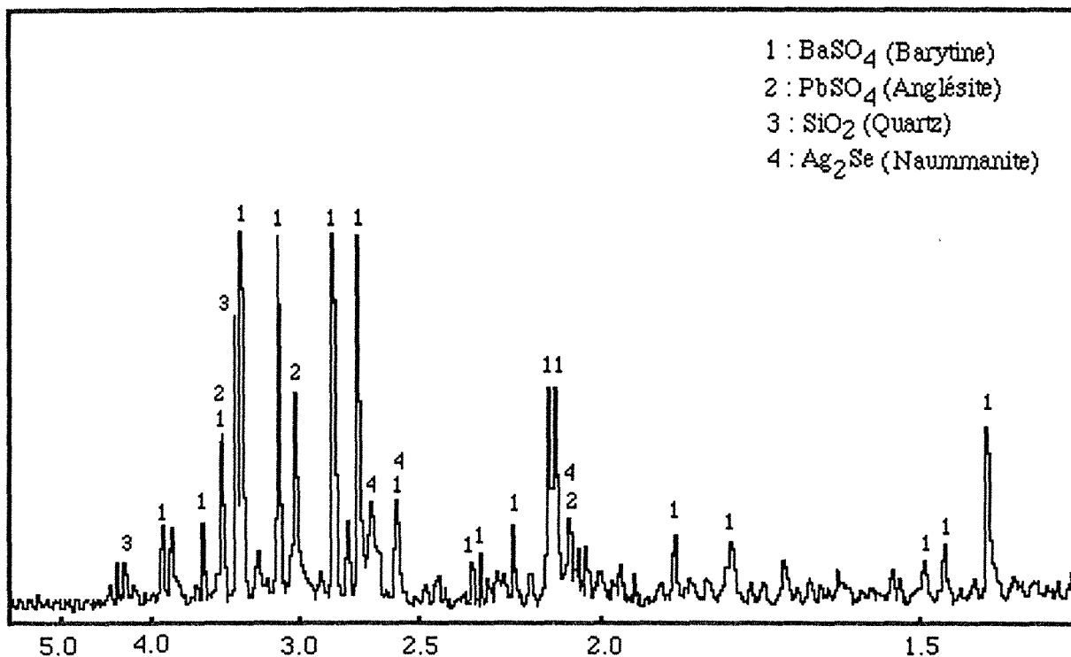
Figure VII-14 : Diffractogramme du résidu d'autoclavage sous pression d'oxygène, des boues anodiques RTM; H 2 SO 4 2,2M; L/S 12/1; T° 100 °C; Po 2 0,5 bars; Cond. 2 heures.
