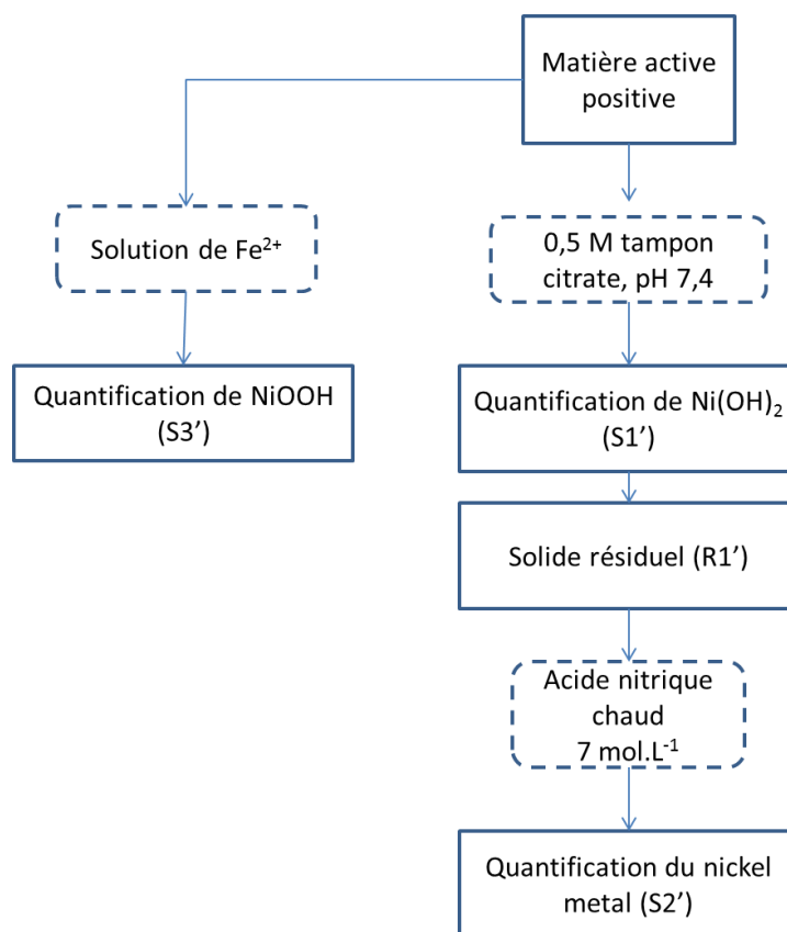
Figure 45 : solubilisation séquentielle sélective de NiOOH-Ni(OH)_2 et Ni^0
