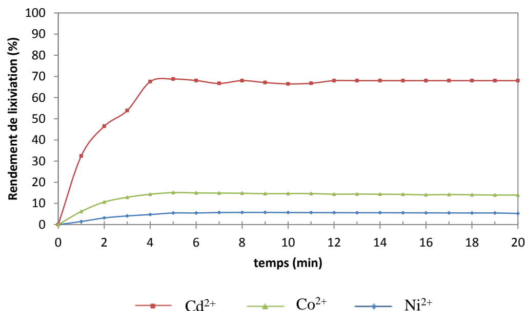
Figure 51 : évolution des rendements de lixiviation de la matière active reconstituée (H 2 SO 4 0,25 mol.L -1 )
