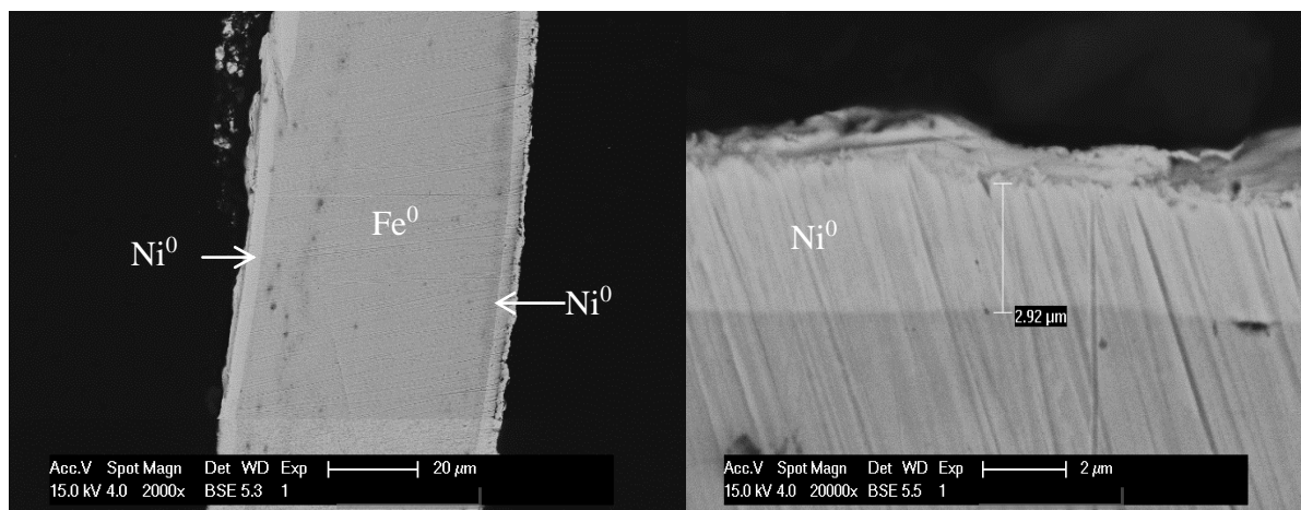
Figure 31 : images du support d'électrode obtenues par M.E.B.
