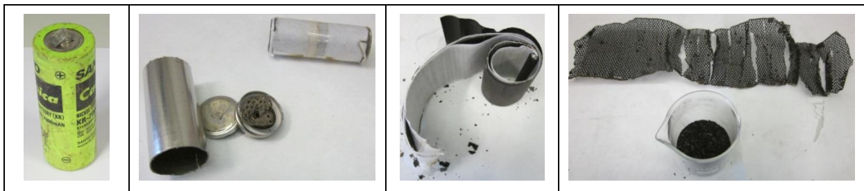
Figure 28 : démantèlement d'un accumulateur Ni-Cd
