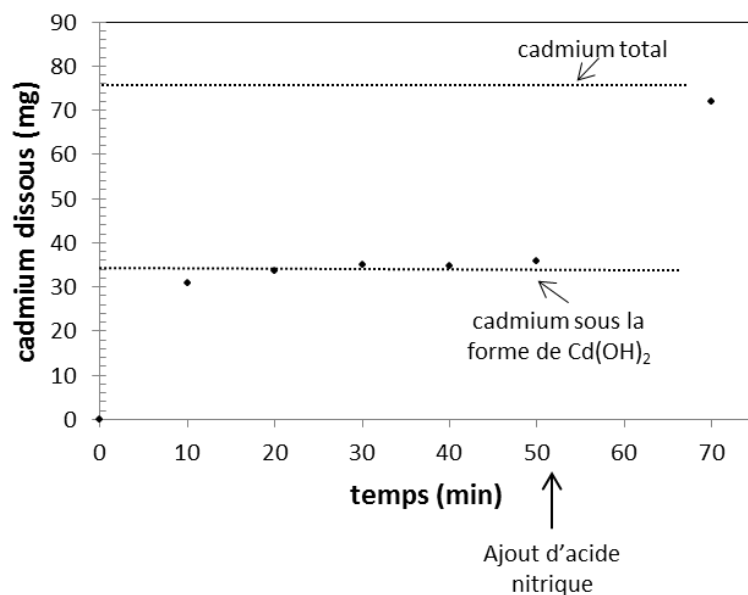
Figure 37 : spéciation du cadmium à partir d'un mélange synthétique \text{Cd(OH)}_2 - \text{Cd}^0
