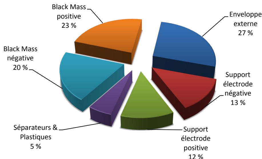
Figure 29 : composition moyenne des accumulateurs (% massique)
