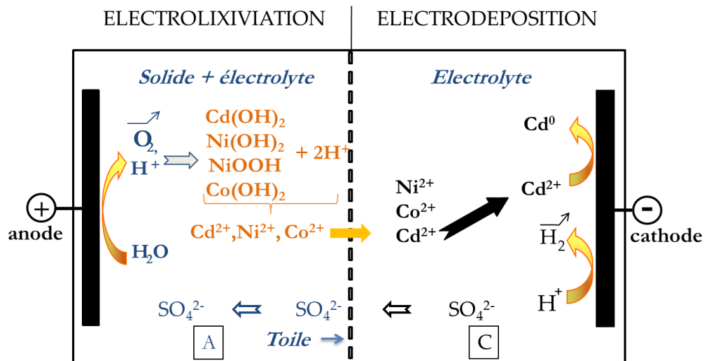
Figure 74 : principe de traitement de la matière active reconstituée par électrolixiviation/électrodéposition
