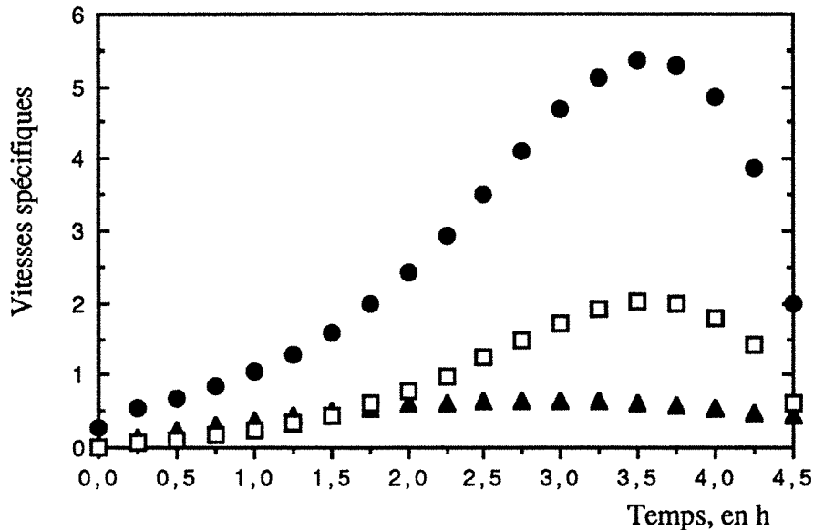
Figure 4 : Evolution des vitesses spécifiques calculées, en g de produit par g de matière sèche et par heure. Biomasse (▲), éthanol (◻) et glucose (●).
