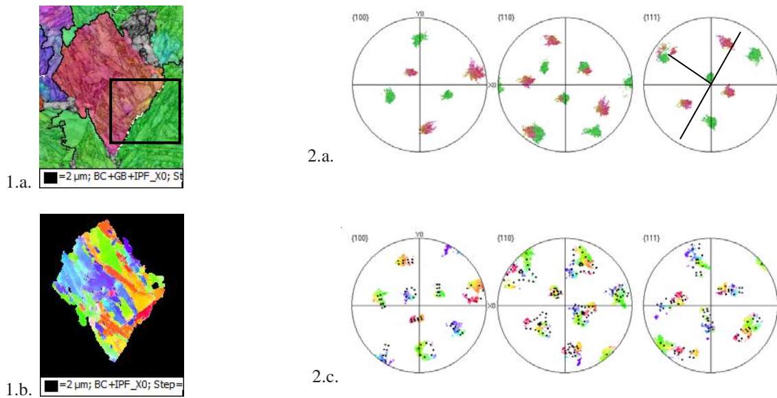
Figure IV.18 : Microstructure obtenue à \dot{\epsilon} = 0.1s^{-1} , \epsilon = 0.6 1) Carte d'orientation a) \gamma recalculée et b) \alpha héritée du grain \gamma rose, 2) Figures de pôles (AC=X0), a) des deux grains \gamma rose et vert situés dans l'encadré noir, ainsi que celle b) des variants théoriques hérités des grains \gamma rose superposés aux variants \alpha expérimentaux
