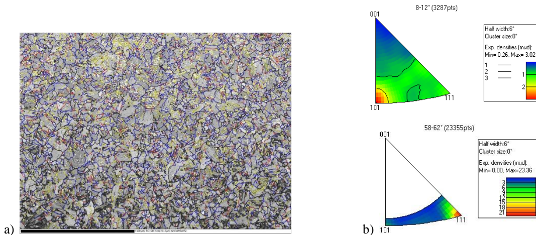
Figure III.30 : Microstructure de l'échantillon trempé avec \phi_\gamma=12\mu\text{m} a) Carte des désorientations angulaires, b) Axe de rotation des désorientations angulaires comprises entre 8 et 12°, entre 58 et 62°
