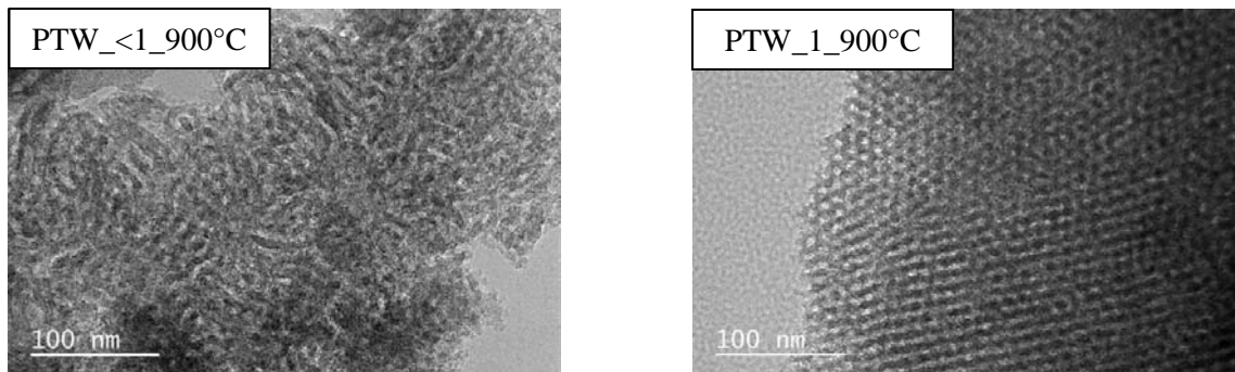
Fig. 11: Photos MET des carbones mésoporeux ordonnés préparés à partir de tanin soumis à HTC à pH très acide ( < 1 ; gauche) et 1 (droite) et pyrolyse postérieur à 900^\circ\text{C} .
