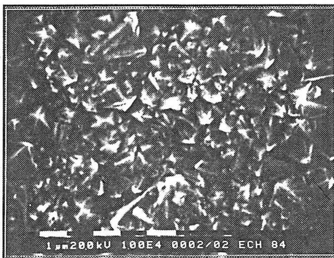
Figure IV.13. : effet de la température/densité de plasma (échantillon n°39)
