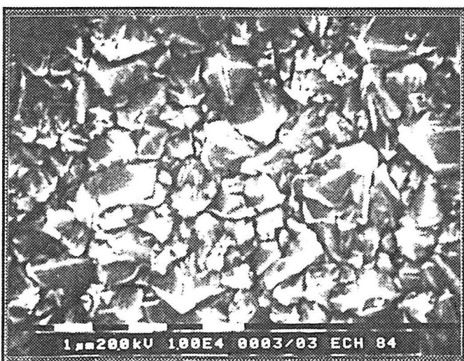
Figure IV.14. : effet de la température/densité de plasma (échantillon n°39)
