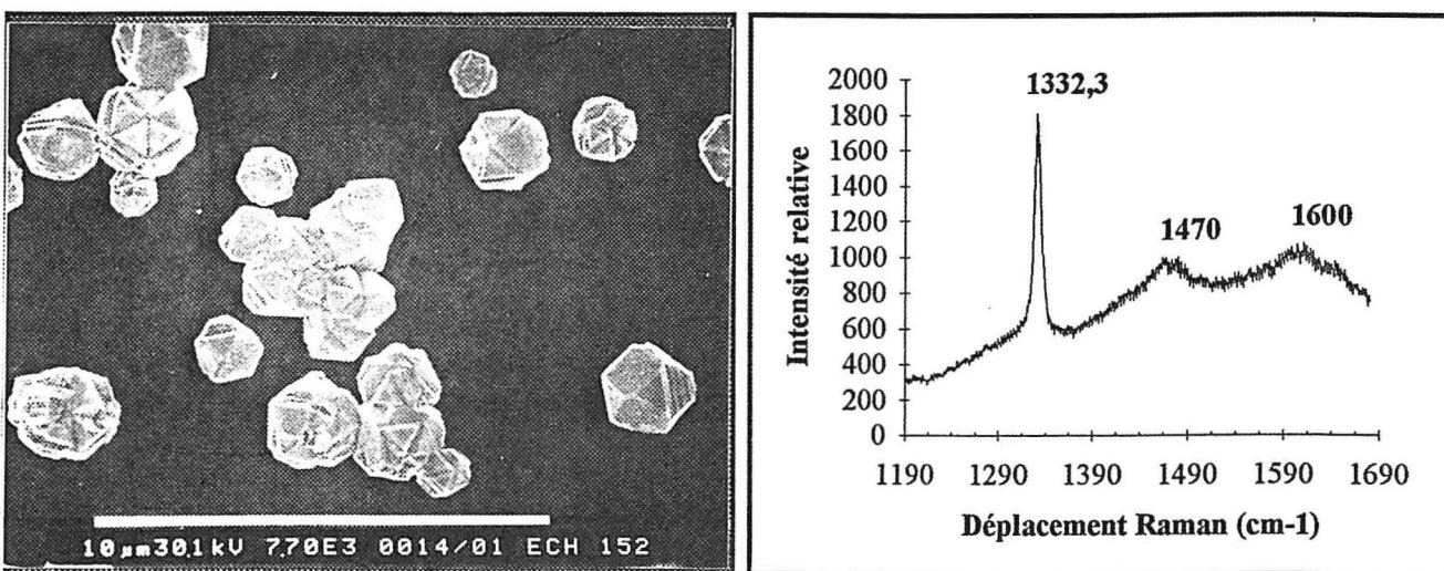
Figure III.14. : effet de la teneur en oxygène (échantillon n°6) Morphologie (MEB) et spectre Raman. [\text{O}_2] = 0,5 \text{ vol\%} , [\text{CH}_4] = 0,2 \text{ vol\%} , \bar{T} = 1150 \text{ K} .
