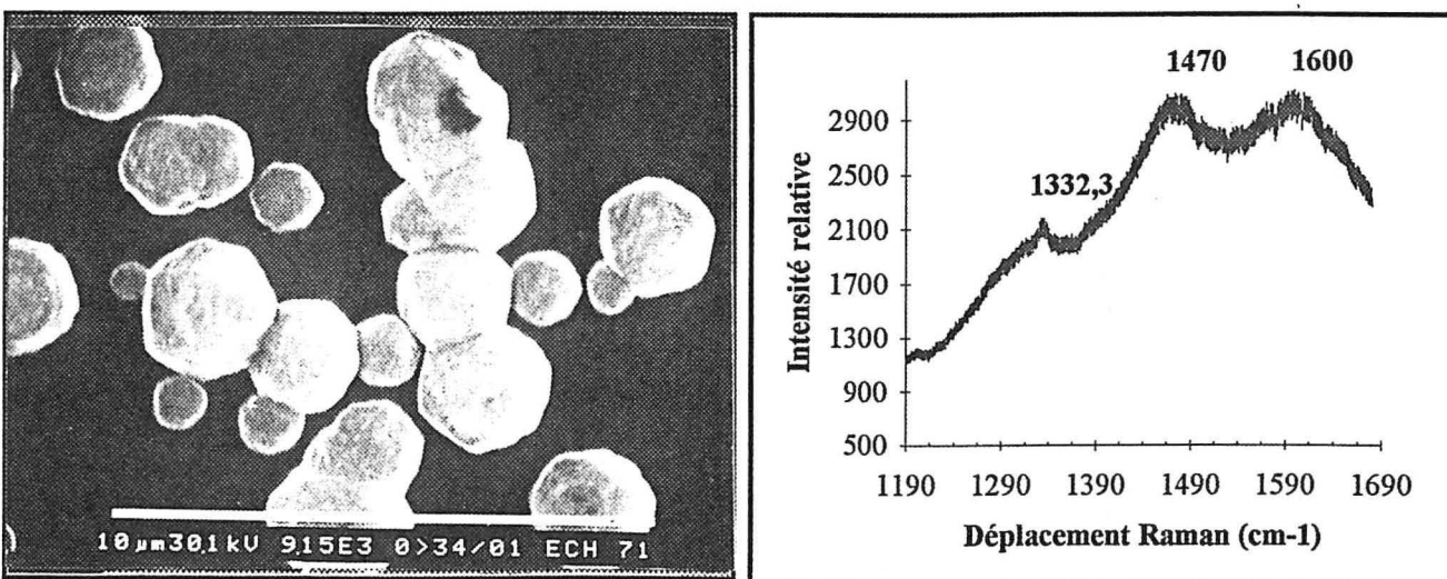
Figure III.17. : effet de l'argon (échantillon n°9) Morphologie (MEB) et spectre Raman. [Ar] = 10 \text{ vol\%} , [CH_4] = 1,5 \text{ vol\%} , \bar{T} = 1030 \text{ K} .
