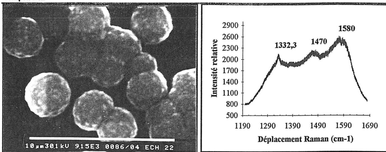
Figure III.12. : effet de la teneur en méthane (échantillon n°4) Morphologie (MEB) et spectre Raman. [\text{CH}_4] = 1,0 \text{ vol\%} , \bar{T} = 1000 \text{ K} .
