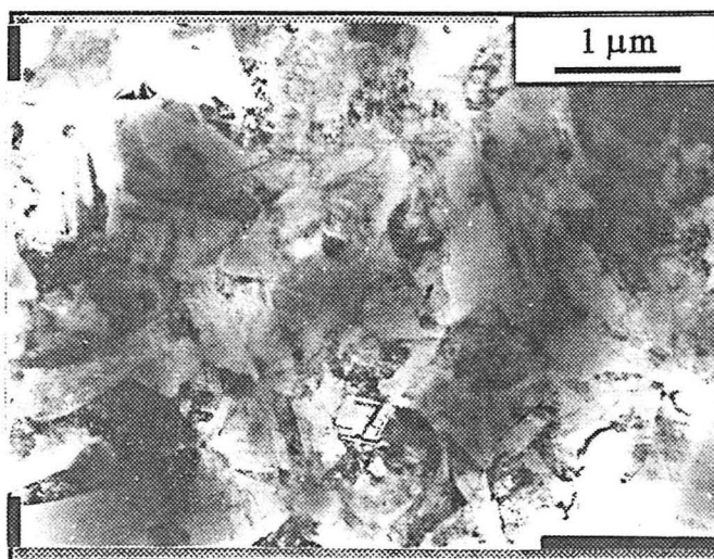
Figure IV.16. : effet de la température/densité de plasma (échantillon n°39) Micrographie en fond clair du dépôt dans la zone d'analyse A. [CH_4] = 0,4 \text{ vol}\% , \overline{T} = 1040 \text{ K} .
