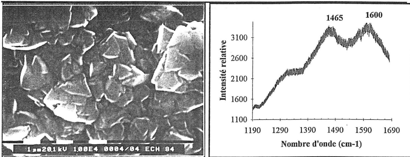
Figure IV.15. : effet de la température/densité de plasma (échantillon n°39) Morphologie (MEB) et spectre Raman de la zone d'analyse D. [CH_4] = 0,4 \text{ vol}\% , \overline{T} = 1040 \text{ K} .
