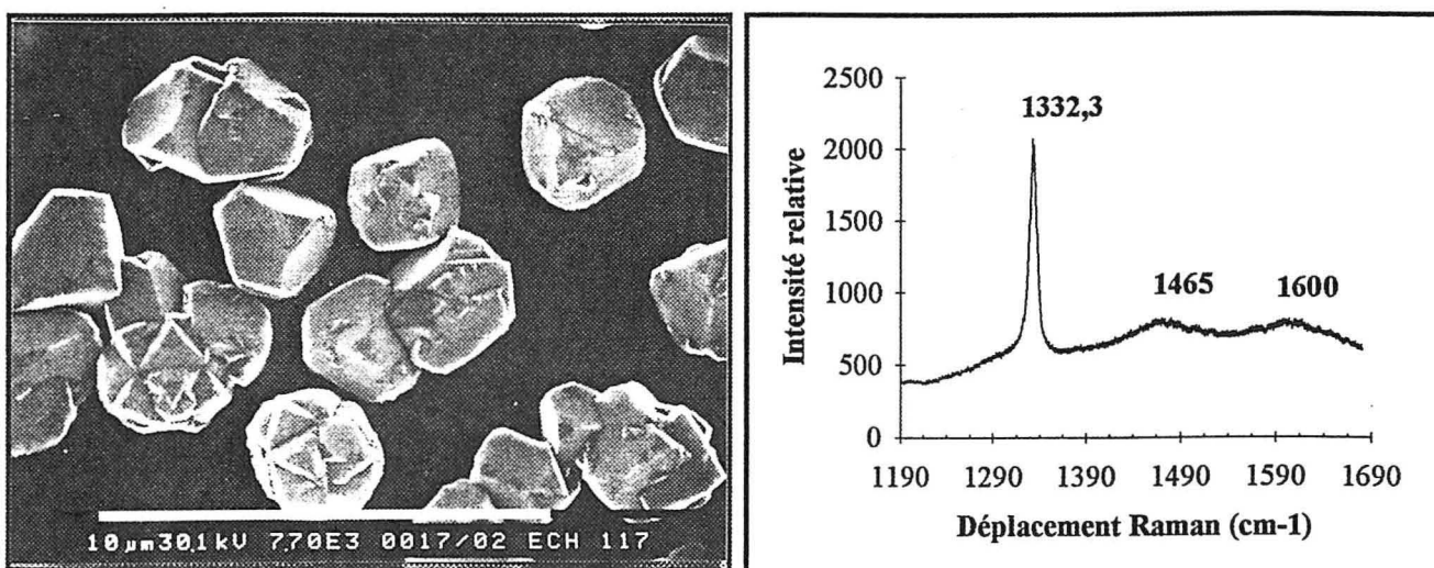
Figure III.13. : effet de la teneur en oxygène (échantillon n°5) Morphologie (MEB) et spectre Raman. [\text{O}_2] = 0 \text{ vol\%} , [\text{CH}_4] = 0,2 \text{ vol\%} , \bar{T} = 1150 \text{ K} .
