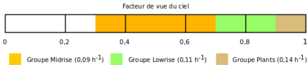
Figure 5.14 : Intervalles de valeurs de SVF associés aux groupes Midrise, Lowrise et Plants. Les valeurs moyennes de \chi_{DN}'' pour chaque groupe sont indiquées entre parenthèses.
