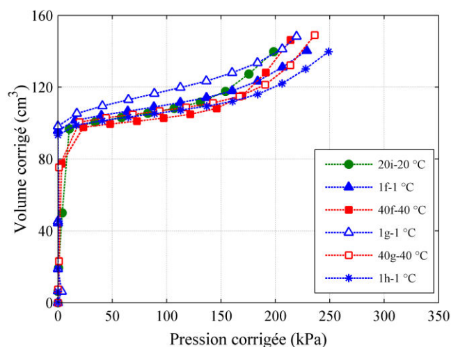
Figure IV.35. Courbes pressiométriques : essai de cycles thermiques (20-1-40-1-40-1-40 °C).
