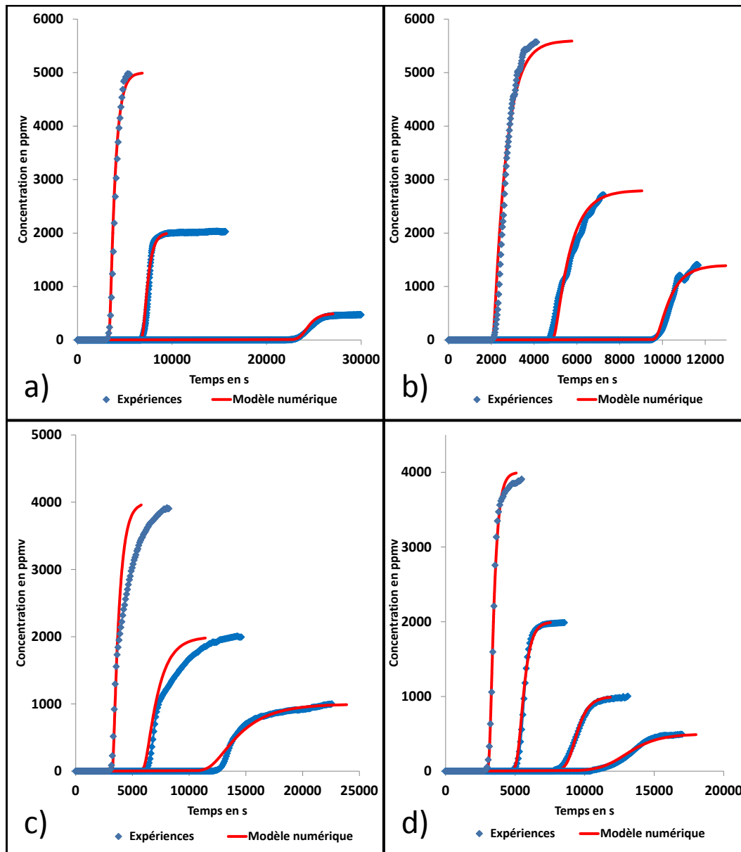
Figure 6.2.5 – Fronts de percée expérimentaux et simulés a) MEK, b) MIBK c) 1-Chloropentane, d) 2-Chloroisobutane
