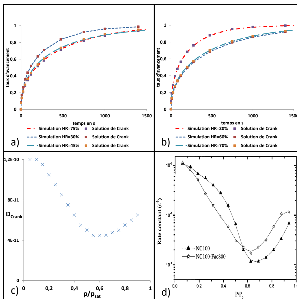
Figure 7.3.4 – Evolution du taux d'avancement en fonction du temps à différentes humidités relatives
