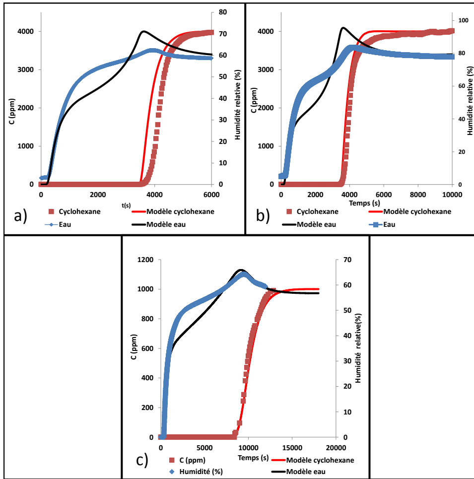
FIGURE 8.2.4 – Comparaison entre les fronts de percée expérimentaux et les fronts de percée simulés à 25°C a) Cyclohexane à 4000 ppmv et HR = 60% b) Cyclohexane à 4000 ppmv et HR = 80% c) Cyclohexane à 1000 ppmv et HR = 60%
