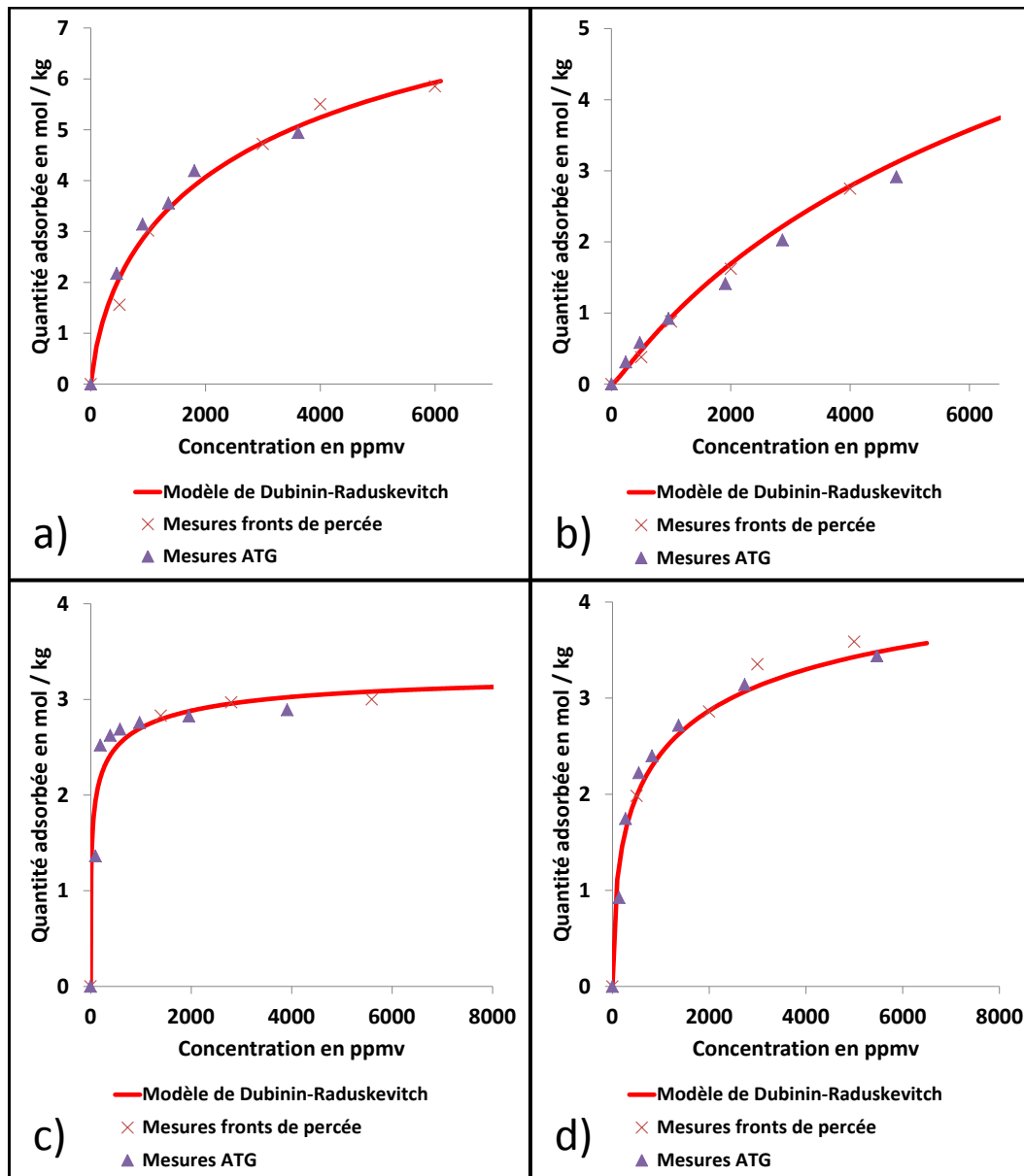
Figure 6.1.8 – Isothermes d'adsorption : résultats expérimentaux et modèle DR avec volume microporeux ajusté a) Ethanol, b) Acétonitrile c) MIBK, d) MEK
