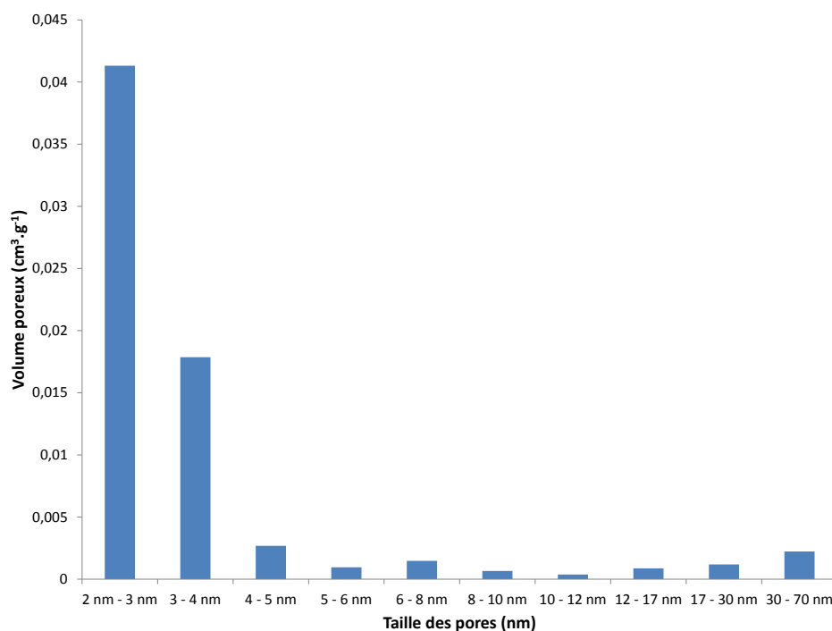
Figure 4.1.3 – Volume mésoporeux déterminé par la méthode BJH
