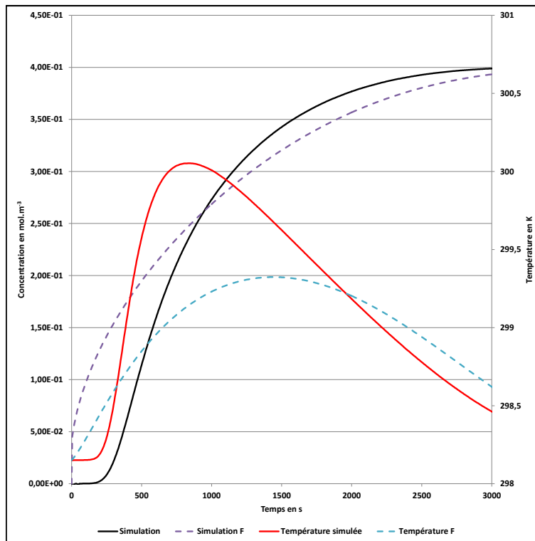
FIGURE 7.3.15 – Comparaison entre la modélisation avec l'équilibre de DS (traits pleins) et le modèle de Freundlich (traits pointillés), simulations à 30% d'HR à 25°C
