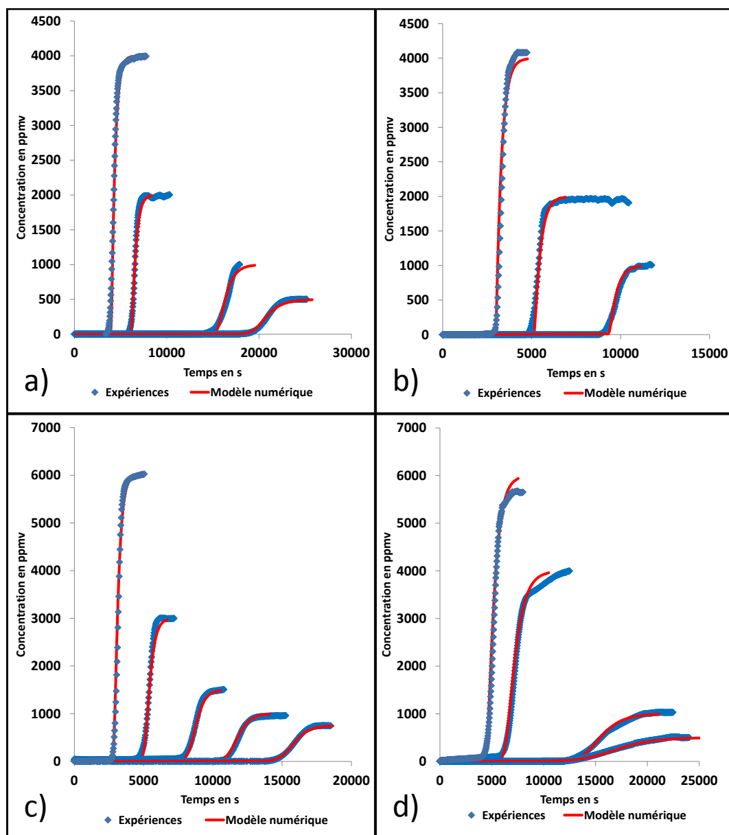
Figure 6.2.4 – Fronts de percée expérimentaux et simulés
