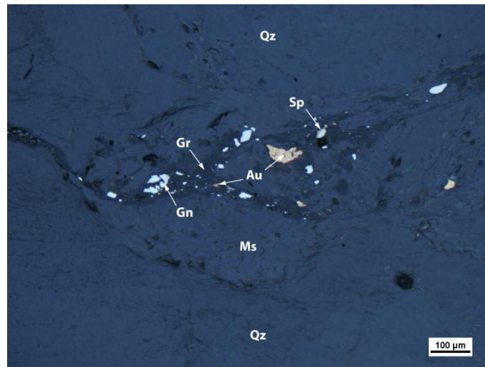
Figure 32 : Paragenèse minérale associée à l'or dans les fractures des veines de quartz (microscope optique, lumière réfléchie ; Qz : quartz, Ms : muscovite, Gn : galène, Gr : graphite, Sp : sphalérite)
