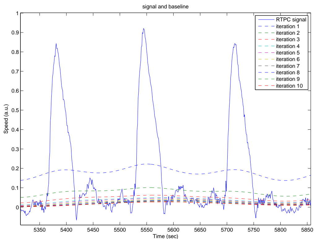
FIGURE 5.10 – Visualisation de l'évolution de la ligne de base en fonction des itérations de l'algorithme de calcul de la ligne de base du signal RTPC.
