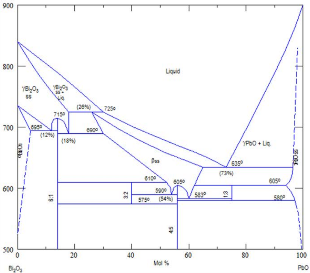
Figure A5-F2 : Diagramme d'équilibres de phases \text{Bi}_2\text{O}_3 - \text{PbO} d'après Biefeld et White [3]
