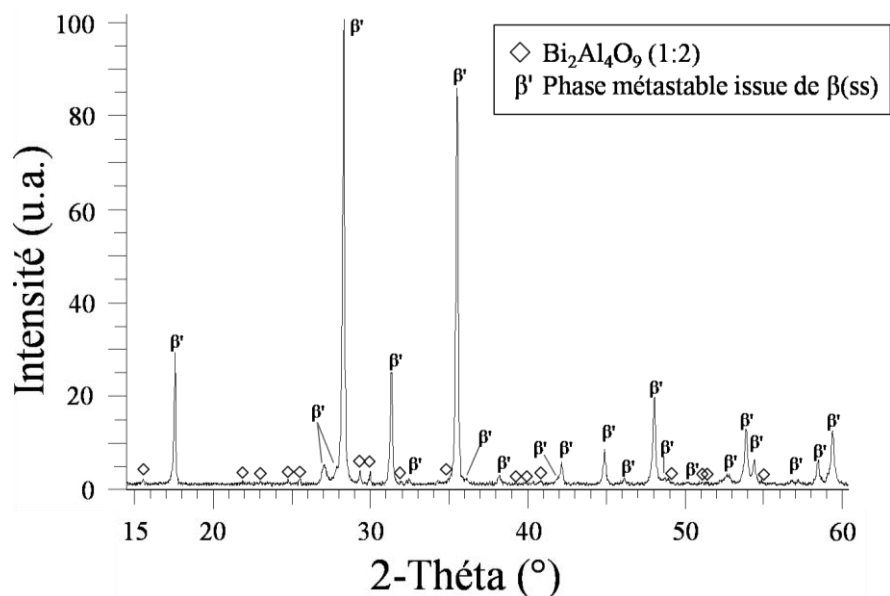
Figure V.10 : Diffractogramme X de l'échantillon #8 recuit pendant 1 semaine à 600°C sous une faible P_{\text{O}_2} ( \sim 10^{-15} atm) mettant en évidence un domaine biphasé (1:2) + β'
