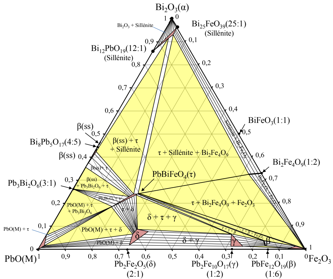
Figure VI.3 : Section expérimentale isotherme à 600°C sous air du système \text{Bi}_2\text{O}_3\text{--PbO--Fe}_2\text{O}_3
