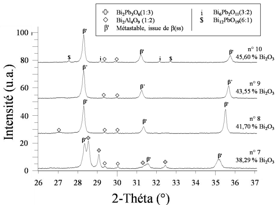
Figure V.11 : Diffractogramme X de la série d'échantillons #7 - #10 mettant en évidence une solubilité dans la phase métastable β'
