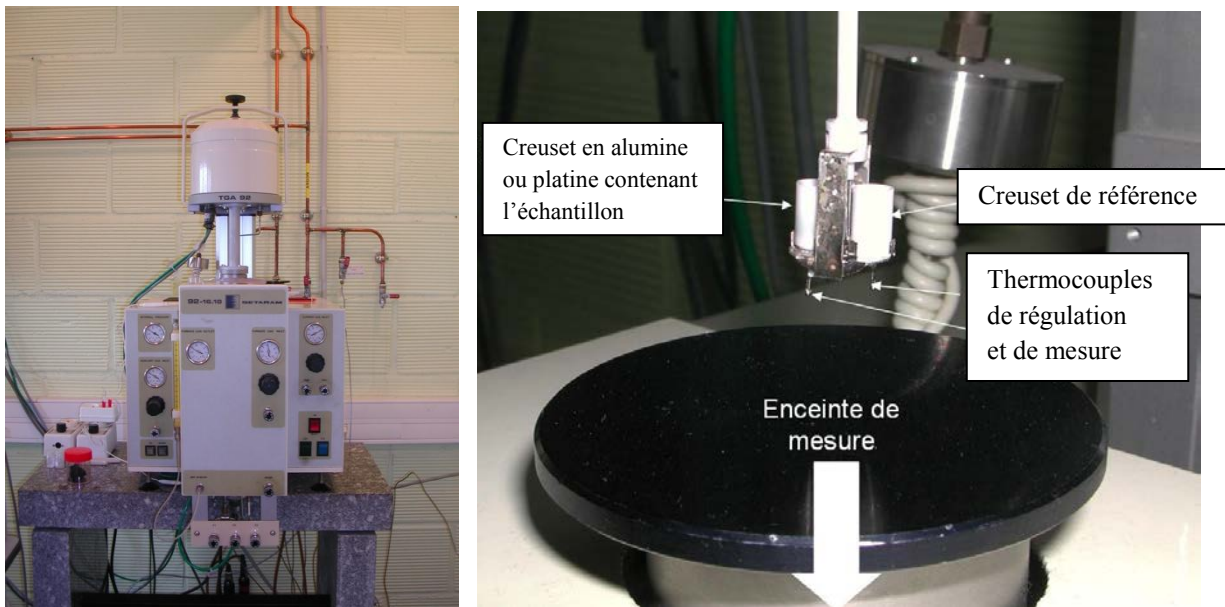
Figure I.5 : ATD-TG 92 (SETARAM) et ses composants
