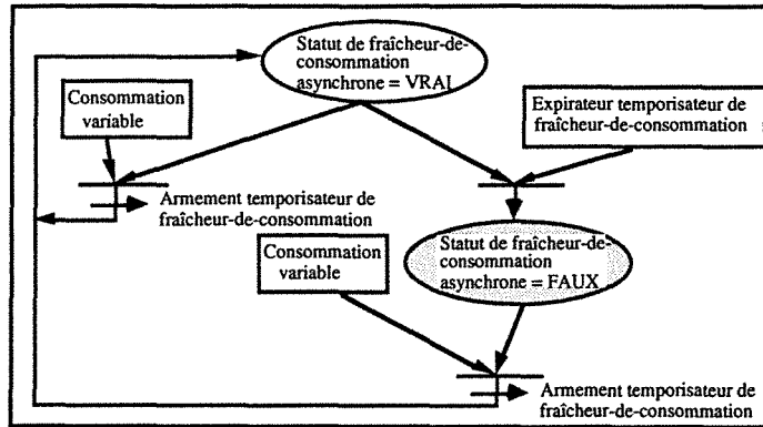
Fig. 5: Machine d'état pour la fraîcheur-de-consommation asynchrone
