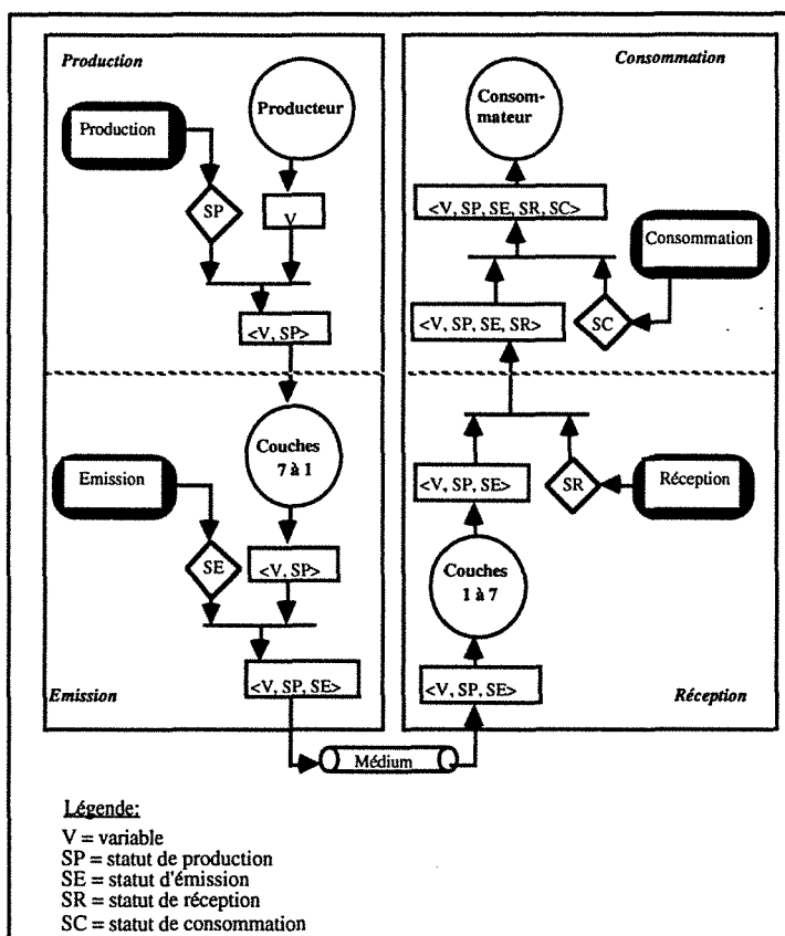
Fig. 3: Mécanismes d'élaboration des statuts temporels au cours de la communication
