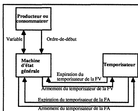
Fig. 10: Modèle de communication utilisé pour la validation
