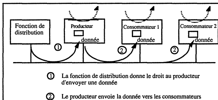
Fig. 1: Modèle de communication Producteurs/Distributeur/Consommateurs
