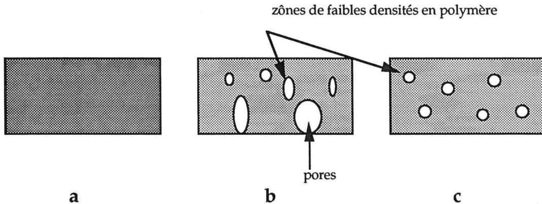
Figure 4.8 : Représentation schématique de la structure des membranes denses et asymétriques obtenus suite à des durées d'évaporation courtes et longues (face amont). (a) membrane dense ; (b) et (c) membranes asymétriques (durée d'évaporation 10 et 30 secondes)
