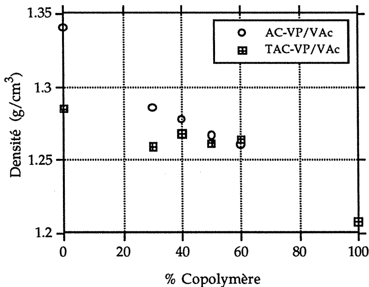
Figure 3.7 : Evolution des densités des alliages celluloses en fonction de la teneur en copolymère VP/VAc.
