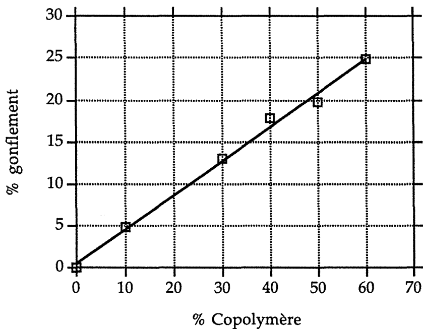
Figure 3.12 : Composition du liquide sorbée dans l'acétate de cellulose en fonction de la teneur en copolymère dans l'alliage. Composition du mélange test : 25 % en éthanol, T = 40\text{ °C} .
