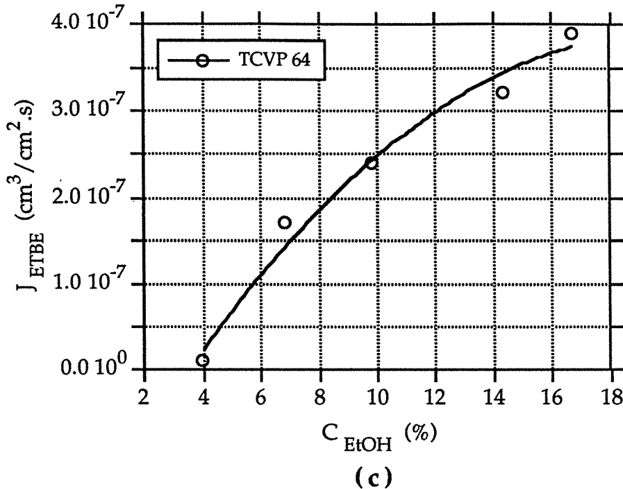
Figure 3.23 : Corrélations empiriques entre le flux d'ETBE et la fraction massique d'éthanol dans la membrane, à l'équilibre de sorption pour les différents alliages de TCVP.
