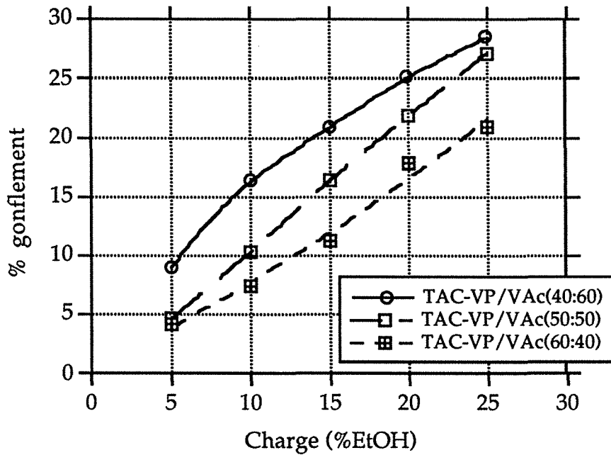
Figure 3.9 : Variation du taux gonflement de divers alliages cellulésiques en fonction de la composition du bain d'immersion ( T = 40\text{ }^{\circ}\text{C} ).
