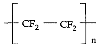
Polytetrafluoroéthylène
