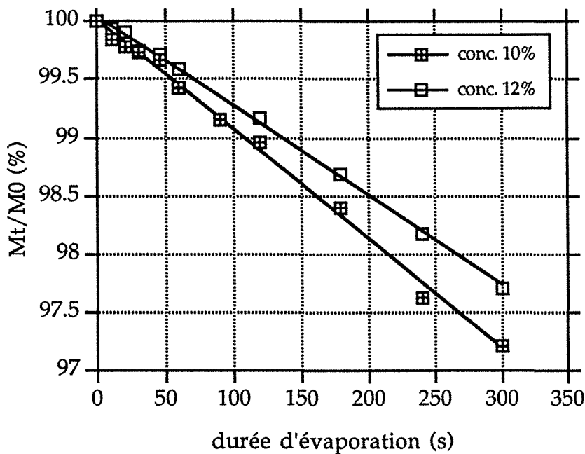
Figure 4.12 : Influence de la durée d'évaporation sur le perte de poids de films de collodions ACVP 55 disposés dans l'air immobile.
