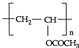
Polyvinylacétate
