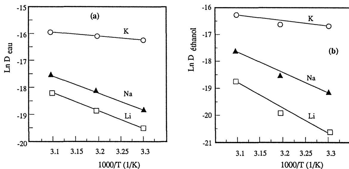
Figure 6.4: Variation des coefficients de diffusion de l'eau (a) et de l'éthanol (b) dans un mélange eau-éthanol contenant 10% en masse d'eau, en fonction de la température et la nature des contre-ions contenus dans les membranes carboxyliques. Epaisseur de la membrane: 35 \mu m
