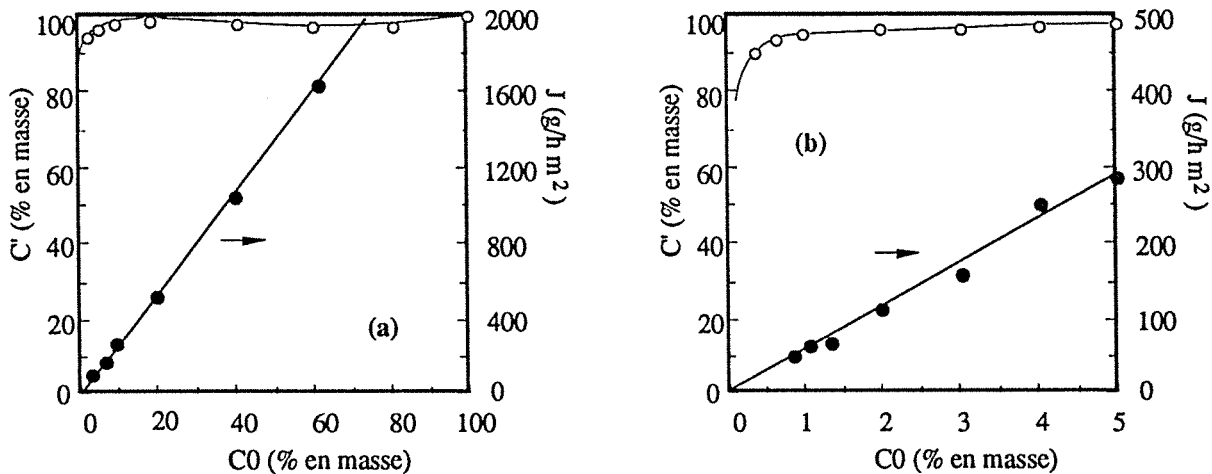
Figure 5.10: Fractionnement à 75°C d'un mélange eau-éthanol à travers une membrane composite en PVA réticulé par 5 % de glutaraldéhyde.
