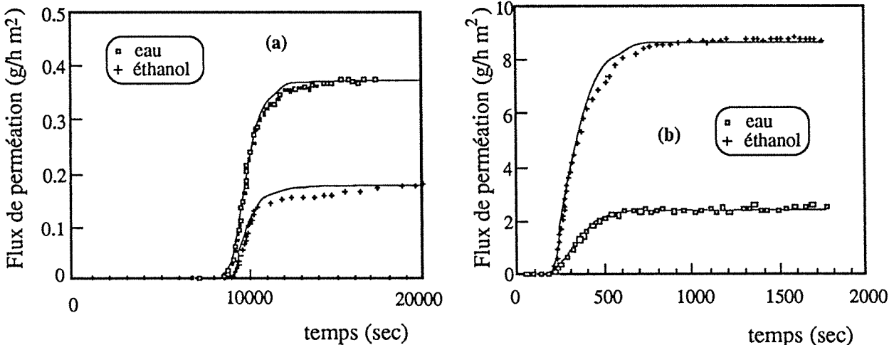
Figure 4.16: Variation des flux transitoires de l'eau et de l'éthanol d'un mélange (10:90) en fonction du temps à travers une membrane en PVA-PVP contenant (a) 20% et (b) 40% de PVP à 30°C. Épaisseur des membranes: 30 \mu\text{m}
