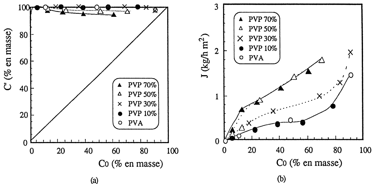
Figure 4.14: Teneur en eau dans le perméat (a) et flux de perméation (b) en fonction de la teneur en eau dans un mélange eau-THF en pervaporation à 30°C. Epaisseur de la membrane: 30µm
