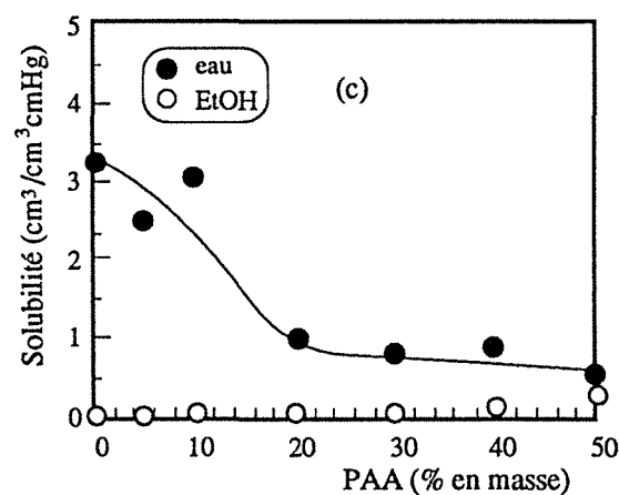
Figure 5.22: Variation des coefficients de diffusion (a), de perméation (b) et de solubilité (c) de l'eau et de l'éthanol à 50°C en fonction de la teneur en PAA dans les alliages PVA-PAA réticulés
