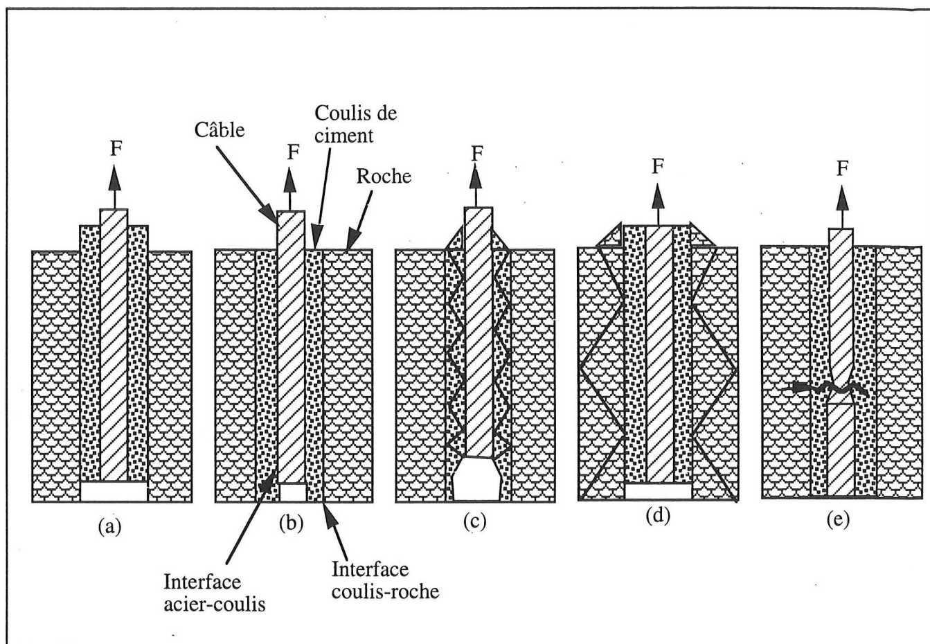
Figure 2.7 : Types de rupture d'un câble d'ancrage : a) rupture à l'interface roche-ciment, b) rupture à l'interface ciment-câble, c) rupture du ciment, d) rupture de la roche (tirée de Jeremic et Delaire, 1983) et e) rupture de l'acier
