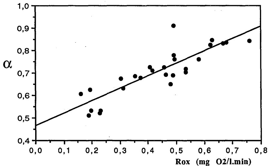
Figure III.2 : Influence de la vitesse de consommation de l'oxygène sur le facteur \alpha pour N=700 \text{ tr.min}^{-1}
