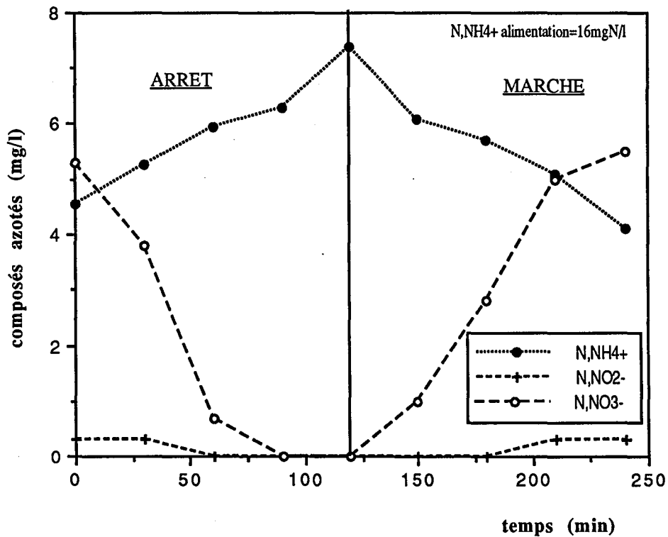
Figure III.15 : Evolution des composés azotés
