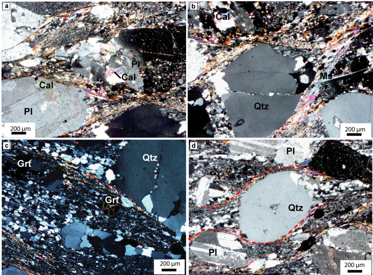
Figure 32: Microphotographie en lumière polarisée du Métagrauwaque (09MKZ12) de la série de zalbi.
