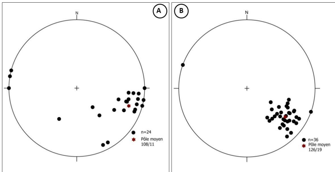
Figure 42: Stéréogramme des schistosités au sein des formations basiques.
