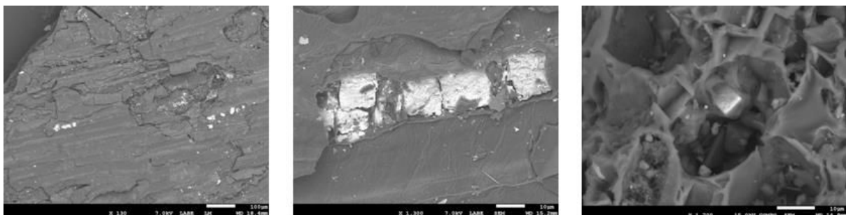
Figure 31 : Exemples de cristaux de calcite retrouvés après sorption des métaux en solution multiélément.
