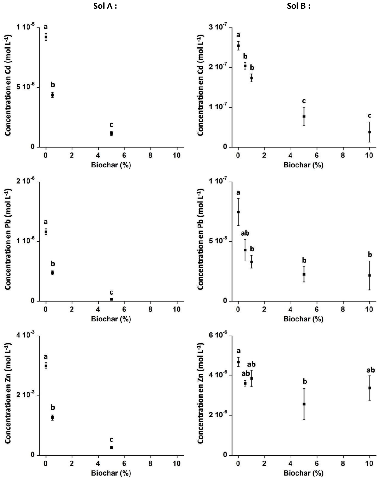
Figure 68 : Variation suivant la dose de biochar des concentrations de Cd (en haut), Pb (au milieu) et Zn (en bas) dans la solution du sol A (à gauche) et B (à droite). Les barres d'erreurs correspondent à l'erreur standard. Différentes lettres indiquent des différences significatives (Student-Newman-Keuls, p < 0,05 ).
