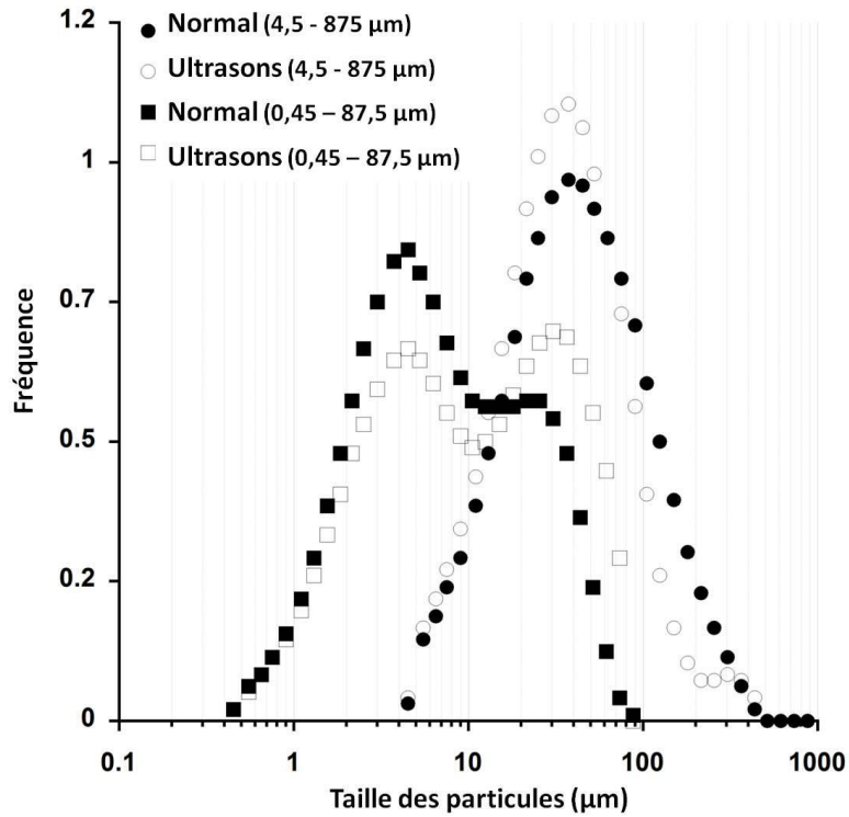
Figure 7 : Distribution volumétrique de taille de particules du biochar 1 tamisé à 500 µm, mesurée après 5 minutes d'agitation directement ("Normal") ou après traitement aux ultrasons ("Ultrasons") sur deux lentilles optiques spécifiques à une gamme de taille
