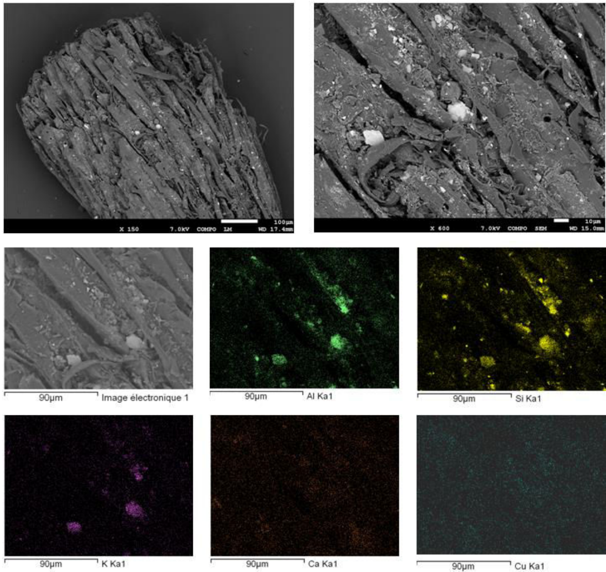
Figure 47 : Mapping en EDX d'une particule de bois feuillus peu ou pas pyrolysé récupéré après sorption de Cu en solution monoélément. Al, Si et K sont localisés dans des phases minérales bien précises, mais le Cu semble être présent uniformément en surface, sans lien avec le Ca.
