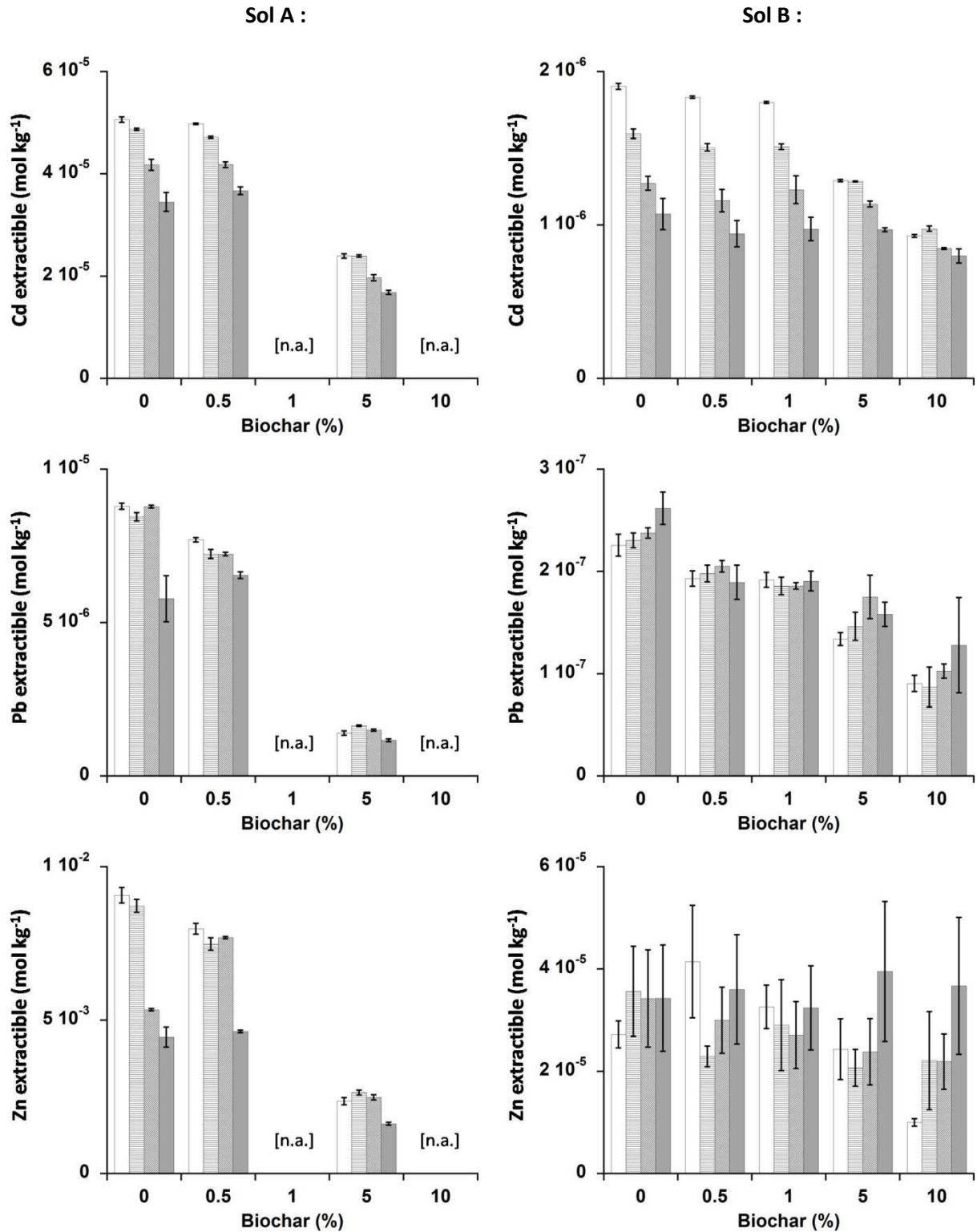
Figure 70 : Comparaison des quantités extractibles de Cd (en haut), Pb (au milieu) et Zn (en bas) entre modalité de couvert végétal suivant la dose de biochar, pour le sol A (à gauche) et B (à droite), à la fin de l'expérience 1. Blanc : sol nu ; Gris clair : sol global sous couvert de L. perenne ; Gris moyen : sol global sous couvert de N. caerulescens ; Gris foncé : sol de la rhizosphère de N. caerulescens . Les barres d'erreurs correspondent à l'erreur standard.
