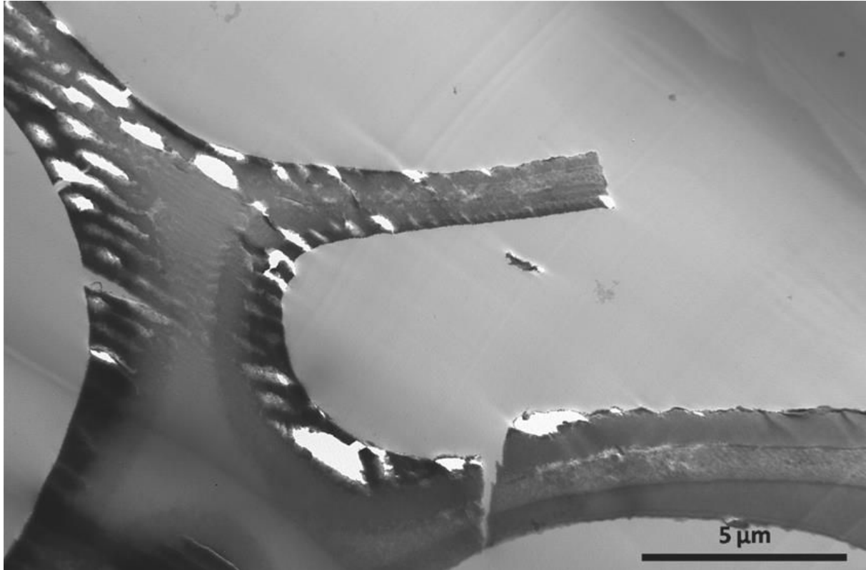
Figure 20 : Image au MET d'une particule de bois mal pyrolysé en coupe. Le gradient de texture apparent dans la paroi pourrait traduire des degrés de pyrolyse différents. Les bandes parallèles et les tâches blanches observées sont des artéfacts liés à la découpe de la lame ultra-mince.
