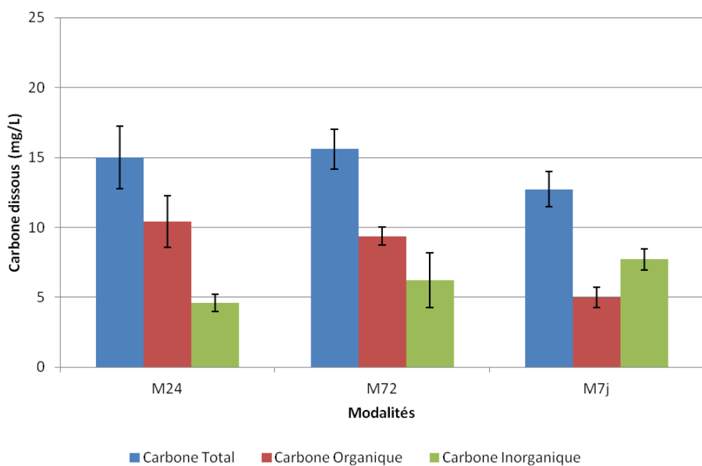
Figure 118 : Comparaison du paramètre "Durée de sorption" à 24h (M24), 72h (M72) et 7 jours (M7j) sur le carbone dissous en solution
