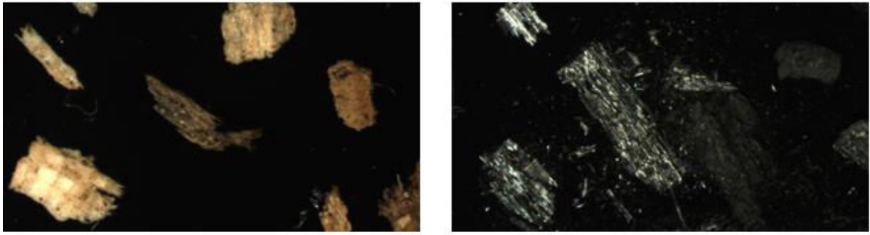
Figure 101 : Cliché prise sous la loupe binoculaire de copeaux de bois avant pyrolyse (à gauche) et du biochar 2 correspondant (à droite)
