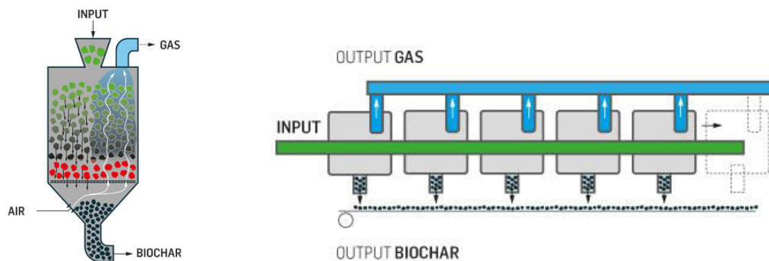
Figure 6 : Schéma du procédé de pyrolyse Schottdorf , avec description d'un four unitaire de pyrolyse (à gauche) et d'un assemblage de fours en série (à droite). Source : Carbon terra GmbH
