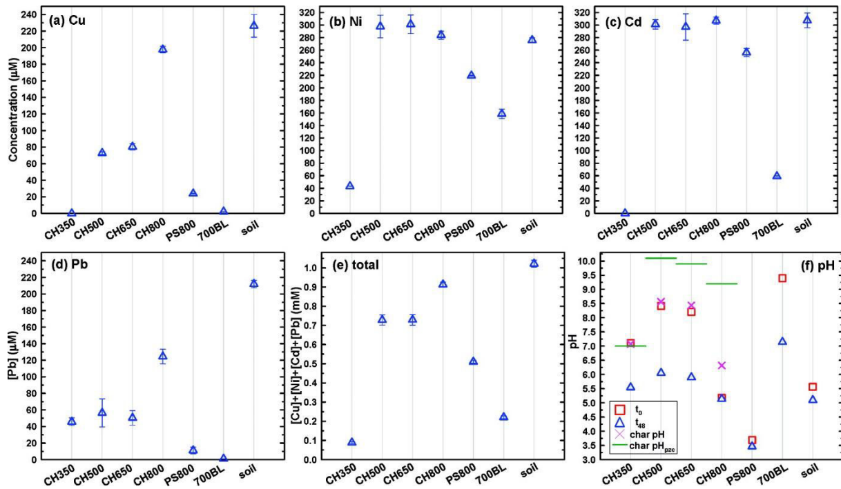
Figure 4 : Exemple de l'effet de la température de pyrolyse et de la nature du charbon sur la concentration de Cu, Ni, Cd et Pb résiduelle en solution 48h après leur introduction dans une suspension de sol sablo-limoneux non contaminé amendé à 10 % en masse de biochar. Le pH initial (carré) et final (triangle) des suspensions est indiqué dans le graphe (f), ainsi que le pH du biochar et le pH correspondant au point de charges nulles. CH350-800 : biochar issu de résidus de coton pyrolysé entre 350 et 800°C ; PS800 : charbon actif obtenu par pyrolyse à 800 °C d'enveloppes de noix de Pécan et traité à l'acide phosphorique ; 700BL : biochar issu de litière animale pyrolysée à 700°C ; soil : suspension de sol sans biochar. Source : (Uchimiya et al. 2011d).
