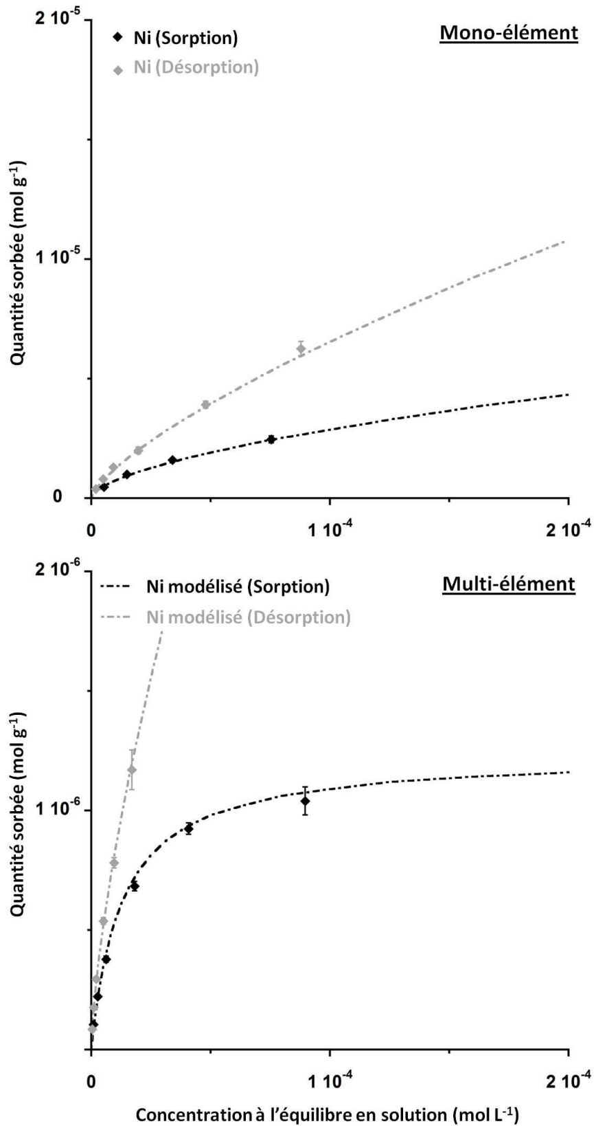
Figure 28 : Variations des quantités de Ni sorbé sur le biochar 1 avec leur concentration en solution à l'équilibre dans Ca(NO 3 ) 2 0,01M en solution mono-élément (en haut) et multiélément (en bas). En noir : courbes de sorption; en gris : courbes de désorption. Les courbes correspondent au modèle de Freundlich (monoélément + Ni dés multi ) ou de Langmuir. Les barres d'erreurs représentent l'erreur standard.
