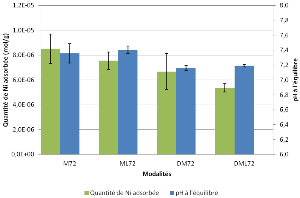
Figure 113 : Comparaison du paramètre "Lavage" sur la quantité de Ni adsorbée (M72 : sans lavage, ML72 : avec lavage) et désorbée (DM72 : sans lavage, DML72 : avec lavage) ainsi que sur le pH
