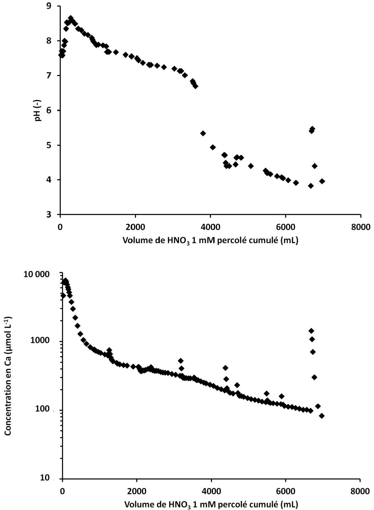
Figure 61 : Evolution du pH (en haut) et de la concentration de Ca (en bas) en sortie de la colonne de biochar en fonction du volume de HNO 3 1 mM apporté cumulé. L'effet des arrêts et reprises d'écoulement est visible à travers les discontinuités positives observées sur les courbes.
