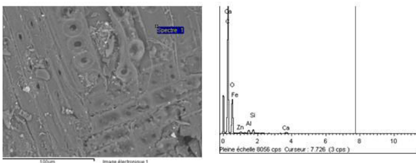
Figure 46 : Analyse EDX d'une particule de bois résineux peu ou pas pyrolysé récupéré après sorption de Zn en solution monoélément. L'analyse révèle que le Zn est présent en présence d'aluminium, de silicium et de Ca à un endroit a priori non relié à une phase minérale précise.
