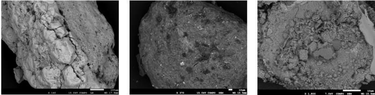
Figure 21 : Images au MEB de trois particules minérales présentes dans le biochar 1, avec Si, Ca, Fe, Al et d'autres éléments.
