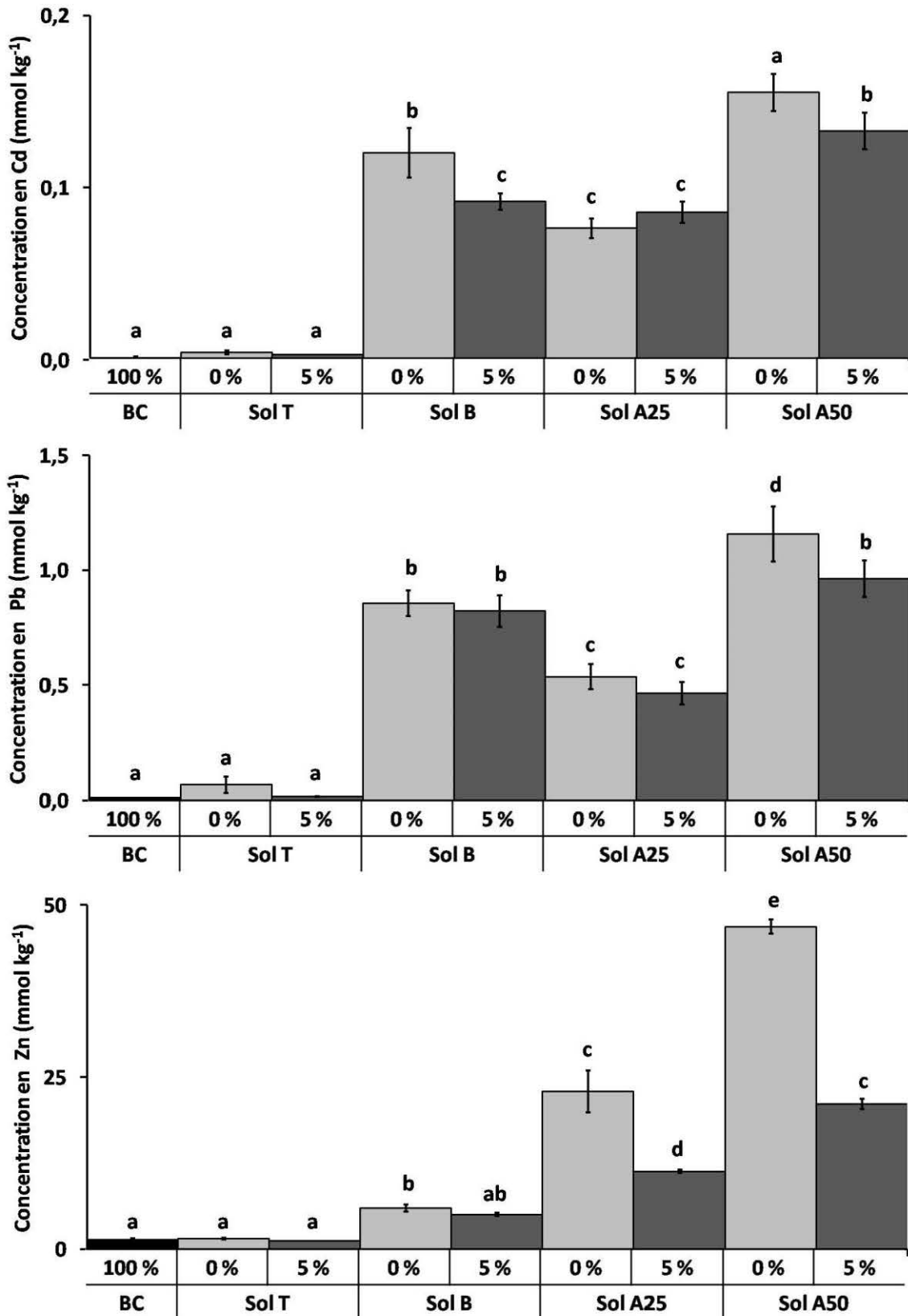
Figure 89 : Concentration de Cd (en haut), Pb (au milieu) et Zn (en bas) dans les racines secondaires de V. faba après 7 j d'exposition à différents substrats. BC : biochar pur ; T : sol témoin ; A25 : A mélangé à 25 % dans T ; A50 : A mélangé à 50% avec T. Les barres d'erreurs correspondent à l'erreur standard. Différentes lettres indiquent des différences significatives (Student-Newman-Keuls, p < 0,05 ).
