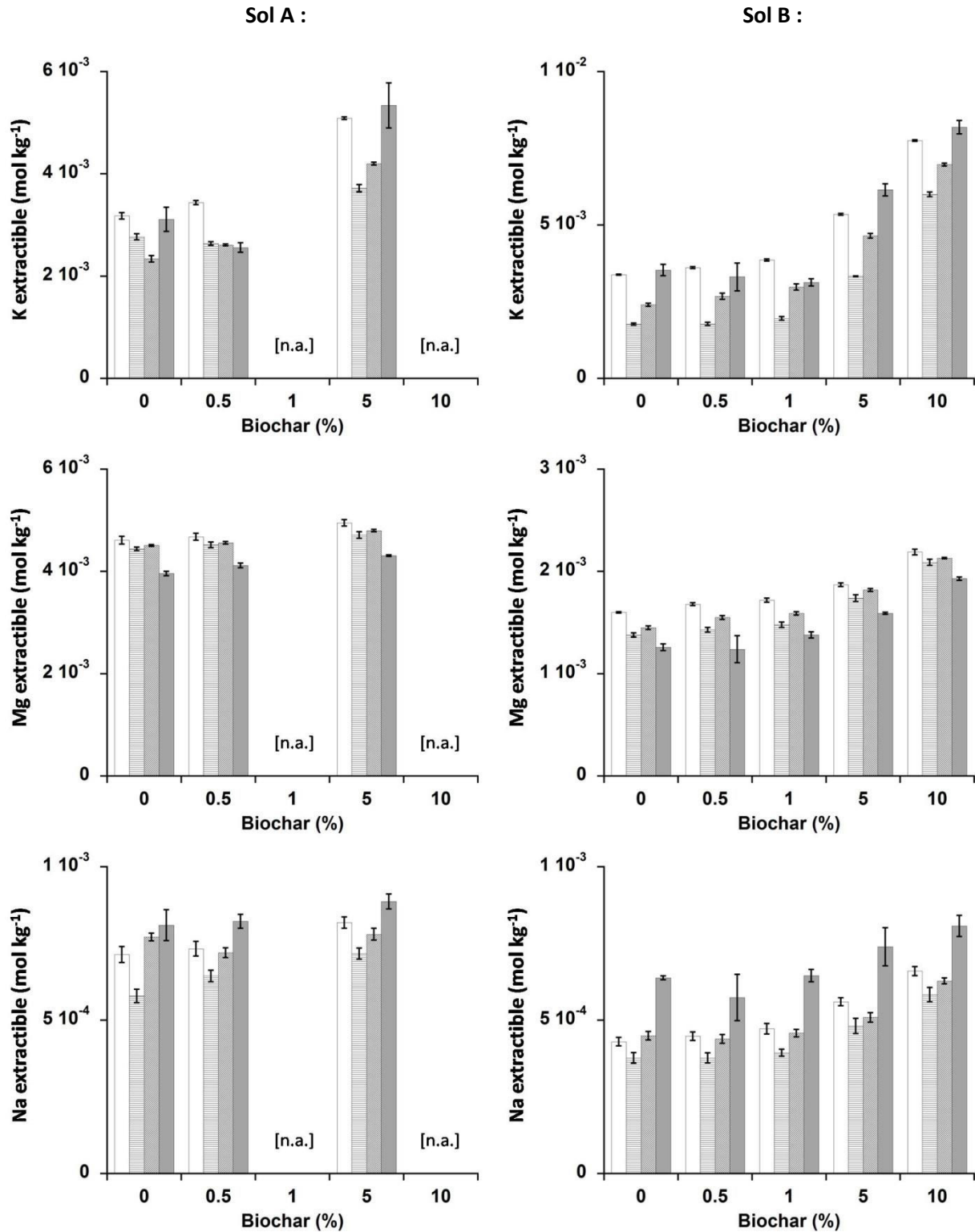
Figure 71 : Comparaison des quantités extractibles de K (en haut), Mg (au milieu) et Na (en bas) entre modalité de couvert végétal suivant la dose de biochar, pour le sol A (à gauche) et B (à droite), à la fin de l'expérience 1. Blanc : sol nu ; Gris clair : sol global sous couvert de L. perenne ; Gris moyen : sol global sous couvert de N. caerulescens ; Gris foncé : sol de la rhizosphère de N. caerulescens . Les barres d'erreurs correspondent à l'erreur standard.
