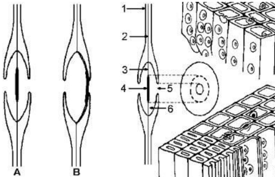
Figure 10 : Schéma d'une ponctuation aréolée présente sur les trachéides des bois résineux. A : aspect normal sans aspiration ; B : Aspiration du torus lors du séchage. 1 : paroi de la trachéide ; 2 : lamelle intermédiaire ; 3 : bord membraneux ; 4 : torus ; 5 : ouverture de l'aréole ; 6 : chambre de l'aréole (Usta 2010)
