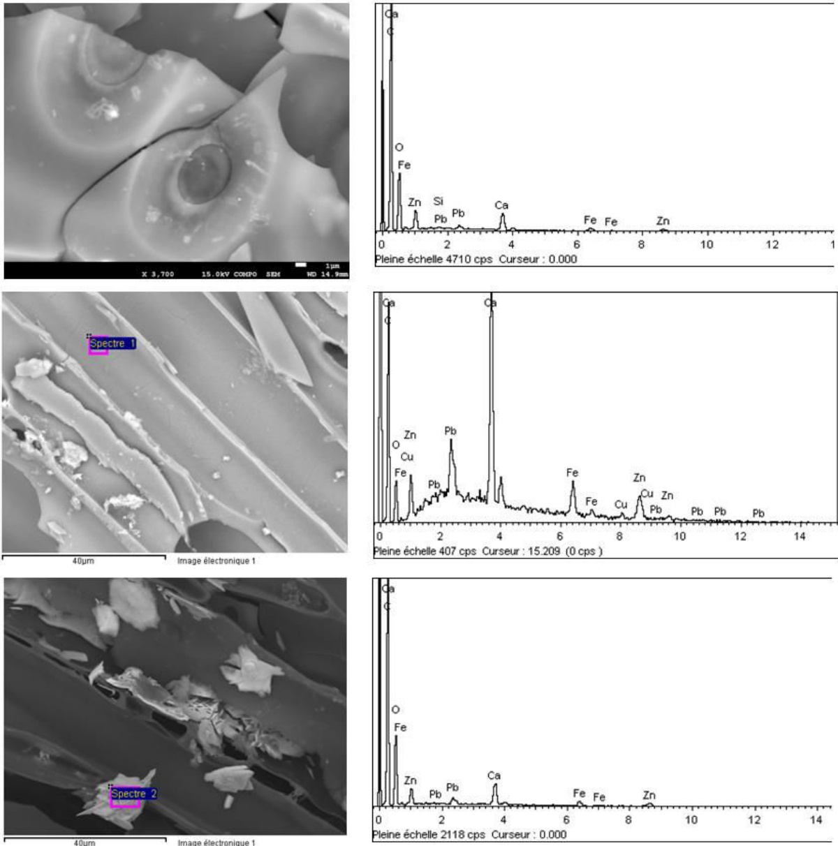
Figure 130 : Images MEB et analyse EDX de copeaux de charbon de bois retrouvés dans le sol contaminé A. Zn, Pb et Cu sont détectés en présence de Ca à la surface d'aréoles (en haut), de trachéides (au milieu) et sur une particule minérale avec Fe (en bas). Des plaques contenant Ba, S et des traces de Zn sont également repérées (en bas).
