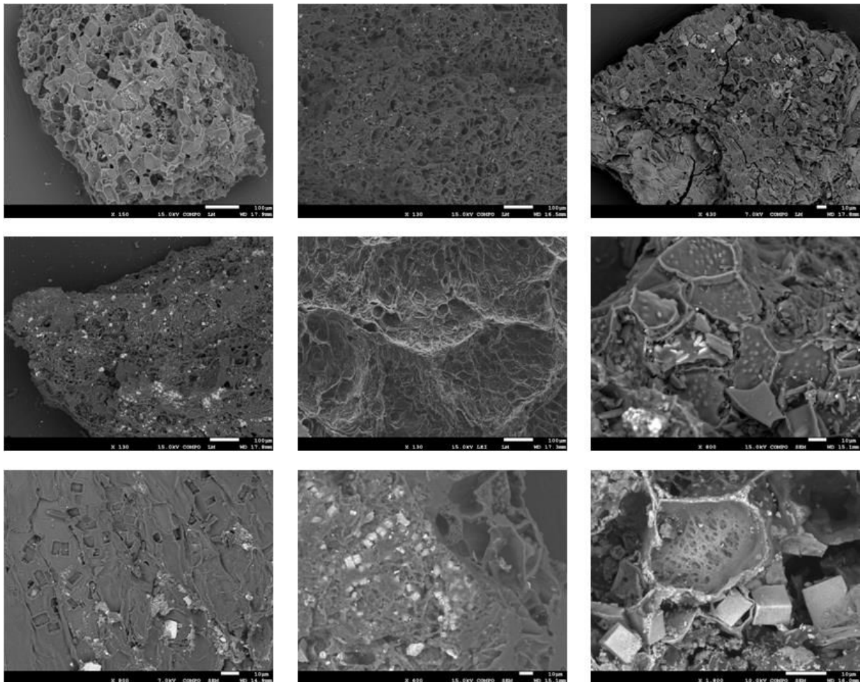
Figure 16 : Images au MEB de particules de biochar avec une structure cellulaire sans vaisseaux, avec présence de cristaux cubiques de calcite
