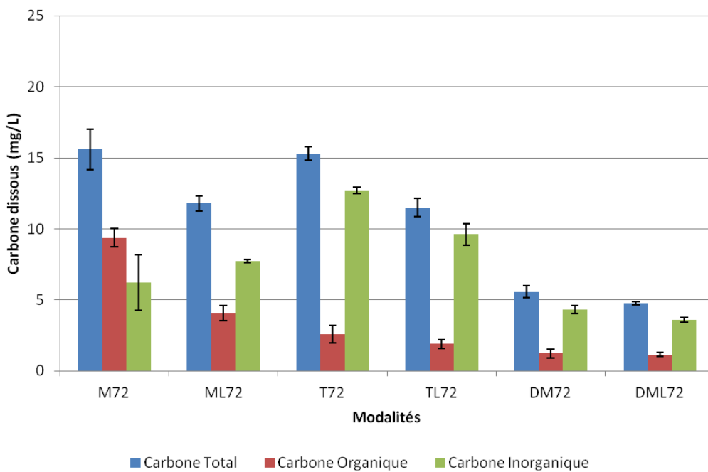
Figure 114 : Comparaison du paramètre "Lavage" sur le carbone dissous mesuré après sorption (M72 ou T72 : sans lavage, ML72 ou TL72 : avec lavage) et désorption (DM72 : sans lavage, DML72 : avec lavage)
