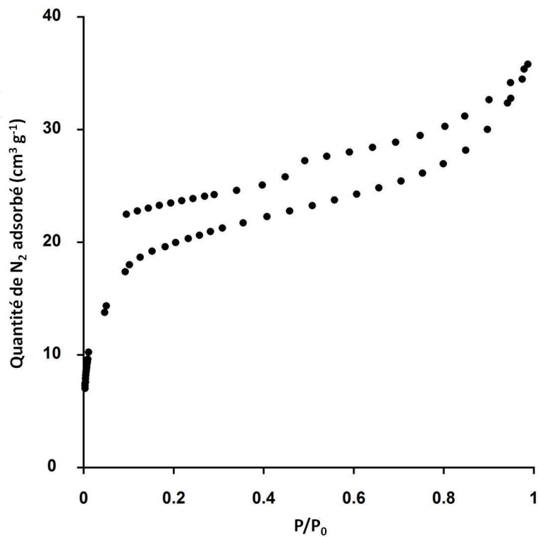
Figure 8 : Isothermes d'adsorption et de désorption de l'azote à 77 K sur les particules < 2 mm du biochar 1, après dégazage à 110°C. Les isothermes obtenues pour les autres fractions granulométriques du biochar ont une allure semblable à celle-ci.
