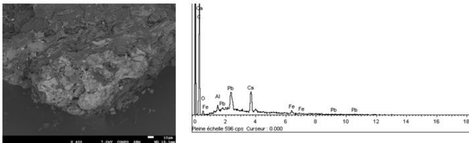
Figure 34 : Image au MEB d'une phase de carbonate de Pb et de Ca après sorption de Pb en solution monoélément sur une particule de biochar de bois feuillus
