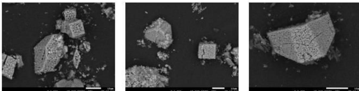
Figure 104 : Images au MEB de phases de calcite observées sur les cendres de bois avant pyrolyse et après pyrolyse (biochar 2)
