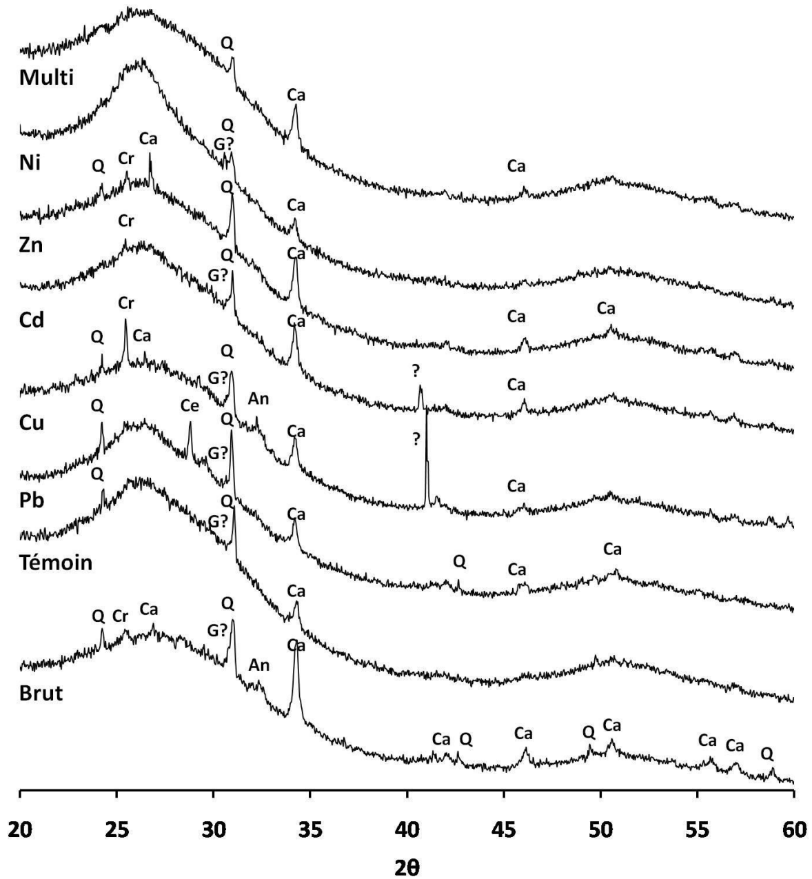
Figure 123 : Diagramme de DRX obtenu sur le biochar 1 réduit en poudre après sorption des métaux. Brut : non traité ; Témoin : récupéré après essais témoins sans métaux ; M = Pb, Cu, Cd, Zn, Ni : récupéré après essais de désorption en solution mono-élément avec une concentration initiale de 500 \mu\text{M} ; Multi : récupéré après essais de désorption en solution multiélément avec une concentration initiale de 100 \mu\text{M} pour chaque métal. Les pics ont été attribués aux cristaux suivants : calcite (Ca), quartz (Q), cristobalite (Cr), anorthoclase (An), graphite (G), céroussite (Ce). Un pic majeur dans l'échantillon Cu ( d = 2,55 ) n'a pas pu être identifié. Les traces de graphites ne peuvent pas être confirmées car elles interfèrent avec le pic de quartz.
