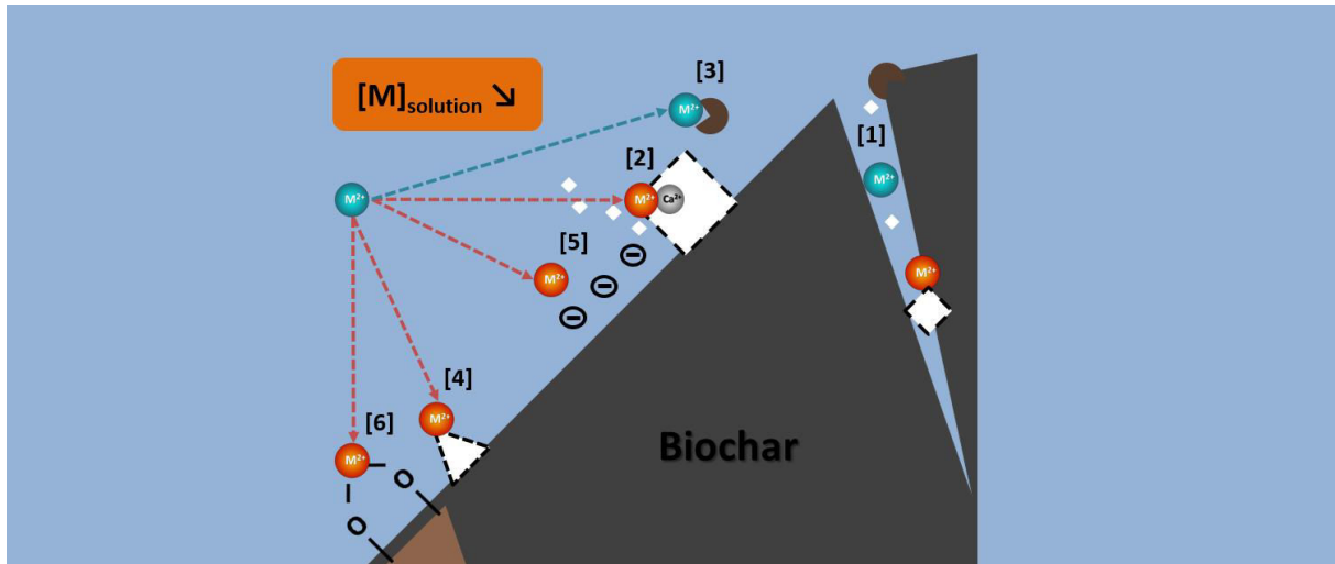
Figure 48 : Schéma mécanistique des interactions entre biochar et métaux en solution. Les métaux M sont soit en solution (en bleu) soit immobilisés à la surface du biochar (en orange).
