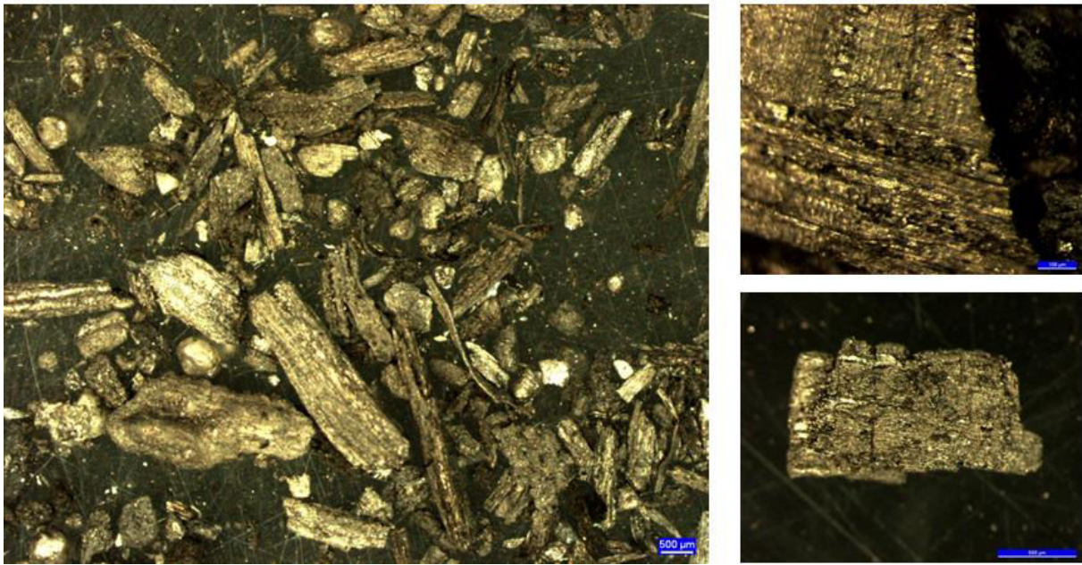
Figure 110 : Clichés de particules du biochar de bois 3 prises sous la loupe binoculaire, avec structure de vaisseaux ligneux reconnaissables
