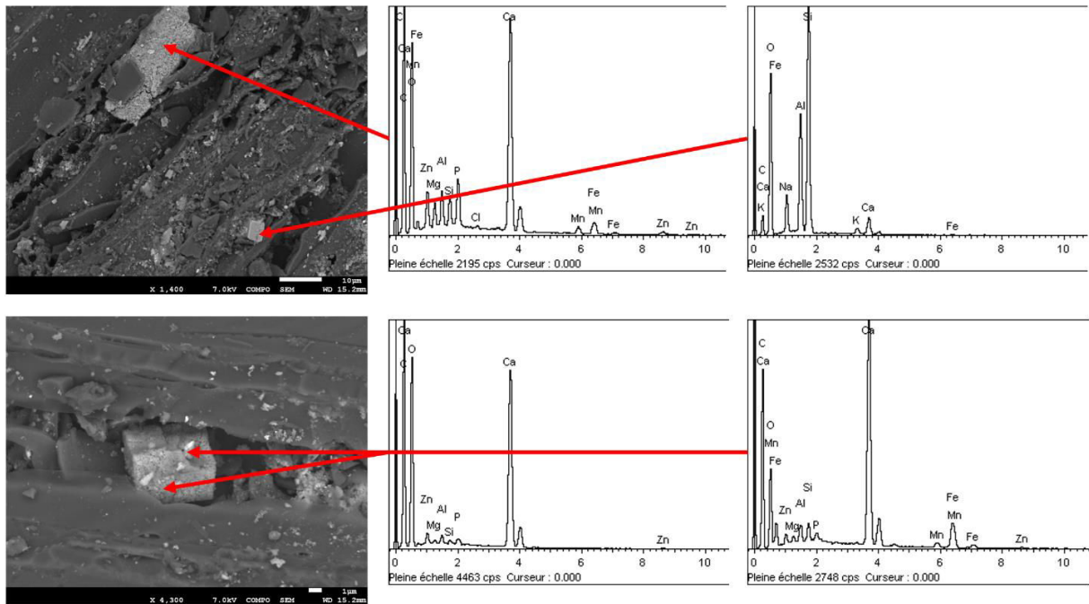
Figure 128 : Observations au MEB de particules de biochar récupéré en entrée de la colonne C2 associée à la colonne C1 contenant le sol A (essai N°1), avec cristaux de calcite contenant Zn, Mg, Al, Si et P et cristaux de Al/Si ou Fe ne contenant pas de Zn
