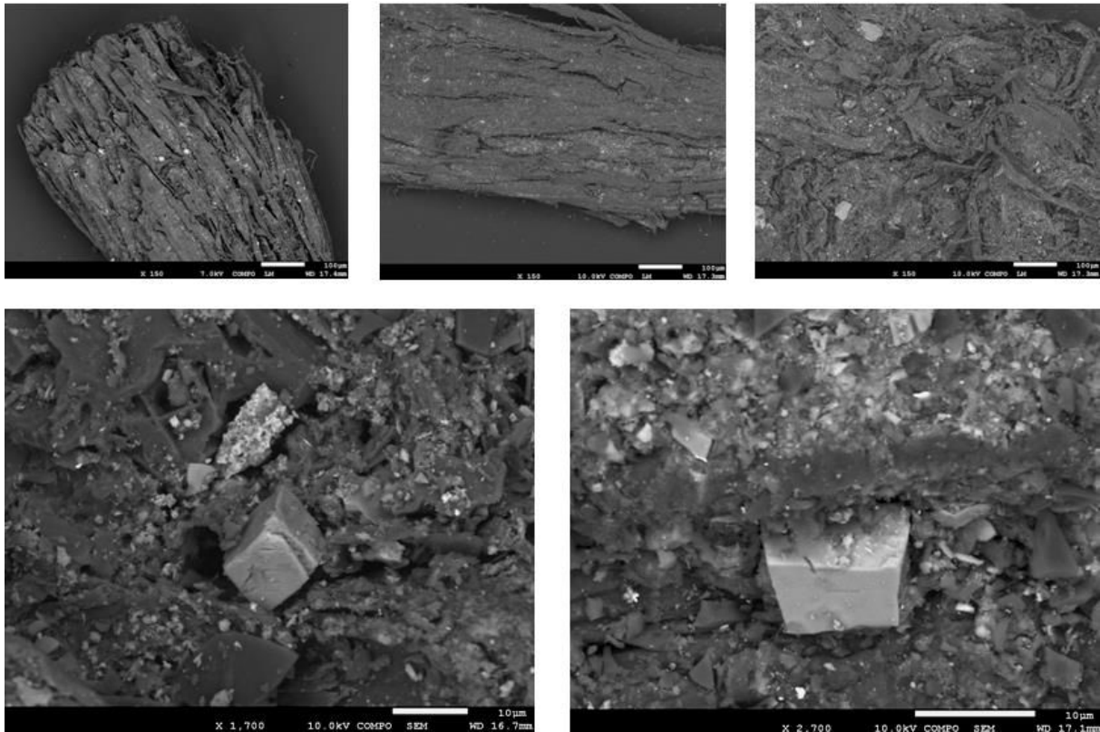
Figure 19 : Images au MEB de particules de bois peu ou pas pyrolysé avec vaisseaux ligneux apparents et différentes phases minérales en surface (calcite ou minéraux silicatés)
