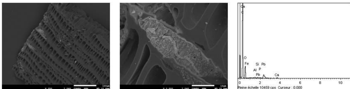
Figure 39 : Rayons ligneux avec formation d'un précipité de carbonate de Pb et de Ca sur une particule de biochar résineux récupéré après sorption d'une solution monoélément
