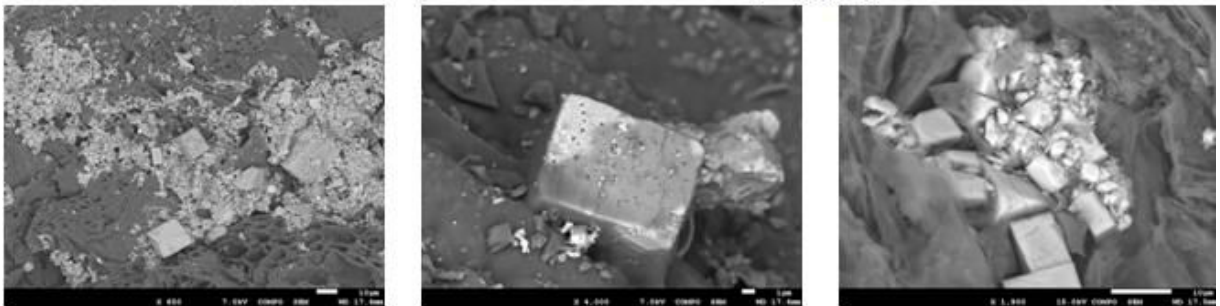
Figure 102 : Cristaux de calcite observés au MEB sur le bois avant pyrolyse et sur le biochar 2 résultant après pyrolyse
