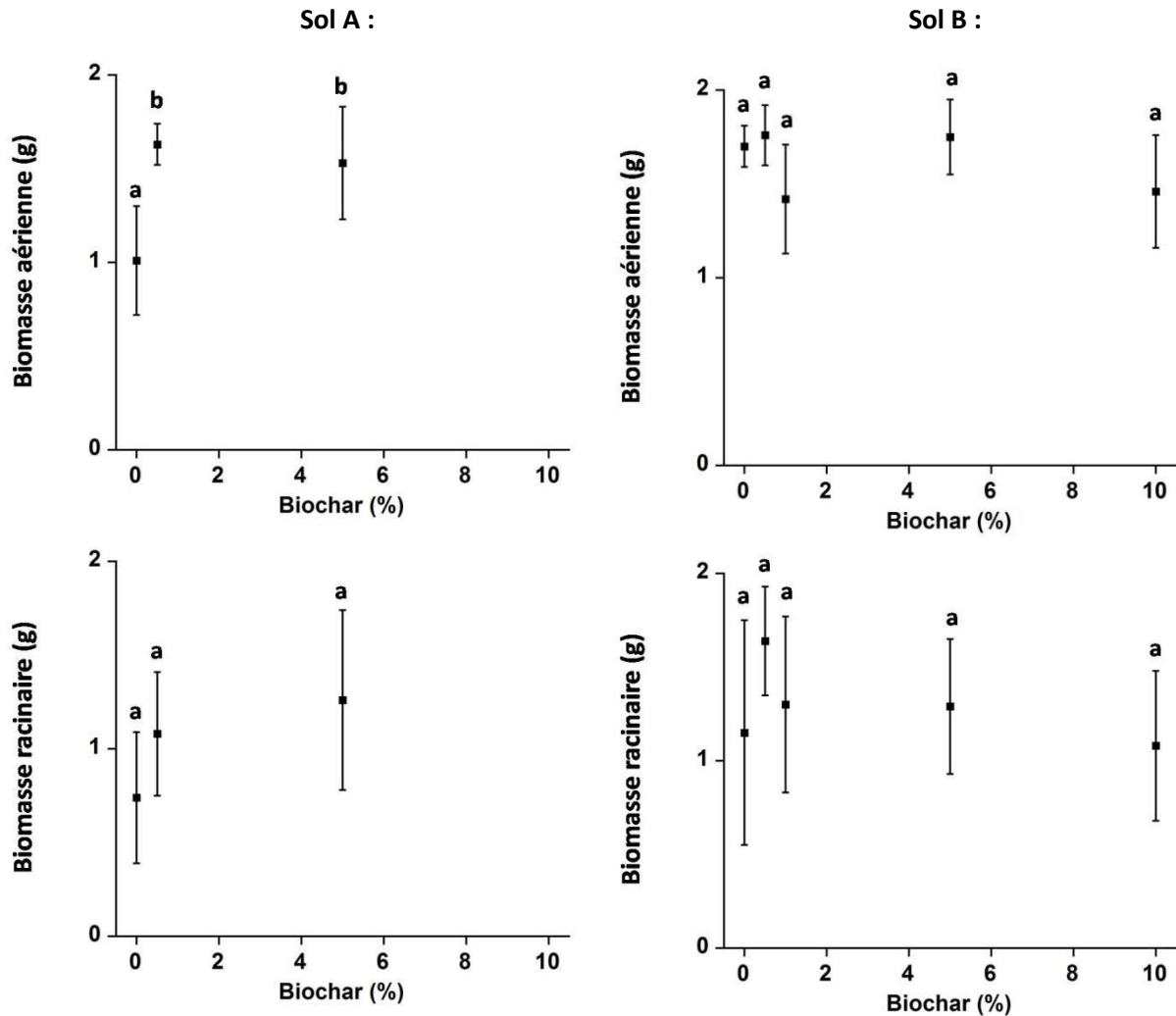
Figure 131 : Variation suivant la dose de biochar de la biomasse aérienne (en haut) et racinaire (en bas) de L. perenne produites à 12 semaines par pot, sur le sol A (à gauche) et B (à droite). Les barres d'erreurs correspondent à l'erreur standard. Différentes lettres indiquent des différences significatives (Student-Newman-Keuls, p < 0,05 ).
