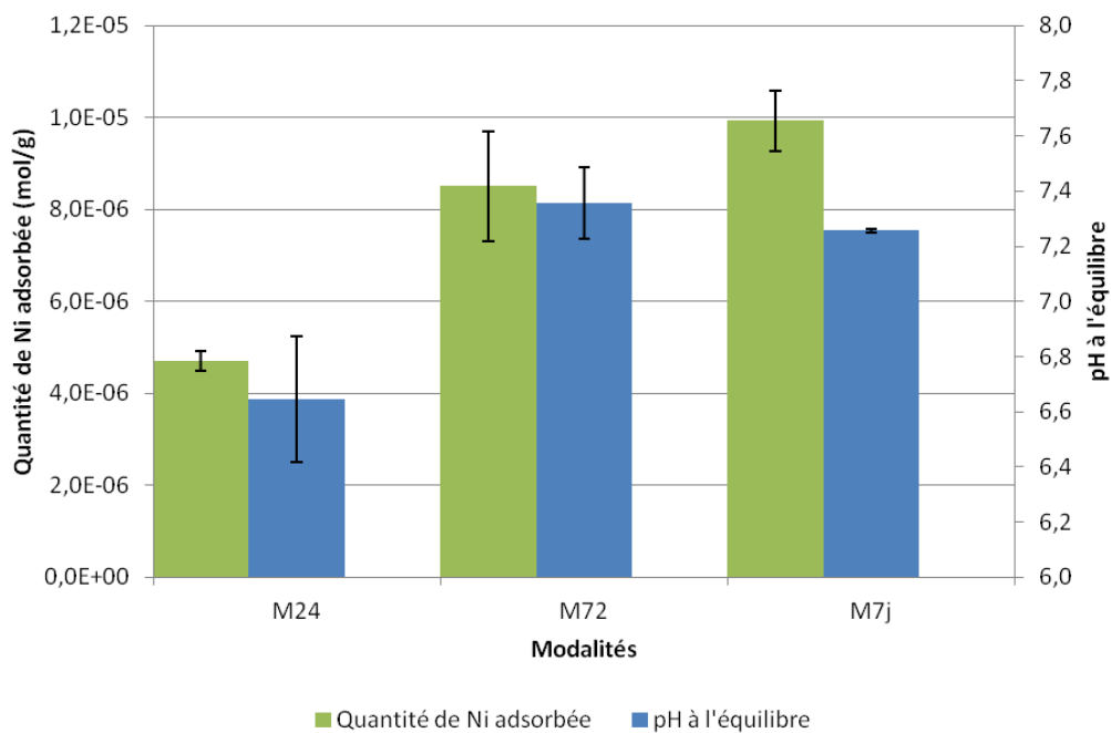
Figure 117 : Comparaison du paramètre "Durée de sorption" à 24h (M24), 72h (M72) et 7 jours (M7j) sur la quantité de Ni adsorbée et le pH de la suspension
