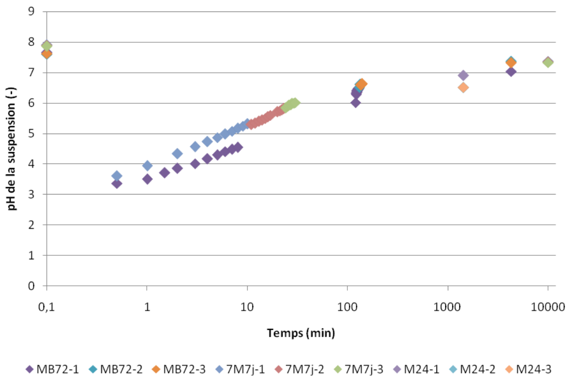
Figure 121 : Evolution du pH des suspensions de biochar suivant l'injection d'une solution acidifiée de Ni (échantillons MB72, 7M7j et M24, échelle logarithmique)
