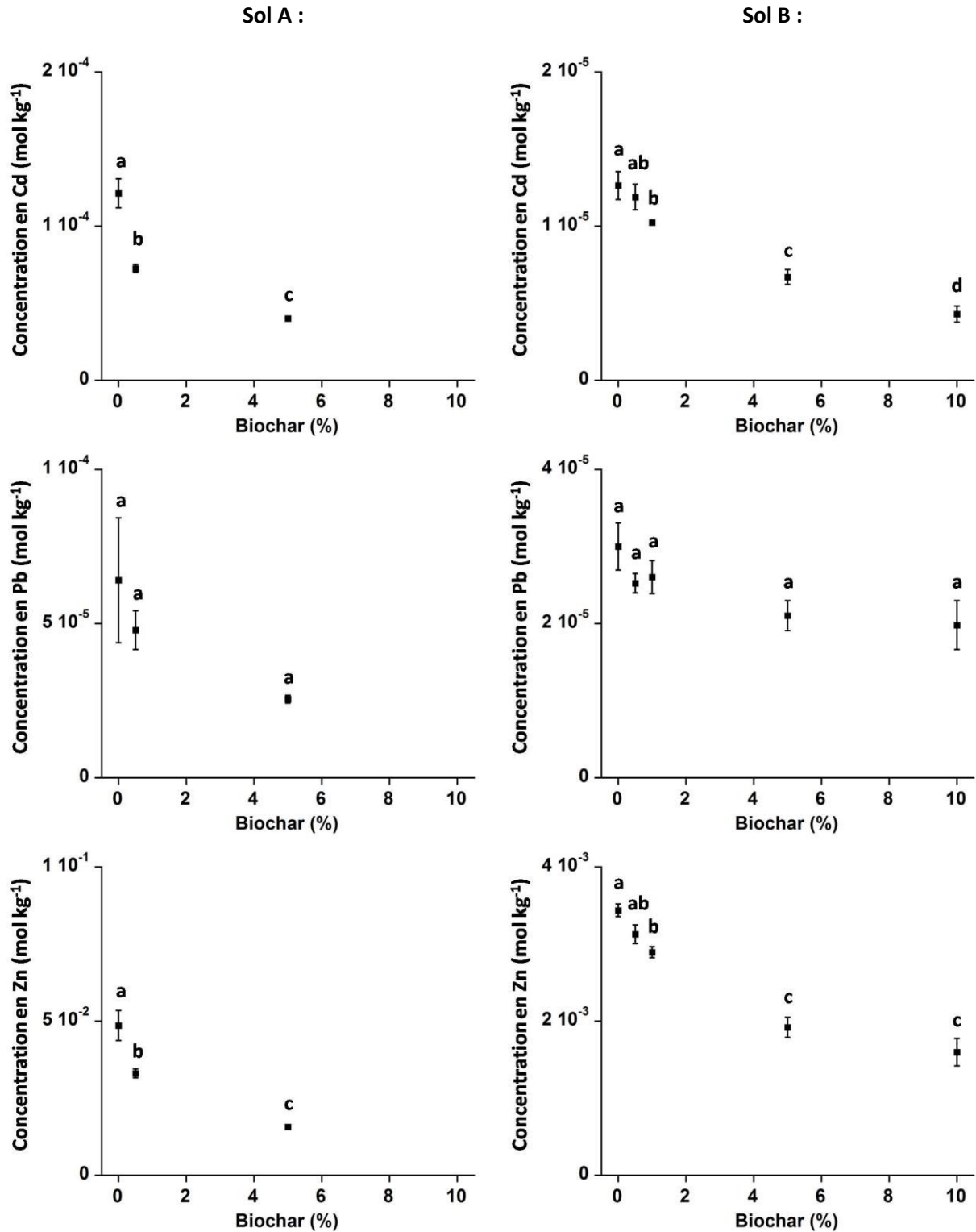
Figure 65 : Variation suivant la dose de biochar des concentrations de Cd (en haut), Pb (au milieu) et Zn (en bas) dans les parties aériennes de L. perenne produites à 6 semaines, sur le sol A (à gauche) et B (à droite). Les barres d'erreurs correspondent à l'erreur standard. Différentes lettres indiquent des différences significatives (Student-Newman-Keuls, p < 0,05 ).
