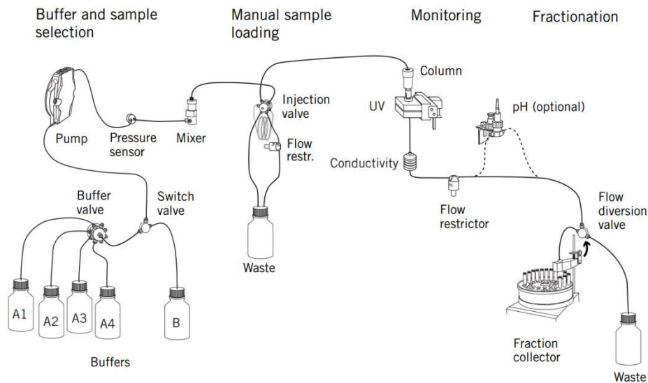
Figure 124 : Description du système Äkta Prime (documentation GE Healthcare)
