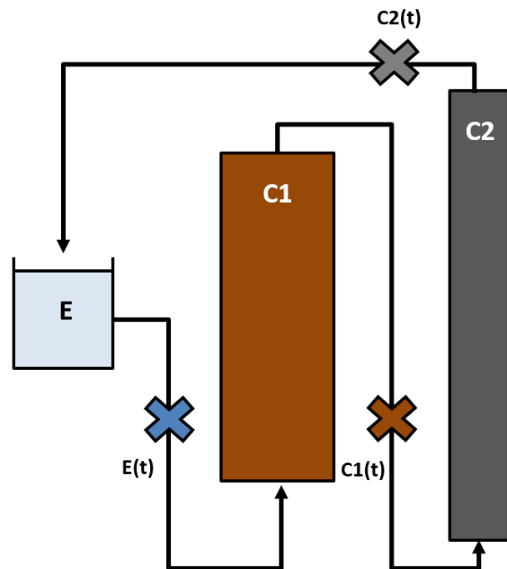
Figure 53 : Schéma simplifié des essais de lixiviation en boucle à deux colonnes
