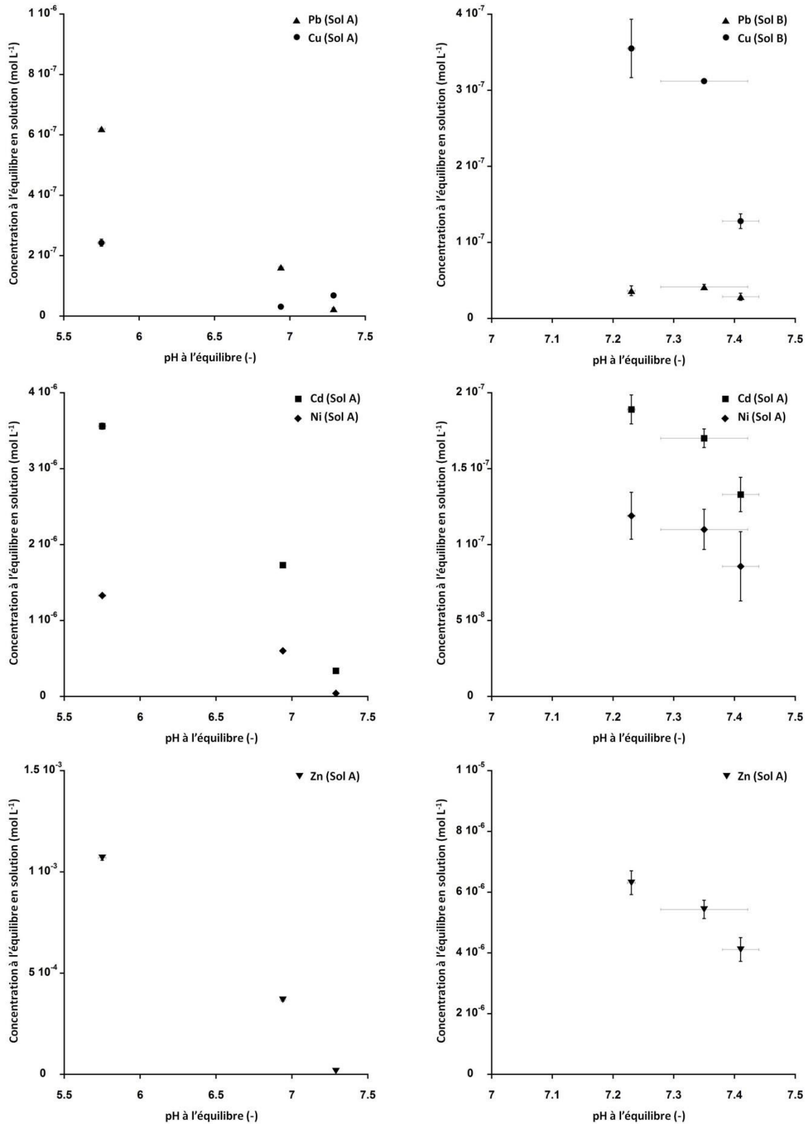
Figure 127 : Variation des concentrations de Pb et Cu (en haut), Cd et Ni (au milieu) et Zn (en bas) dans les suspensions à l'équilibre avec le pH, en mélangeant les modalités témoin, biochar et NaOH. Les barres d'erreur représentent l'erreur standard.
