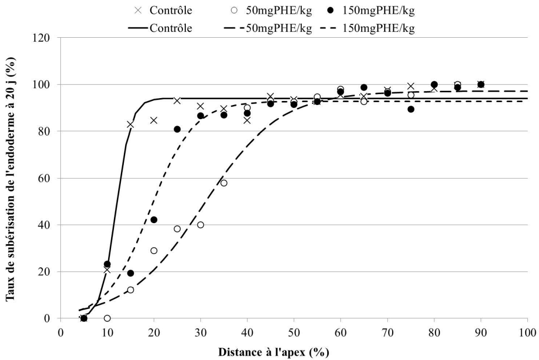
Figure 70 - Évolution du taux de subérisation de l'exoderme et l'endoderme de la racine principale selon les trois niveaux d'exposition en PHE à 20 j de culture (n = 5)
