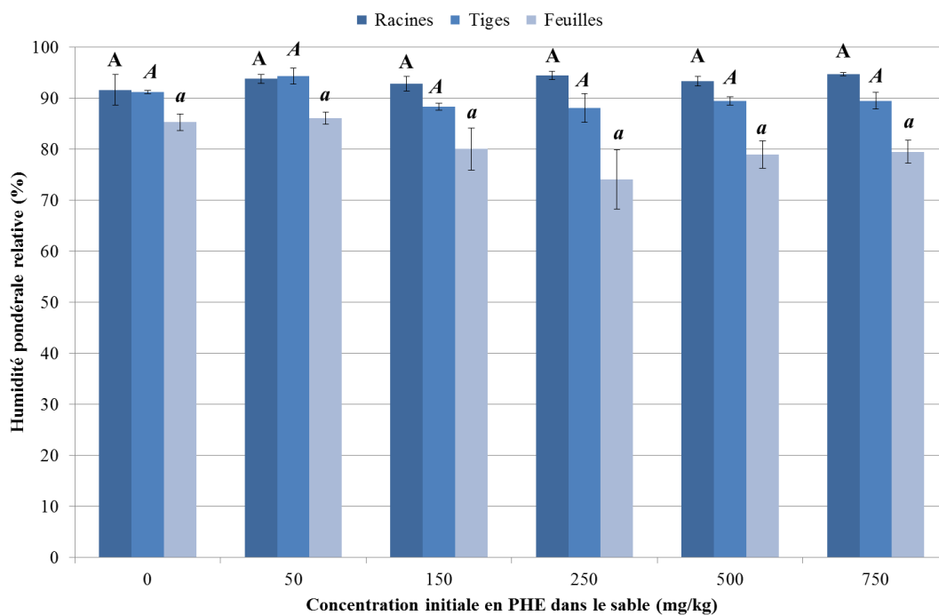
Figure 68 – Humidité pondérale relative des différents organes des maïs selon la concentration initiale en PHE dans le sable ( n = 6 )
