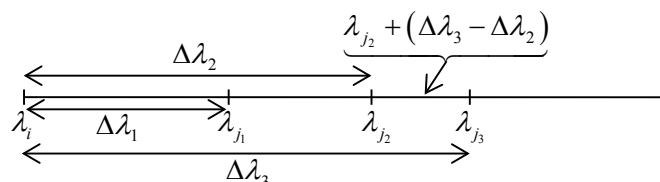
Figure 20.5 : Décalage itératif des longueurs d'onde
