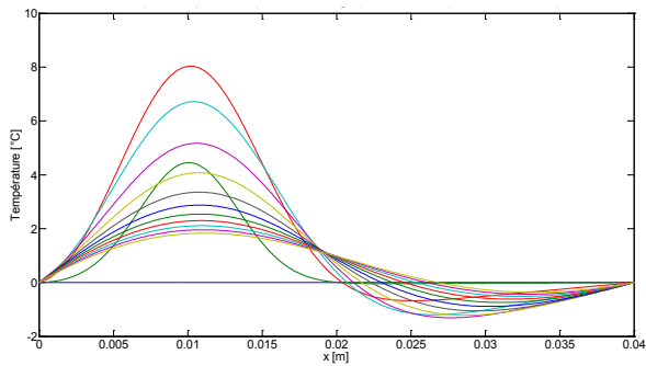
Figure 17.64 : Champ de température après correction affine (pour l'initialisation de la procédure d'estimation)
