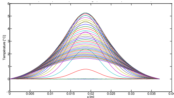
Figure 18.6 : Champ de températures expérimental après correction affine (pour l'initialisation de la procédure d'estimation)
