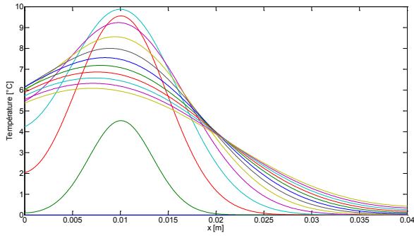
Figure 17.58 : Champ de température avant correction
