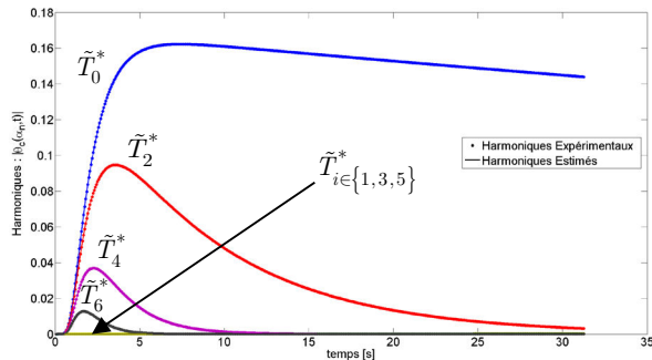
Figure 15.3 : Harmoniques simulés avec FlexPDE TM et estimés (Cos H/H)
