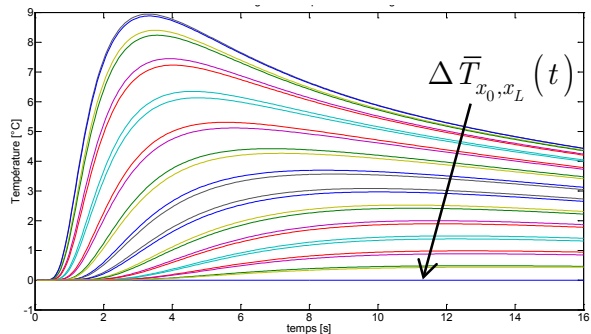
Figure 17.39 : Thermogrammes après correction (« Sin Imp »)
