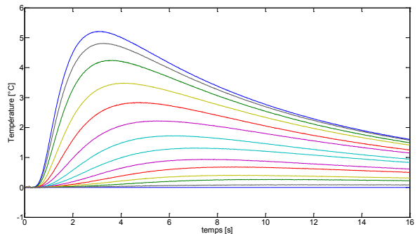
Figure 18.7 : Thermogrammes expérimentaux après correction affine (pour l'initialisation de la procédure d'estimation)
