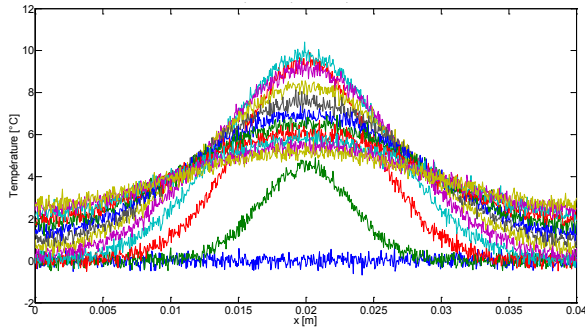
Figure 17.5 : Champ de température bruité
