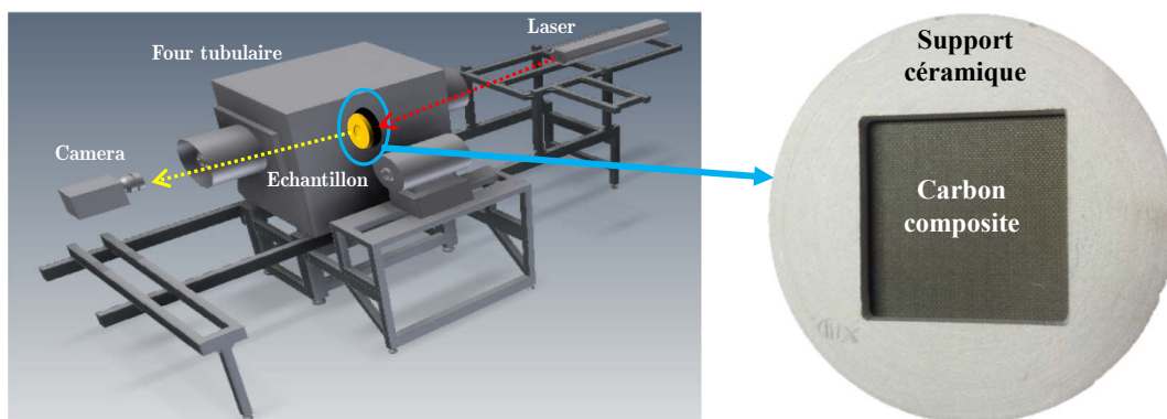
Figure 18.3 : Schéma du montage expérimental
