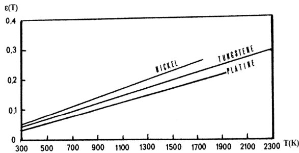
Figure 2.4 : Emissivité totale de métaux [13]
