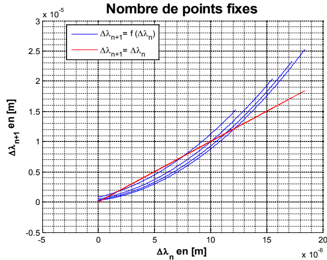
Figure 20.9 : Calcul successif des points fixes à partir de \lambda = 2 \mu\text{m} et T = 873\text{K}
