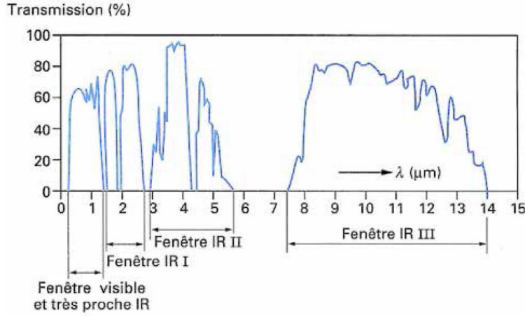
Figure 7.6 : Transmission spectral de l'atmosphère sur 2km au Sol [9]
