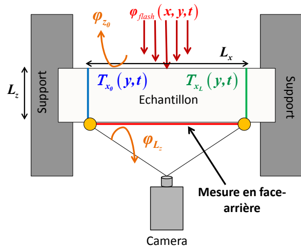
Figure 20.25 : Vue du dessus de l'échantillon et de son support
