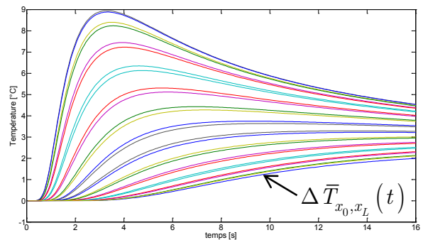
Figure 17.31 : Thermogrammes avant correction
