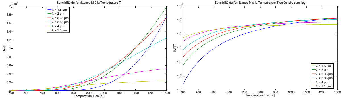
Figure 4.3 : Sensibilité de l'émissance à la température, en échelle linéaire à gauche et semi-log à droite.
