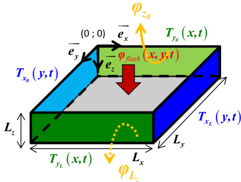
Figure 20.26 : Illustration schématique du problème 3D avant changement de variables
