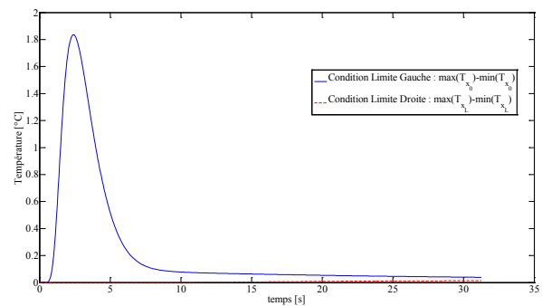
Figure 17.57 : Evolution temporelle de l'écart maximum de température suivant l'épaisseur ( Oz ) en x=0 et x=L_x (CLs)
