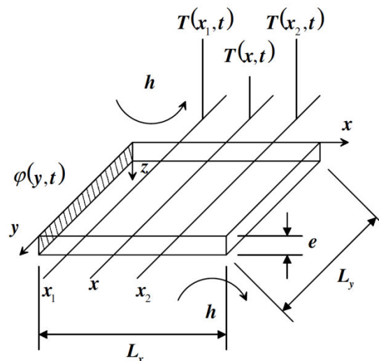
Figure 20.21 : Méthode de mesure basée sur le modèle de l'ailette, et proposée par Remy
