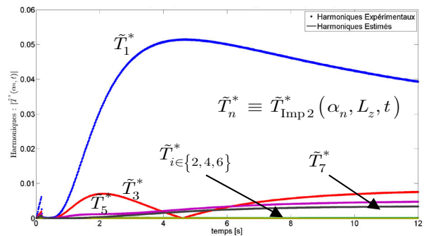
Figure 19.2 : Harmoniques expérimentaux et estimés de la méthode « Sin-Imp2 »
