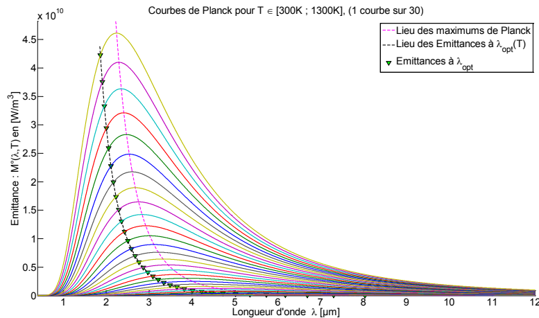
Figure 4.9 : Représentation graphique sur courbes de Planck des longueurs d'ondes optimales au sens de la minimisation de l'erreur relative sur la température en mono-spectrale.
