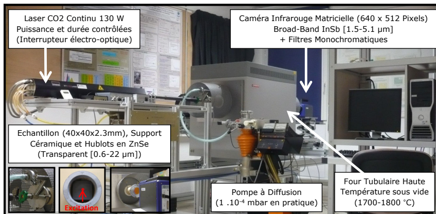
Figure 18.1 : Banc de mesures des diffusivités thermiques à haute température (extrait de [84])
