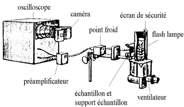
a. Montage original de la méthode flash de Parker [122]
