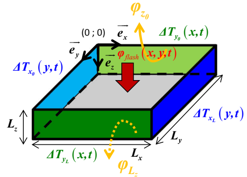
Figure 20.27 : Illustration schématique du problème 3D après changement de variables
