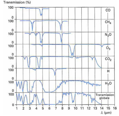
Figure 7.7 : Absorption moléculaire des constituants atmosphériques [9]
