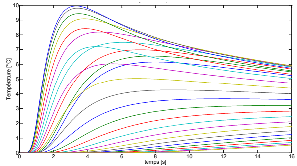
Figure 17.59 : Thermogrammes avant correction
