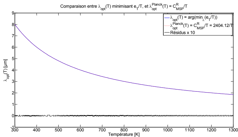
Figure 20.2 : Longueurs d'ondes optimales obtenues numériquement et par la loi \lambda_{opt}^{Planck} = C_{MSP}^R / T , pour T \in [300k;1300K] et \lambda \in [0,4\mu m;12\mu m] . Les résidus ont été multipliés par 100.
