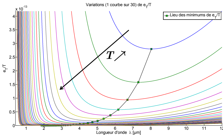
Figure 20.1 : Variations de \left[ 1 - \exp\left(-C_2/\lambda T\right) \right] \lambda / M_\lambda \propto \frac{e_T}{T} , pour T \in [300K; 1300K] et \lambda \in [0, 4\mu m; 12\mu m] . Pour des raisons de clarté, seule 1 courbe sur 30 est représentée.
