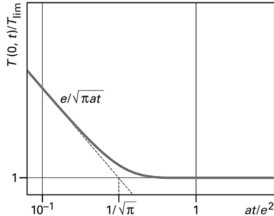
Figure 20.15 : Réponse (adimensionnée) au flash en face avant en échelles logarithmiques, et définition du temps de rupture de pente [120].
