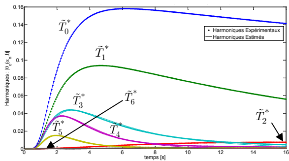
Figure 17.70 : Harmoniques expérimentaux (simulés) et estimés (Cos H/H)
