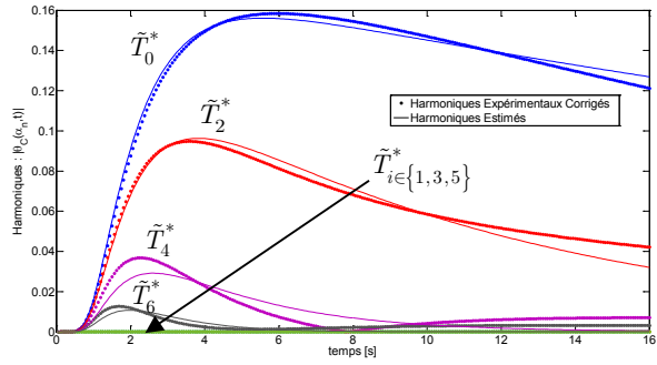
Figure 17.23 : Harmoniques expérimentaux et estimés (Cos AH)
