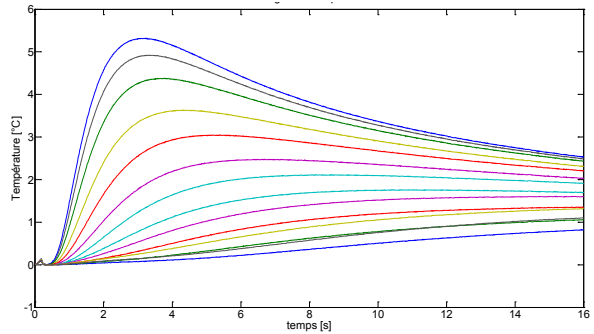
Figure 18.5 : Thermogrammes expérimentaux (avant correction)
