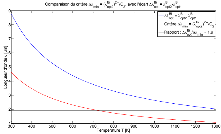
Figure 5.9 : Comparaison des écarts imposés par le critère \Delta\lambda_{\min} = \left(\lambda_{opt2}^{bi-Planck}\right)^2 T / C_2 , et ceux correspondant à la différence \Delta\lambda_{opt}^{bi-Planck} = \lambda_{opt2}^{bi-Planck} - \lambda_{opt1}^{bi-Planck} .
