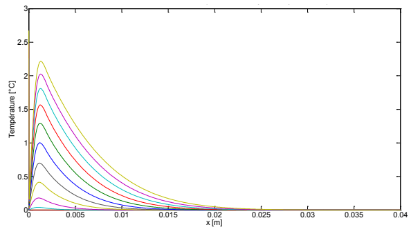
Figure 17.8 : Fonctions de correction gauche de « Sin Imp »
