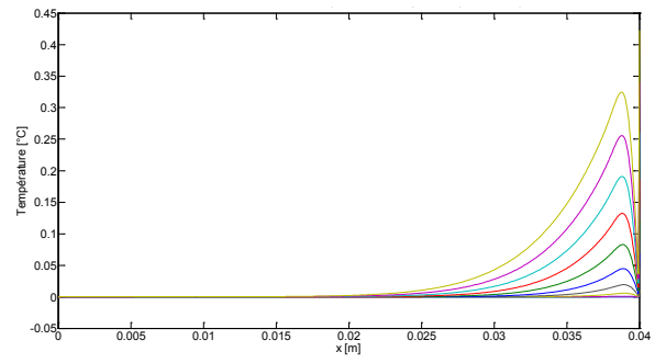
Figure 17.63 : Fonctions de correction droite « Sin Imp »
