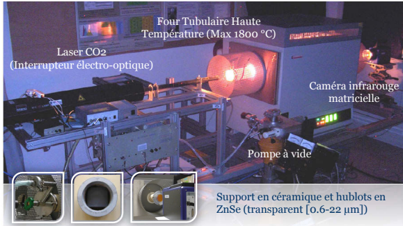
Figure 20.22 : Banc expérimental de caractérisation à haute température
