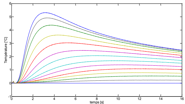
Figure 18.11 : Thermogrammes expérimentaux après correction (« Sin Imp »)
