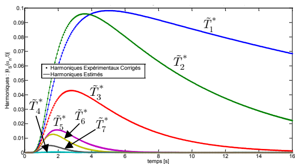
Figure 17.72 : Harmoniques expérimentaux (simulés) corrigés (SP1) et estimés (Sin Ind)
