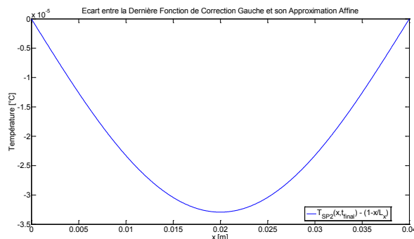
Figure 13.5 : Ecart entre la fonction de correction gauche à t=50s et son approximation affine
