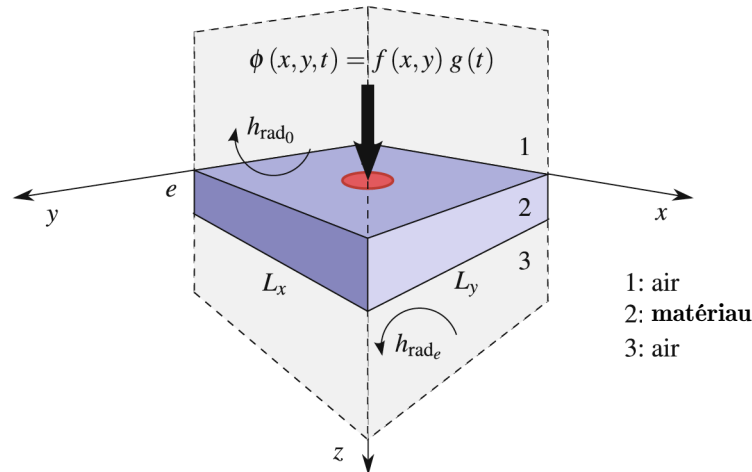
Figure 9.10 : Modélisation de Souhar du couplage conductif entre l'échantillon et l'air avoisinant par modèle multicouches. (Extrait de [183]).
