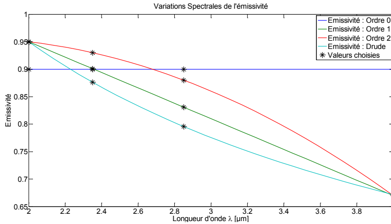
Figure 6.10 : Variations spectrales de l'émissivité utilisées pour la validation numérique
