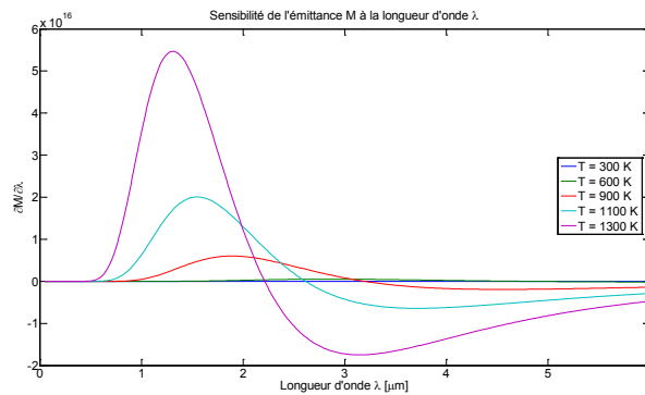
Figure 4.5 : Sensibilité de l'émittance à la longueur d'onde.
