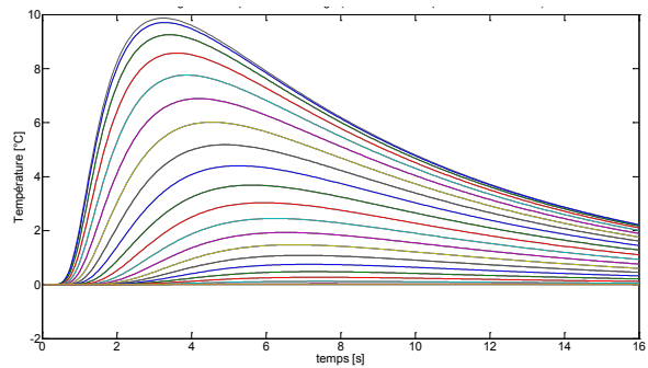
Figure 17.10 : Thermogrammes après correction affine (pour l'initialisation de la procédure d'estimation)
