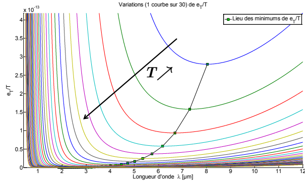
Figure 4.7 : [1 - \exp(-C_2/\lambda T)] \lambda / M_\lambda \propto \frac{e_T}{T} , pour T \in [300K ; 1300K] et \lambda \in [0, 4\mu m ; 12\mu m] .
