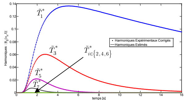
Figure 15.4 : Harmoniques simulés avec FlexPDE TM corrigés (SP1) et estimés (Sin Ind)
