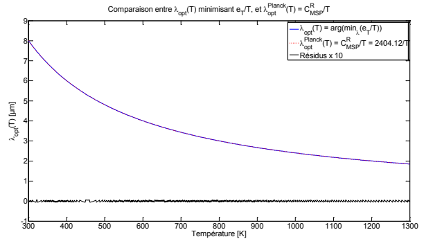
Figure 4.8 : Longueurs d'ondes optimales obtenues numériquement et par la loi \lambda_{opt}^{Planck} = C_{MSP}^R / T , pour T \in [300K ; 1300K] et \lambda \in [0, 4\mu m ; 12\mu m] . Les résidus ont été multipliés par 100.
