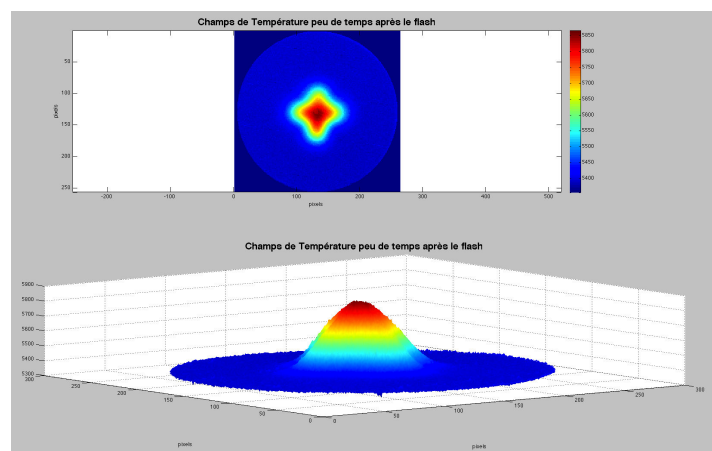
Figure 7.24 : Champ de températures après traitement (20ième image après excitation)
