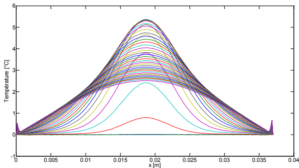
Figure 18.10 : Champ de températures expérimental après correction (« Sin Imp »)
