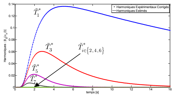
Figure 17.25 : Harmoniques expérimentaux et estimés (Sin Imp)
