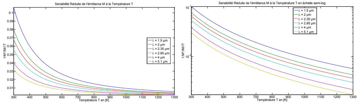
Figure 4.2 : Sensibilité Réduite de l'émittance à la température, en échelle linéaire à gauche et semi-log à droite.
