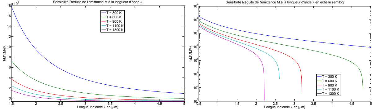
Figure 4.4 : Sensibilité Réduite de l'émission à la longueur d'onde, en échelle linéaire à gauche et semi-log à droite.
