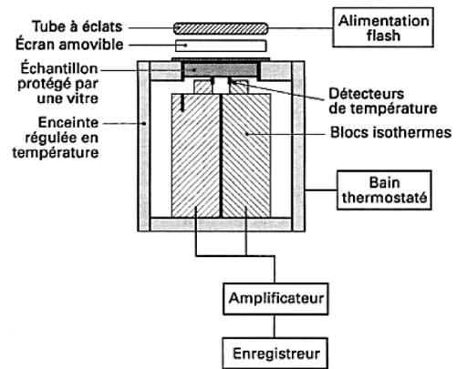
b. Exemple de montage expérimental proposé par Degiovanni [111]
