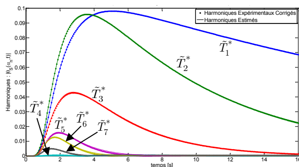
Figure 17.73 : Harmoniques expérimentaux (simulés) corrigés (SP1) et estimés (Sin Imp)
