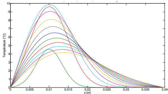
Figure 17.66 : Champ de températures après correction (« Sin Ind »)
