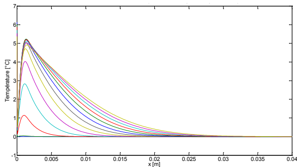
Figure 17.62 : Fonctions de correction gauche « Sin Imp »
