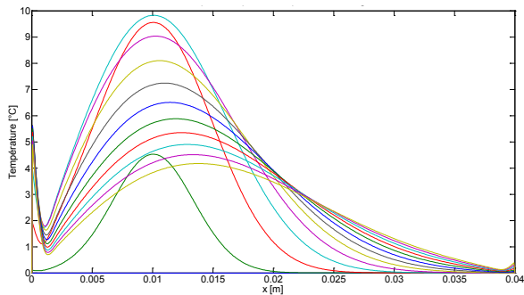
Figure 17.68 : Champ de températures après correction (« Sin Imp »)
