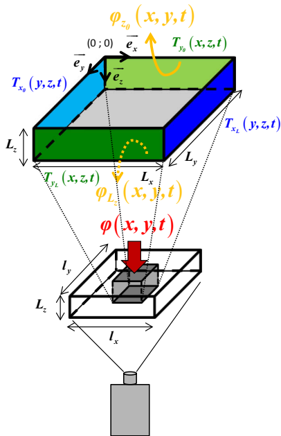
Figure 20.24 : Vue schématique 3D de l'échantillon et de la zone d'étude
