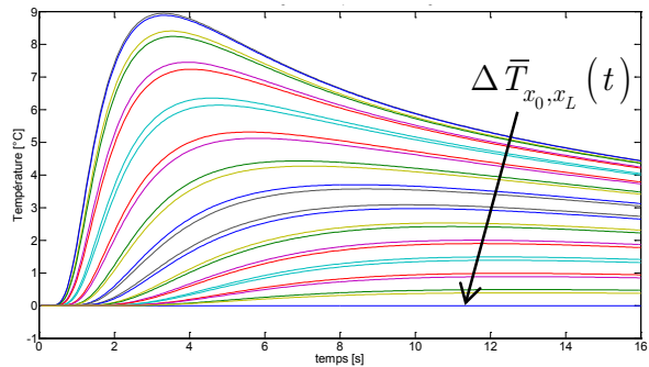
Figure 17.37 : Thermogrammes après correction (« Sin Ind »)
