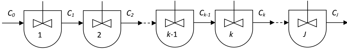
Figure 5.5. Schéma d'une cascade de mélangeurs.
