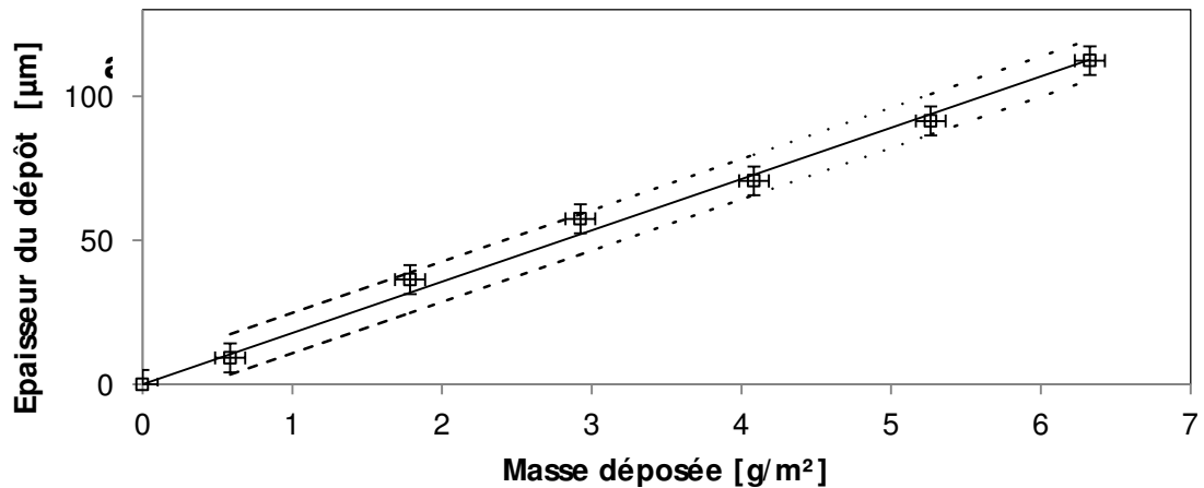
Figure 74 : Épaisseur du dépôt de particules de carbone en fonction de la masse déposée, mesurée par MEGAPAN à une vitesse de 0,8 cm/s
