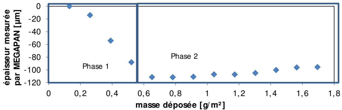
Figure 134 : Valeur d'épaisseur mesurée par MEGAPAN pour un aérosol d'oxyde de titane à un débit de 1,2 cm/s
