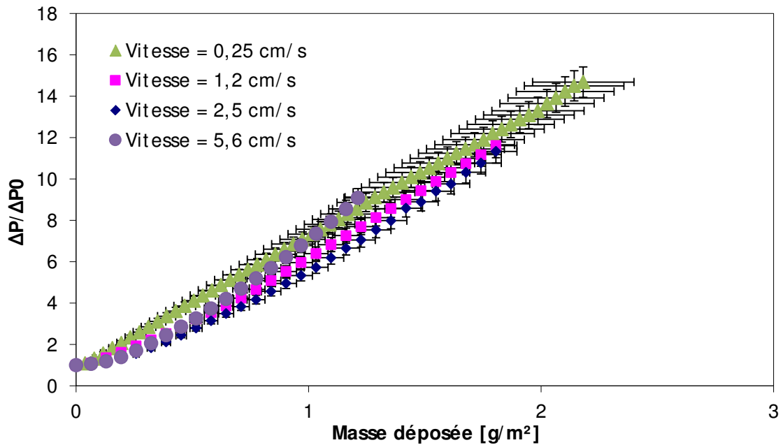
Figure 98 : Evolution de la résistance aéroulique en fonction de la masse déposée pour un pli colmaté avec des aérouls de carbone à différentes vitesses
