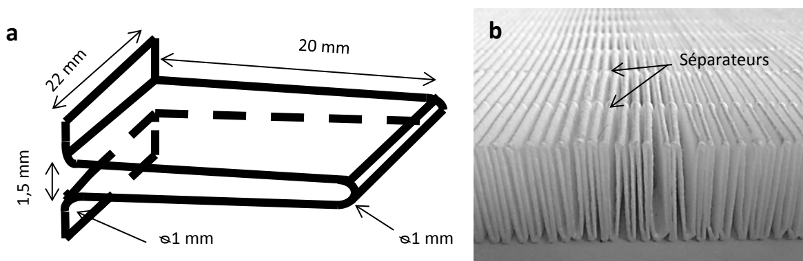
Figure 88 : (a) Géométrie du pli contenu dans le banc (b) photographie d'une nappe de medium plissé
