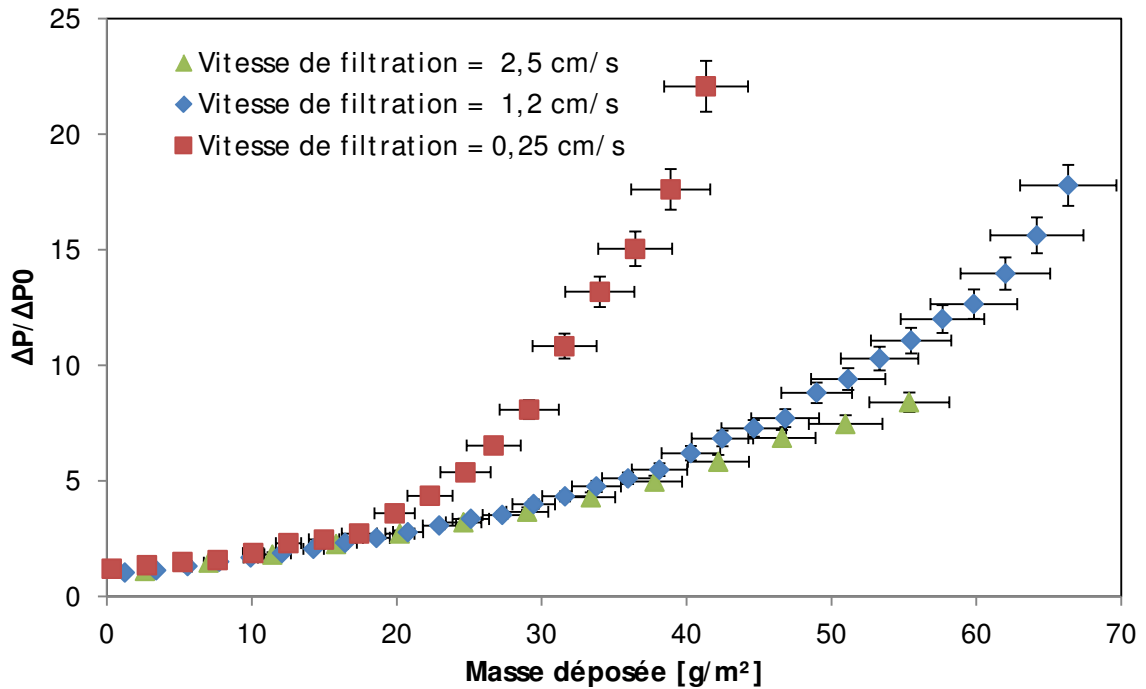
Figure 99 : Courbe d'évolution de la résistance aéroulrique en fonction de la masse d'alumine déposée pour différentes vitesses de filtrations
