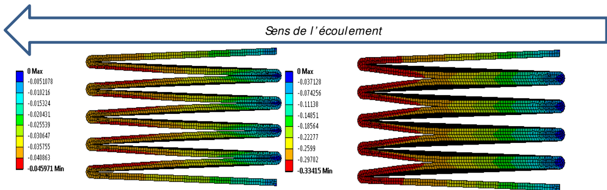
Figure 96 : Illustration de la déformation la vitesse nominale 2,5 cm/s - 250 Pa (gauche) et à 8 cm/s - 2000 Pa (droite)
