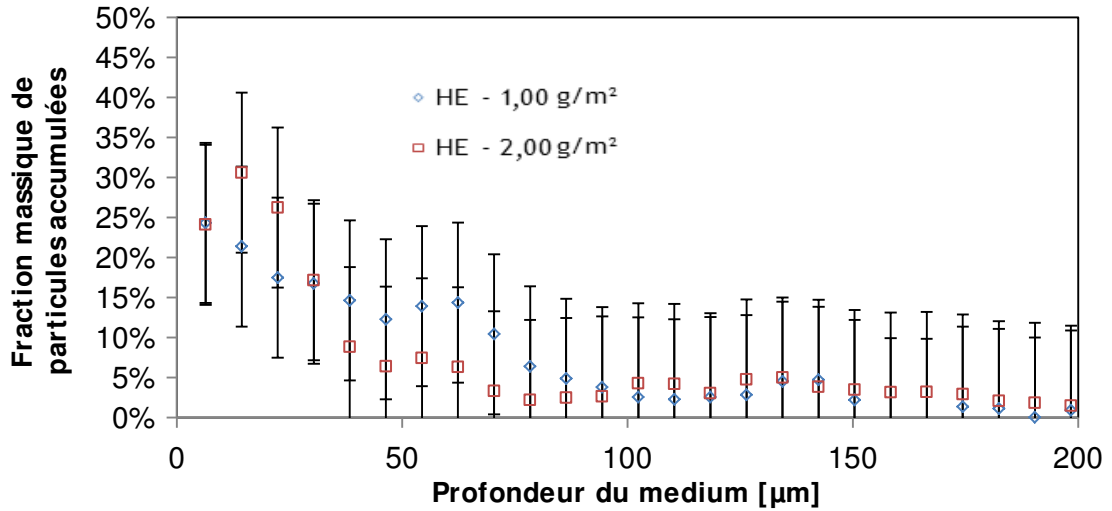
Figure 64 : Répartition des aérosols dans la profondeur du medium HE pour des aérosols d'argent
