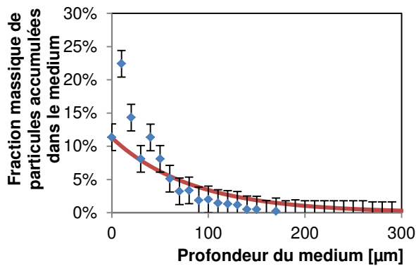
Figure 73 : Comparaison entre les valeurs expérimentales et les valeurs obtenues en appliquant des modèles d'efficacité sur des tranches de médium de 10 µm d'épaisseur avec les paramètres regroupés à droite. (a) particules d'argent (b) particules d'oxyde de titane et (c) alumine
