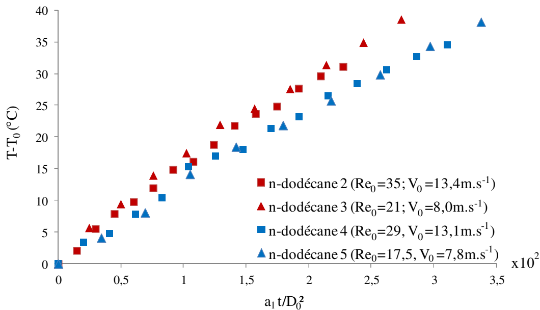
Figure 4.3 : Influence de la vitesse des gouttes sur leur échauffement. Cas de gouttes de n-dodécane ( D_0=155\mu m C_0=4,3 en rouge et C_0=3,2 , D_0=134\mu m en bleu).
