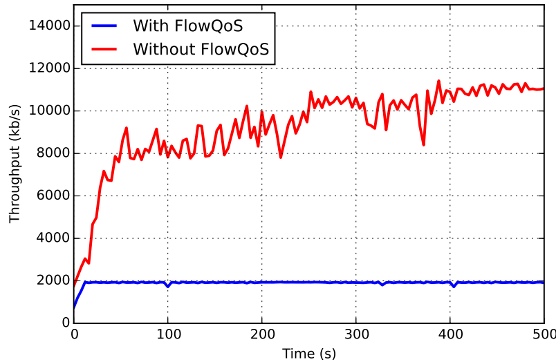
FIGURE 3.11 – L'évolution au cours du temps du débit de téléchargement des flux en concurrence pour la bande passante disponible avec et sans FlowQoS
