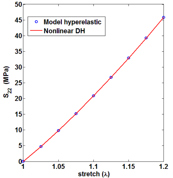
Fig. 8. 16. Evolution des composantes normales S_{11} et S_{22} du second tenseur de Piola-Kirchhoff en fonction des dilatations principales par l'homogénéisation et le modèle hyperélastique
