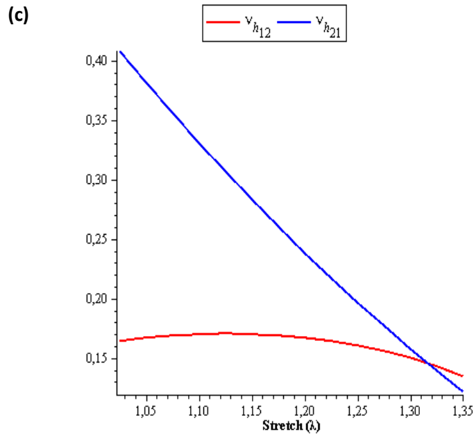
Figure 8.4: propriétés effectives simulées. (a) Modules de traction E_{h_{11}}, E_{h_{22}} (b) Taux d'ondulation \%C_{r_{11}}, \%C_{r_{22}} . (c) Coefficients de contraction v_{h_{12}}, v_{h_{21}} en fonction de la dilatation dans la direction x .
