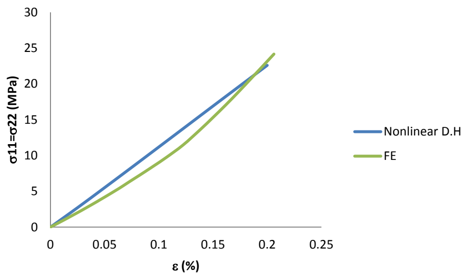
Fig. 8.13 Comparaison de la réponse équi-biaxiale en traction selon x pour le tissage d'armure toile équilibré obtenue par homogénéisation et par EF (ABAQUS).
