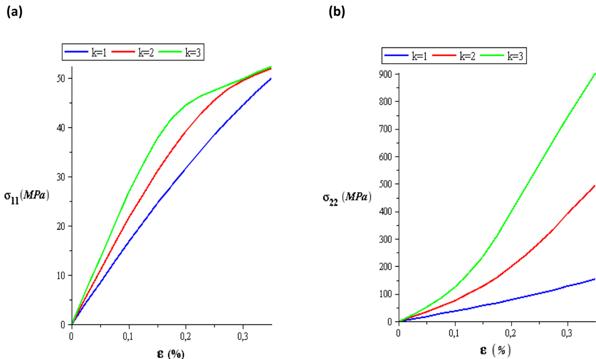
Fig. 8.7 Contrainte de Cauchy (a) direction x et (b) direction y en fonction de la déformation pour un tissage déséquilibré pour différentes valeurs du rapport de biaxialité.
