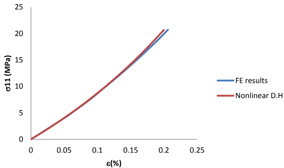
Fig. 8.12. Comparaison de la réponse uniaxiale en traction selon x pour le tissage d'armure toile équilibré obtenue par homogénéisation et par EF (ABAQUS).
