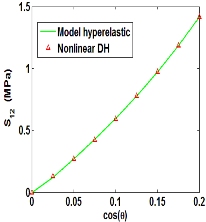
Fig. 8.17. Evolution de la composante de cisaillement du second tenseur de Piola-Kirchhoff S_{12} par l'homogénéisation et le modèle hyperélastique
