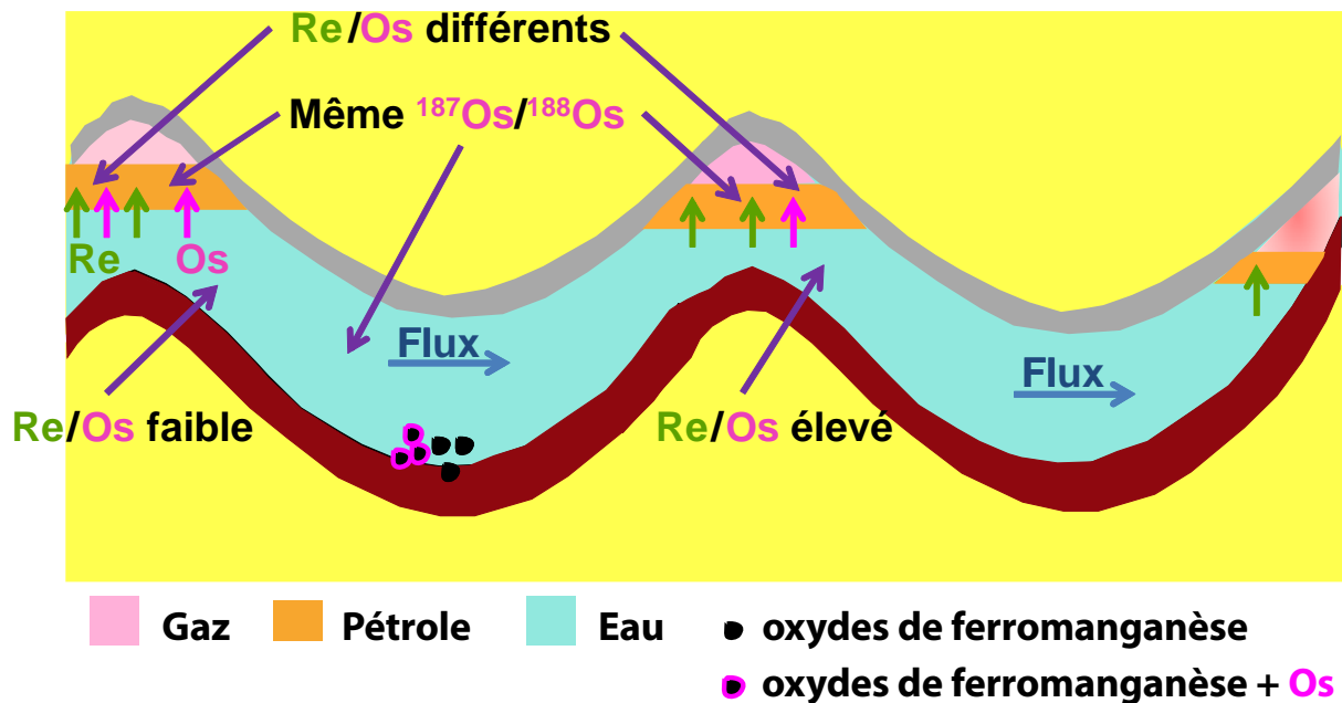
Figure 67. Réinitialisation isotopique – Les rapports isotopiques d'Os sont identiques, tandis que les rapports Re/Os sont différents selon la localité de l'aquifère (exemple de l'influence des oxydes de Fe-Mn). Les différents pièges pétroliers auront ainsi des rapports ^{187}\text{Os}/^{188}\text{Os} identiques mais des rapports Re/Os différents.
