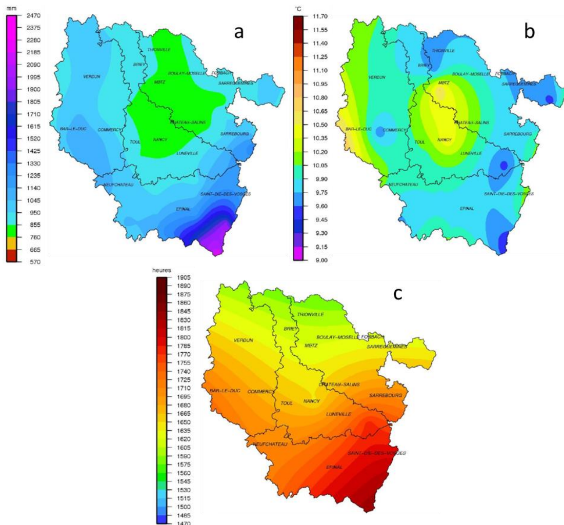
Figure I-5 : Cartographie des normales climatologiques. a) Cumul des précipitations quotidiennes (en mm, 1981-2010), b) Moyenne des températures moyennes quotidiennes (en °C, 1981-2010) et c) Cumul des insulations quotidiennes (en heures, 2001-2010). (Source : Météo France).
