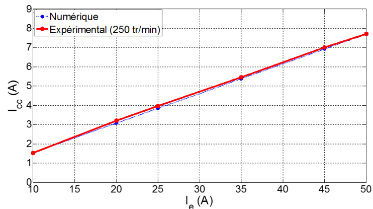
Figure 5-27 Essai en court-circuit à 250 tr/min.
