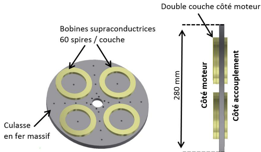
Figure 5-2 Inducteur supraconducteur.
