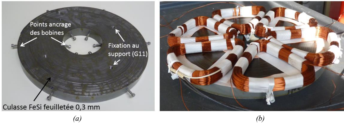
Figure 5-14 Stator avant imprégnation (a) culasse magnétique (b) ancrage des bobines sur la culasse.
