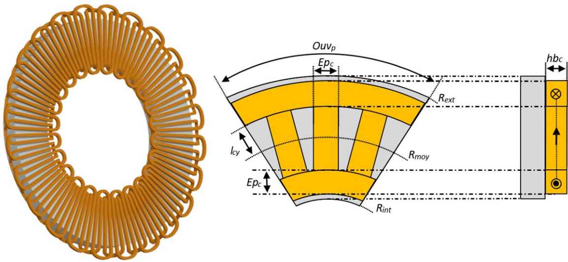
Figure 2-2 Paramètres du stator en cuivre sous un pôle.
