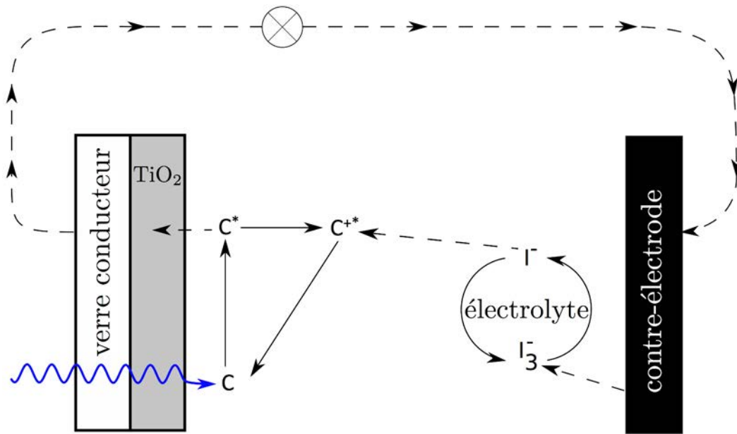
FIGURE I.3.2 – Schéma général de fonctionnement d'une cellule solaire de troisième génération.
