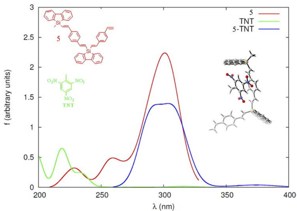
FIGURE IV.3.7 – Spectre d'absorption théorique de 5 , du trinitrotoluène (TNT) et de leur complexe.
