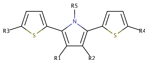
FIGURE IV.2.1 – Structure du donneur dithiényle-pyrrole.
