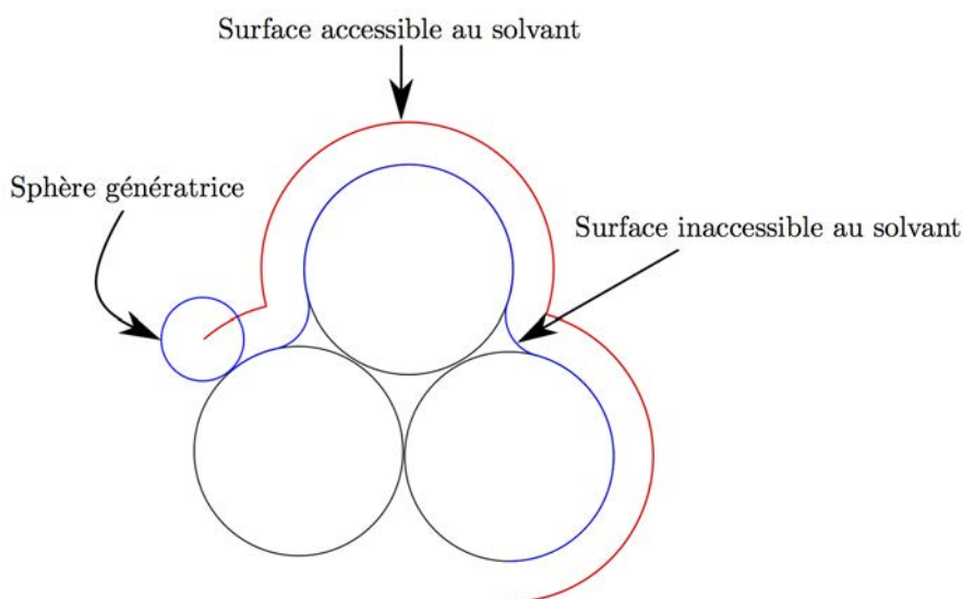
FIGURE II.5.3 – Détail des différentes surfaces et de la sphère génératrice dans le modèle PCM.
