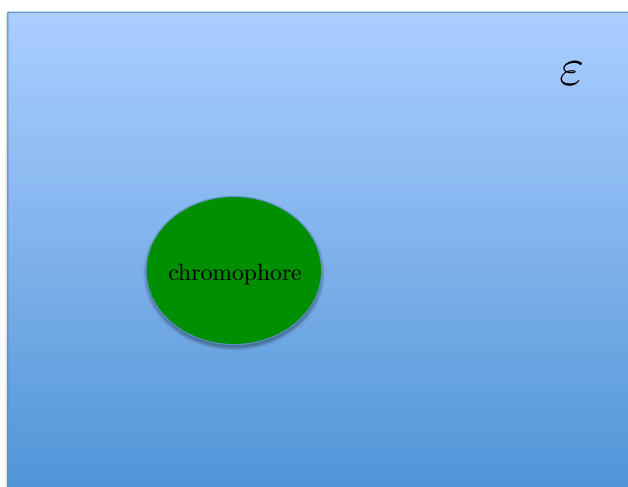
FIGURE I.5.4 – Schématisation grossière du modèle PCM.
