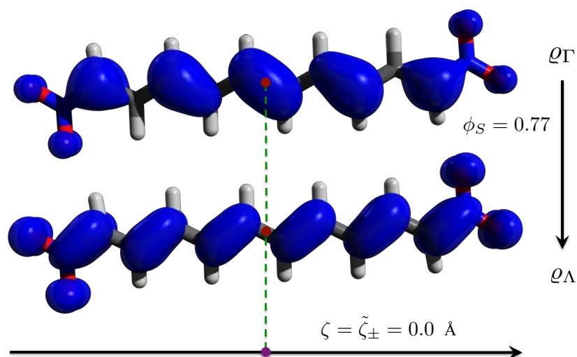
FIGURE IV.1.6 – Illustration de la nullité de la distance de transfert de charge pour une molécule linéaire symétrique.
