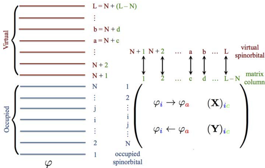
FIGURE III.1.1 – Déplacement d’indices entre orbitales et éléments matriciels.
