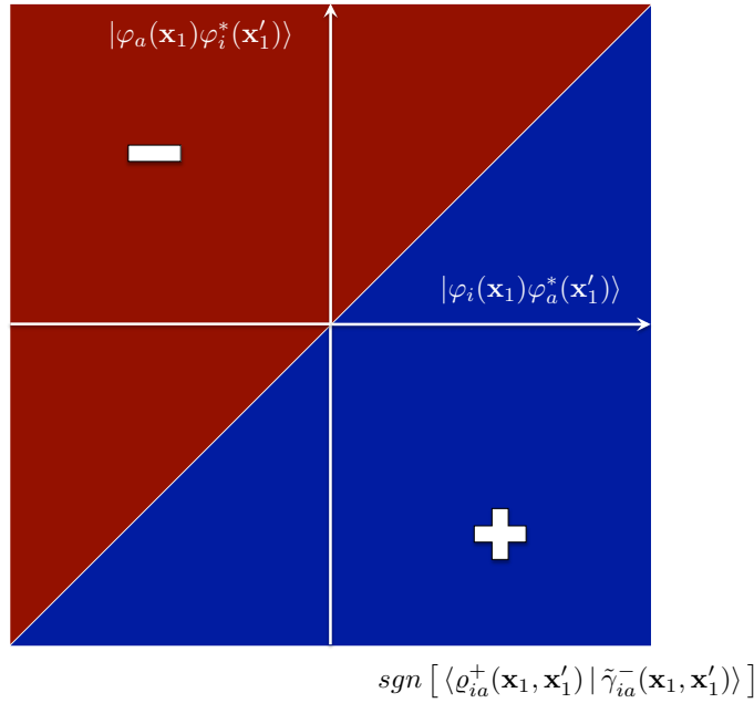
FIGURE III.1.5 – Orientation relative du tenseur canonique de transition élémentaire par rapport aux tenseurs unité de H .
