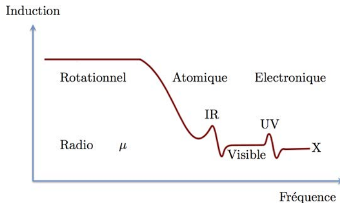
FIGURE II.5.2 – Evolution de la polarisation en fonction de la fréquence d'oscillation du champ électrique.
