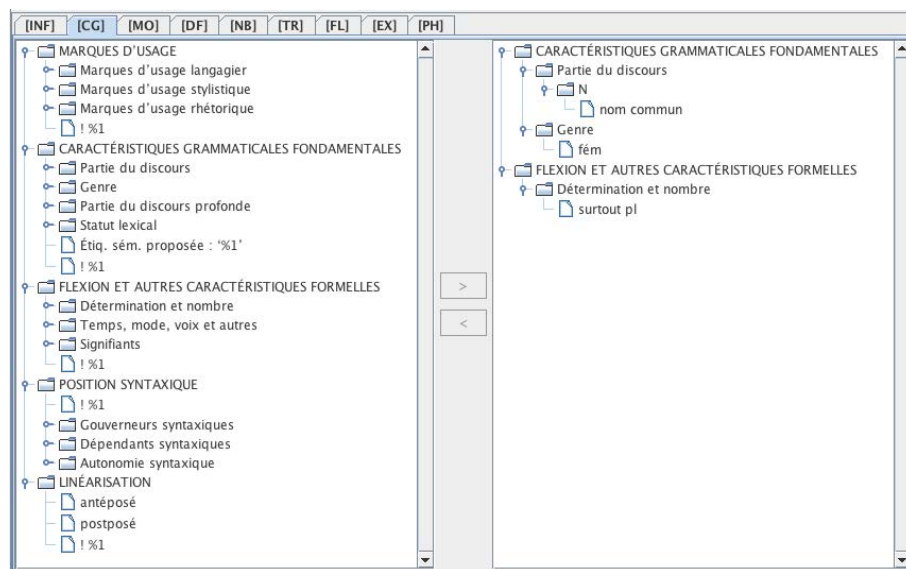
FIG. 2.9 : Caractéristiques grammaticales de ABEILLES l.b
