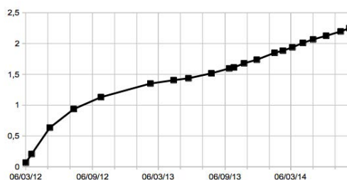
FIG. 2.26 : Évolution du degré sortant moyen
