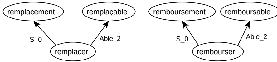
FIG. 4.16 : Exemples de CFC non analogues : méta-pdd ? liens =
