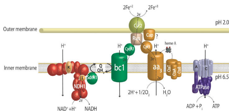
Figure 30 : Représentation de l'oxydation du Fe(II) par A. ferrooxidans ATCC 23270. La réduction de l' O_2 via le complexe aa3 ou la réduction du NAD^+ via un ensemble de quinone et un complexe NDH. La première voie consomme les protons entrant via le complexe ATPase qui entraîne la production d'ATP tandis que la seconde conduit à la production du NADH (Quatrini et al. 2009).
