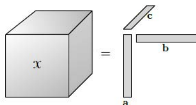
Figure 21 : Tenseur d'ordre 3 de rang 1, X = a \circ b \circ c . L'élément (i, j, k) de X est donné par x_{ijk} = a_i b_j c_k .
