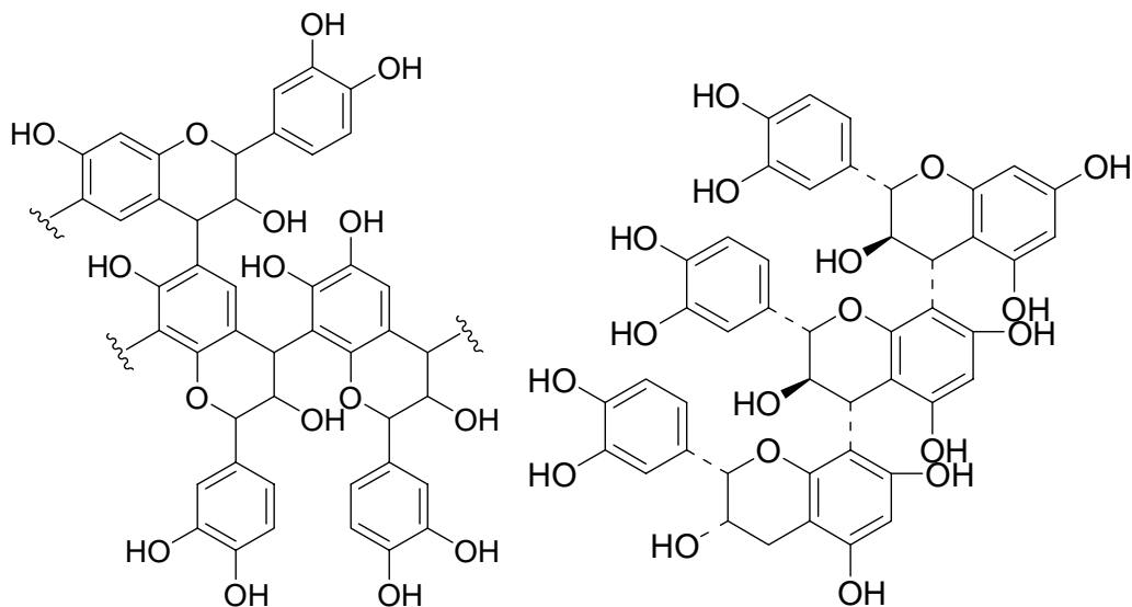
Figure 19 : Structure des tanins condensés
