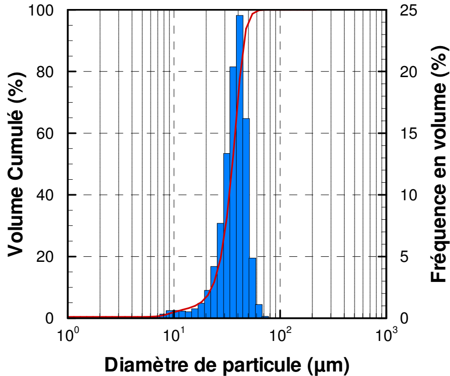
FIGURE 4.7 – Granulométrie fournie par le constructeur pour le brouillard d'eau
