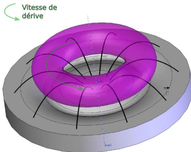
Figure I.2 Forme typique (tore) du plasma magnétron au-dessus de la cible, issu de [Imbert 2006].
