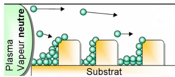
Figure I.4 Dépôt d'un film mince d'atomes neutres sur un substrat [Konstantinidis 2004].
