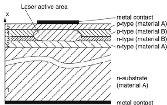
Figure II.9 Schéma d'une hétérojonction
