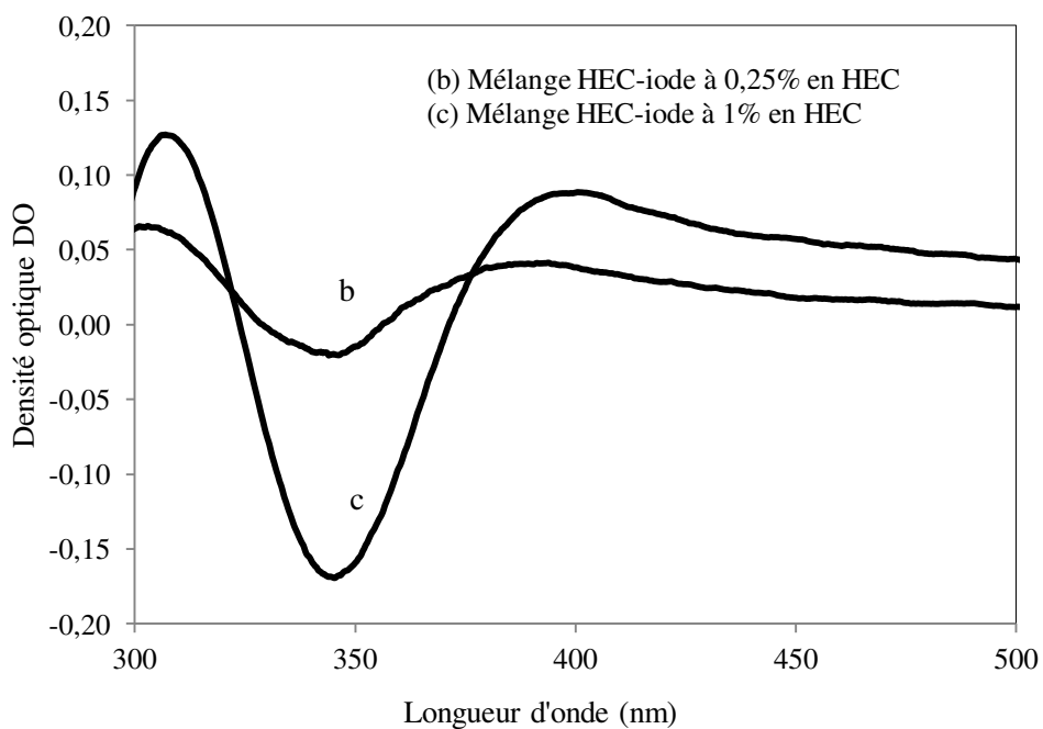
Figure V.9 : Spectre d'absorption de mélanges HEC-iodine en solution aqueuse basique (pH = 7,4-7,8) à 20° C avec une solution KI/I 2 dans l'eau comme référence et des concentrations en ion iodure et en iode égales à : [I^-]_0=1,16 \cdot 10^{-2} M et [I_2]_0=4,5 \cdot 10^{-5} M.
