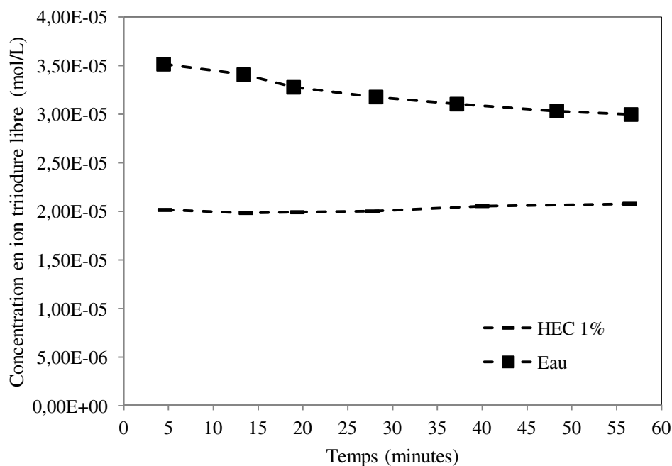
Figure V.18 : Evolution de la concentration en ion triiodure libre au cours du temps en milieu acide (pH = 2-3) à 25° C avec des concentrations en ion iodure et en iode initiales égales à : [I]_0=1,16.10^{-2} M et [I_2]_0= 4,5.10^{-5} M.
