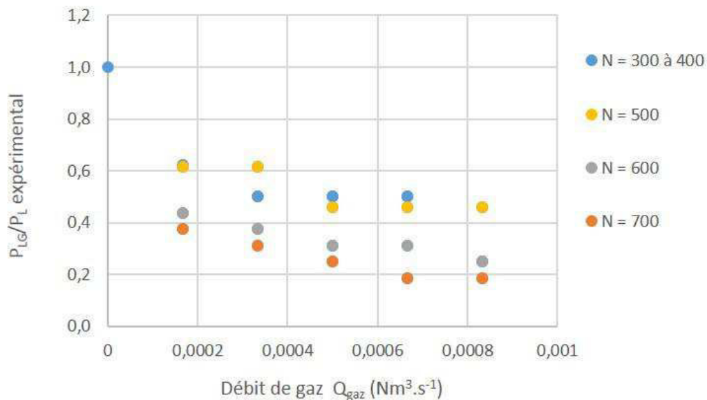
Figure 4.1 – Rapport P_{LG}/P_L en fonction du débit de gaz et de la vitesse d'agitation ( N en min^{-1} )
