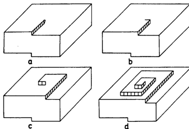
Figure 1.8 – Mécanisme de croissance en spirale - Théorie BCF
