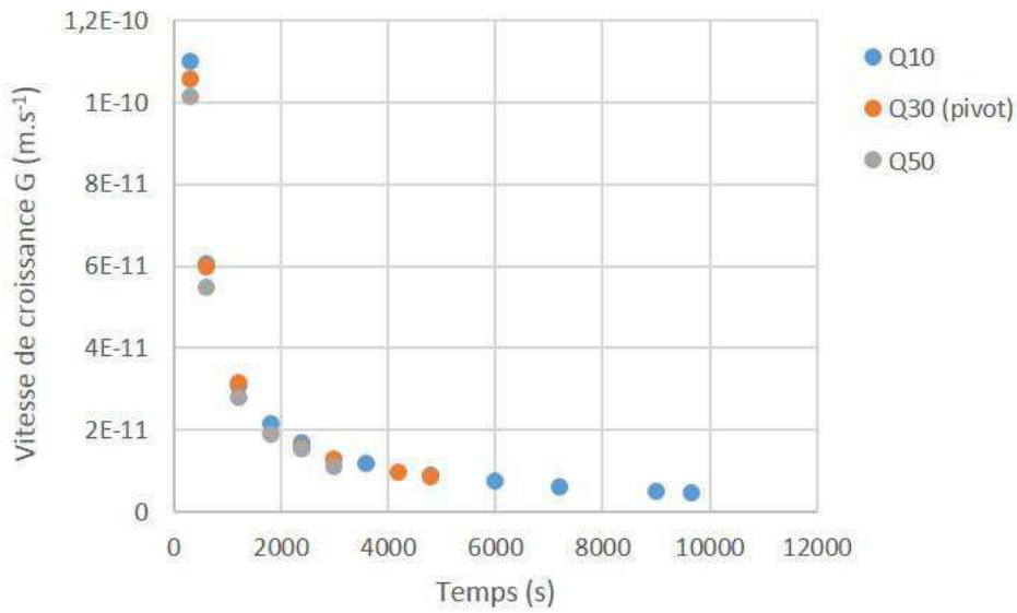
Figure 5.9 – Vitesse de croissance cristalline G en fonction du temps et du débit de gaz ( T = 18\text{ }^{\circ}\text{C} et N = 500\text{ min}^{-1} )
