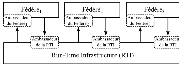
FIGURE 4.1 – Exemple de fédération HLA
