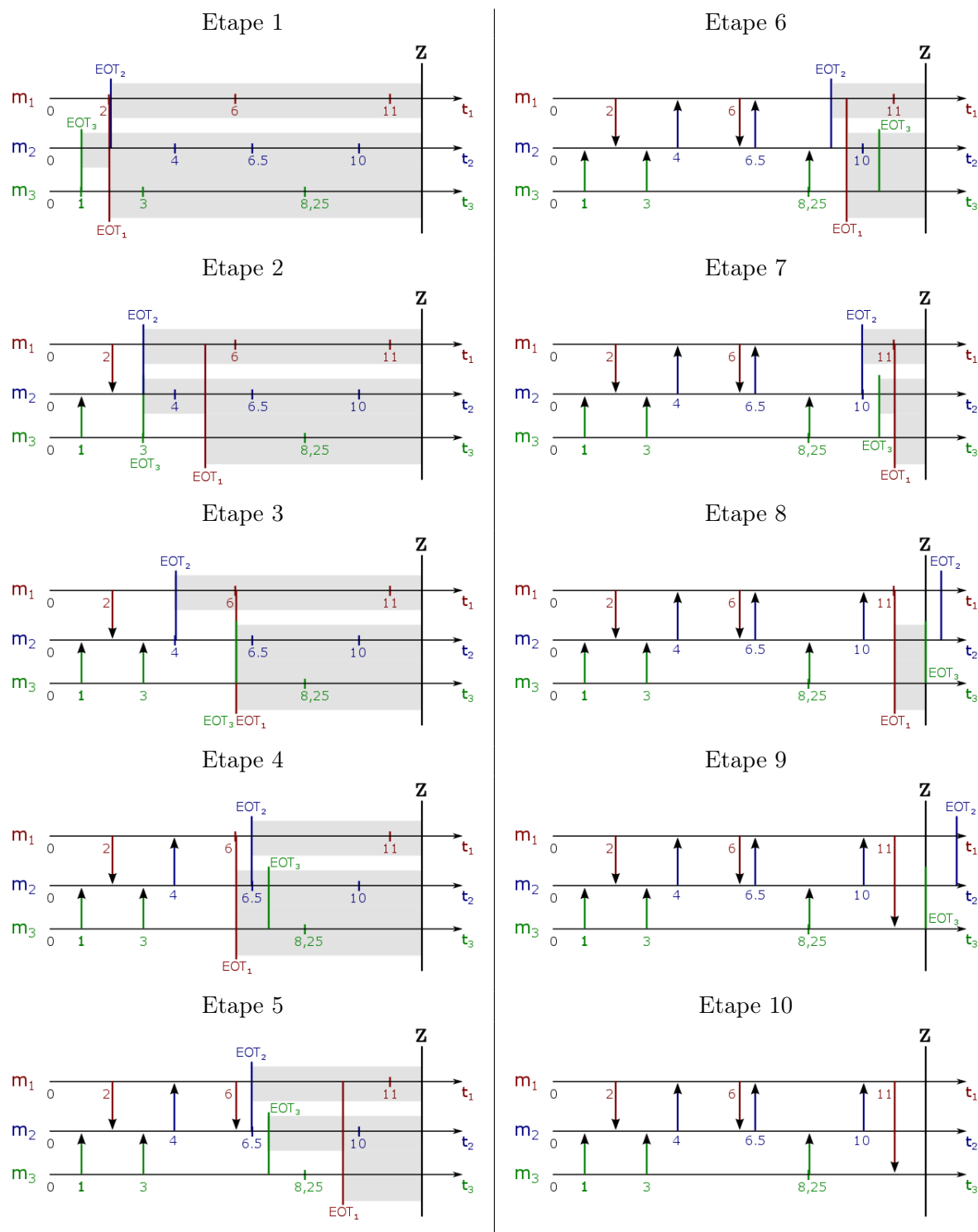
FIGURE 6.5 – Exemple de déroulement de la simulation parallèle du multi-modèle de la Figure 6.1a. Les événements internes planifiés sont disposés sur les axes horizontaux représentant le temps simulé. Chaque flèche verticale indique l'envoi d'un événement externe. Les événements en dehors des zones grises correspondent aux événements sécurisés.
