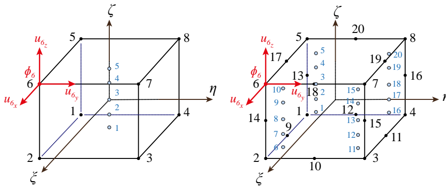
Figure 3.1 Géométrie de référence des éléments finis SHB8PSE et SHB20E et positionnement des points d'intégration ( n_{int}=5 )
