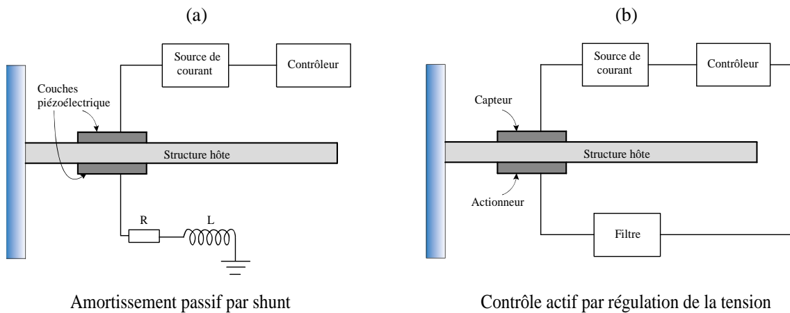
Figure 2 Systèmes d'amortissement passif (a) et actif (b) des vibrations au moyen des matériaux piézoélectriques
