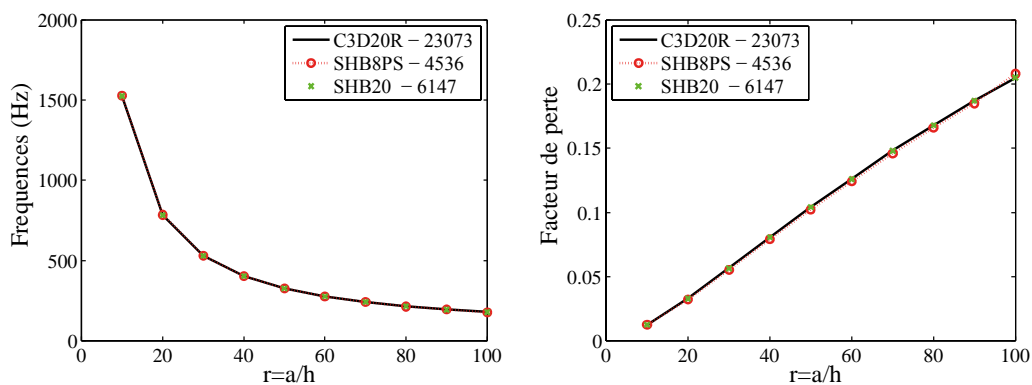
Figure 2.11 Paramètres amortissants : rapport d'épaisseurs r = h_c/h_f fixe, épaisseur totale h \in [0, a/10]
