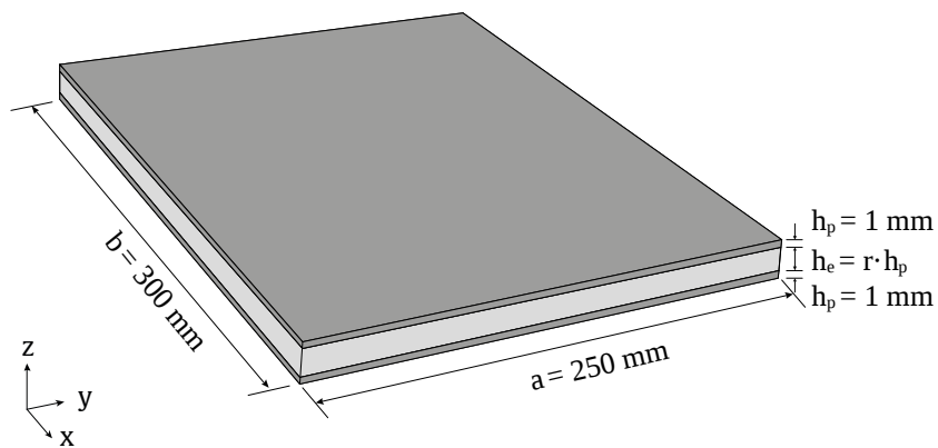
Figure 3.11 Plaque sandwich rectangulaire sur appuis simples
